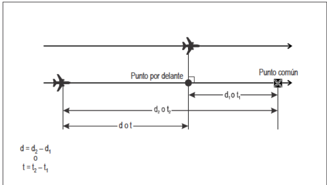
Figura 7-31. Cálculo de la distancia/tiempo longitudinal entre aeronaves — derroteros paralelos [véase 7.4.3.12.5 c)]
