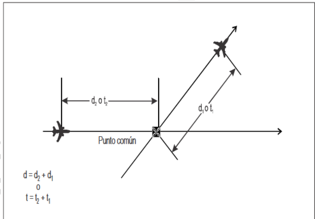
Figura 7-30. Cálculo de la distancia/tiempo longitudinal entre aeronaves — lados opuestos del punto común [véase 7.4.3.12.5 b)]
