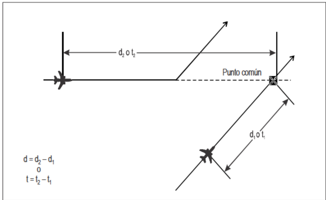
Figura 7-29. Cálculo de la distancia/tiempo longitudinal entre aeronaves — misma derrota prevista, pero no idéntica [véase 7.4.3.12.5 b)]
