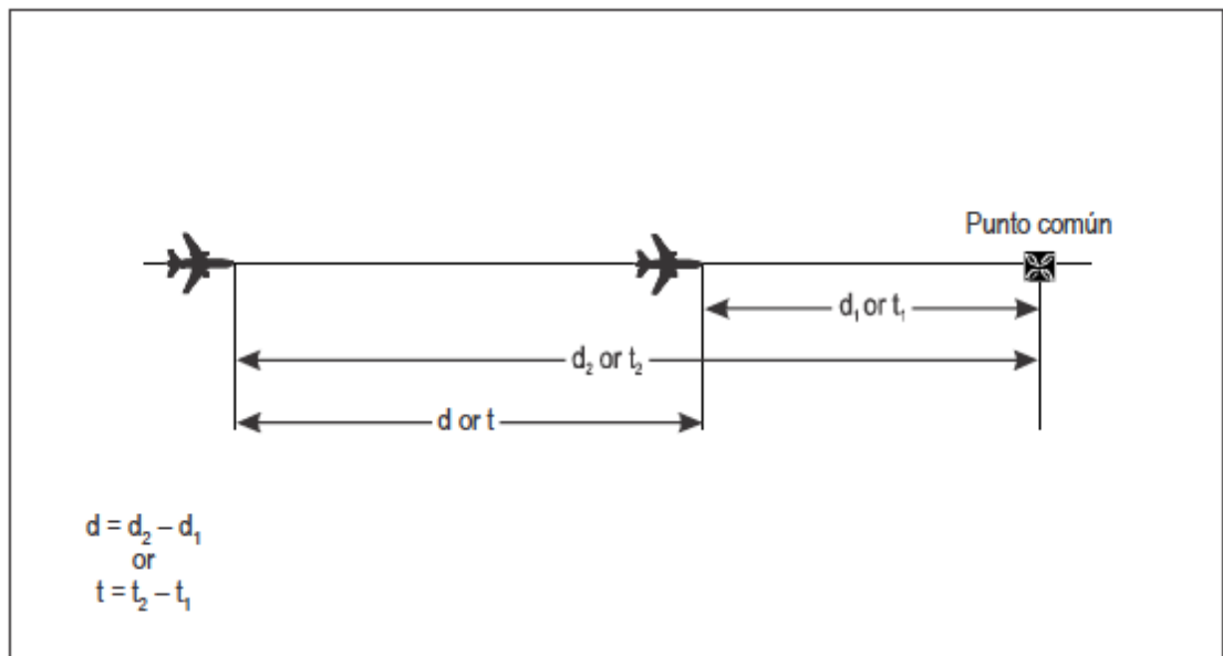
Figura 7-26. Cálculo de la distancia/tiempo longitudinal entre aeronaves — derrota idéntica, mismo sentido [véase 7.4.3.12.5 a)]
