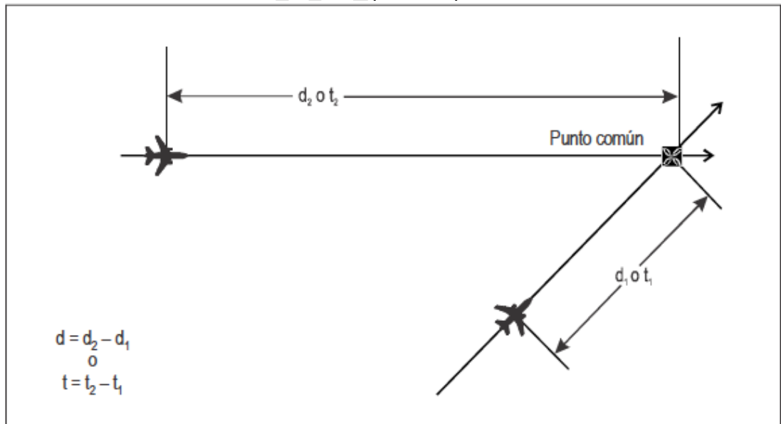
Figura 7-28. Cálculo de la distancia/tiempo longitudinal entre aeronaves — misma derrota, pero no idéntica y derrota que se cruzan [véase 7.4.3.12.5 b)]
