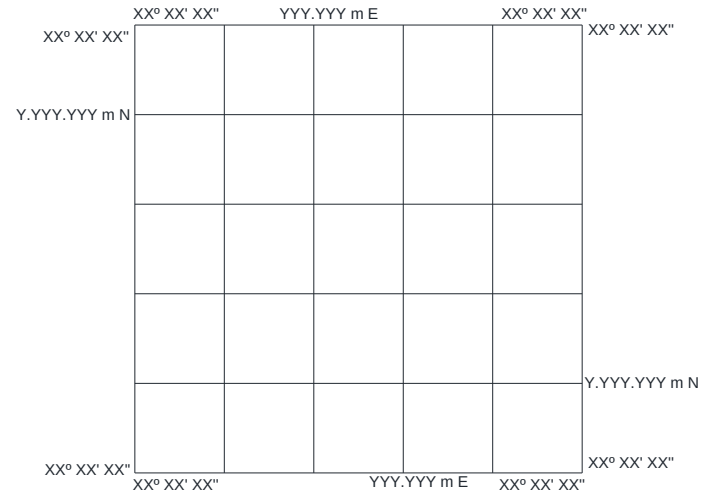
Figura 6-4. Cuadrícula UTM
