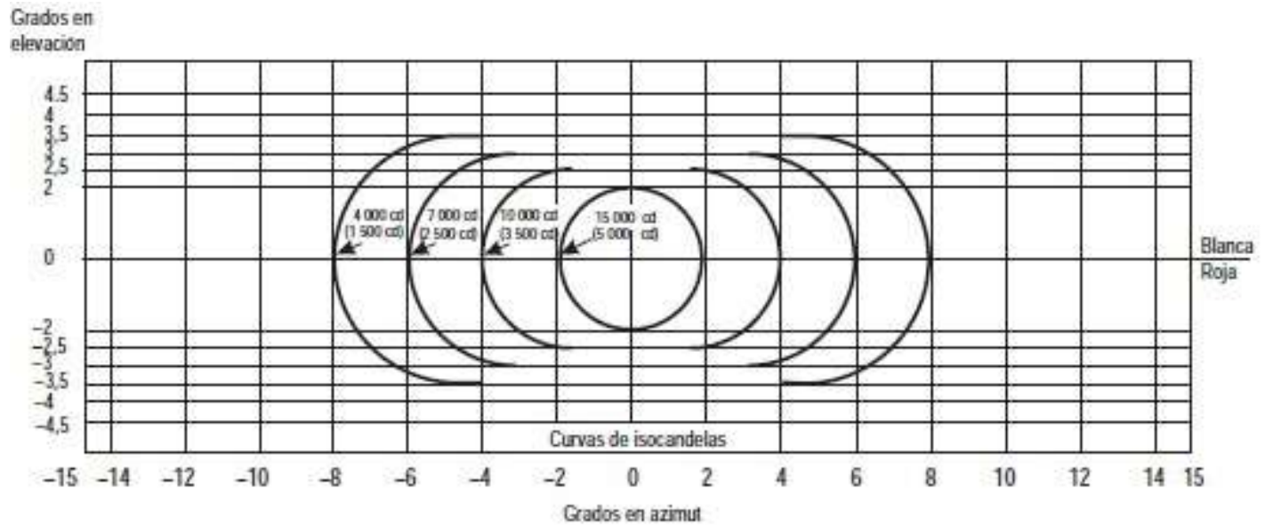
Figura ADJB-23. Distribución de la intensidad luminosa del PAPI y del APAPI
