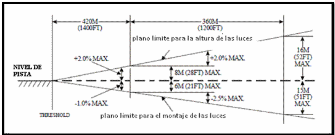
Figura ADJJ-3. Plano límite de instalación de las luces
