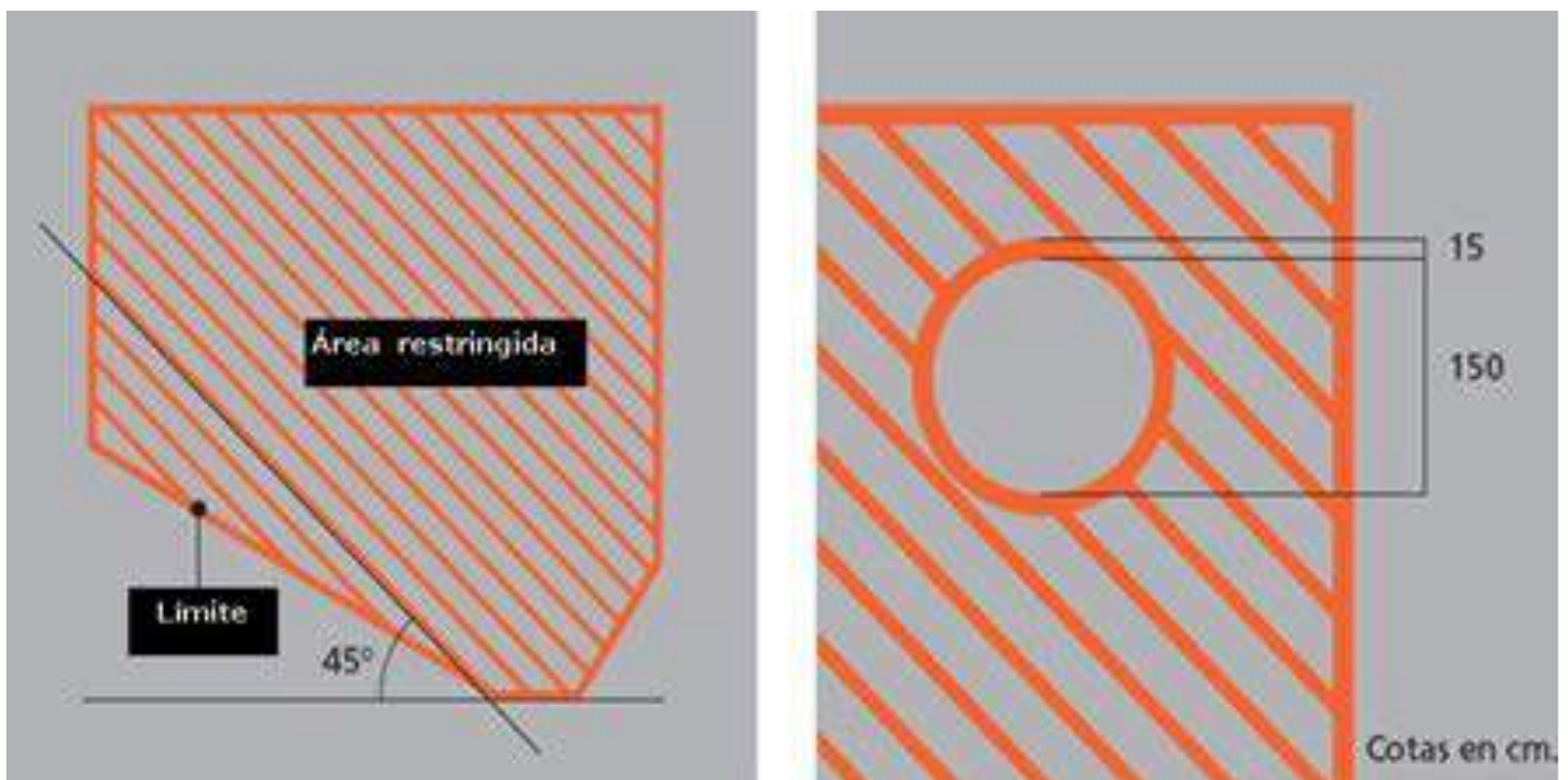
Figura 2-9-2. Señal de área de prohibición de estacionamiento NPL y en su interior la NPA zona de prohibición de estacionamiento y parada de equipos. El círculo representa la posición de reposo de la cabeza de la pasarela
