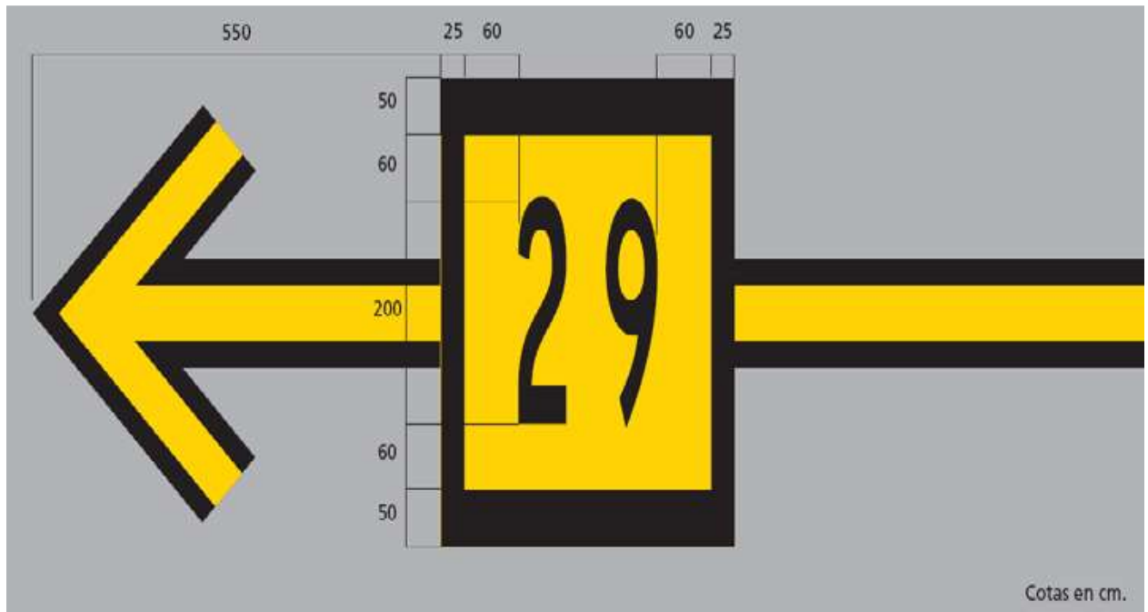
Figura 2-12-1. Puestos de estacionamiento con una dirección única de rodaje hacia el puesto
