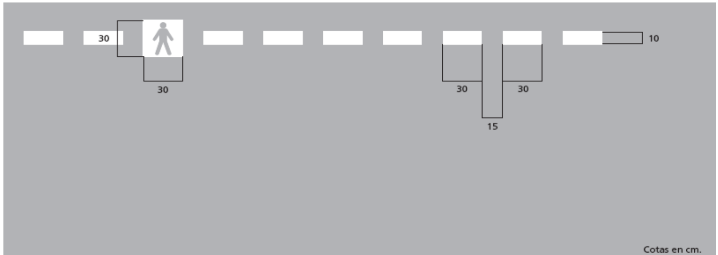
Figura 2-27-1. Señal de senda peatonal en Plataforma
