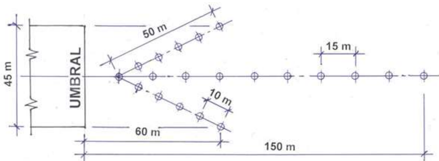
Figura 1-4-3. Sencillo de Iluminación de Aproximación Reducido Configuración 2
