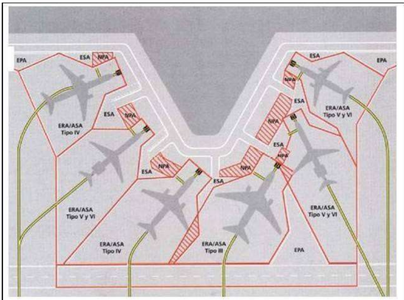
Figura 2-26-3. Ejemplo de Solución de solape para diferentes tipos de aeronave
