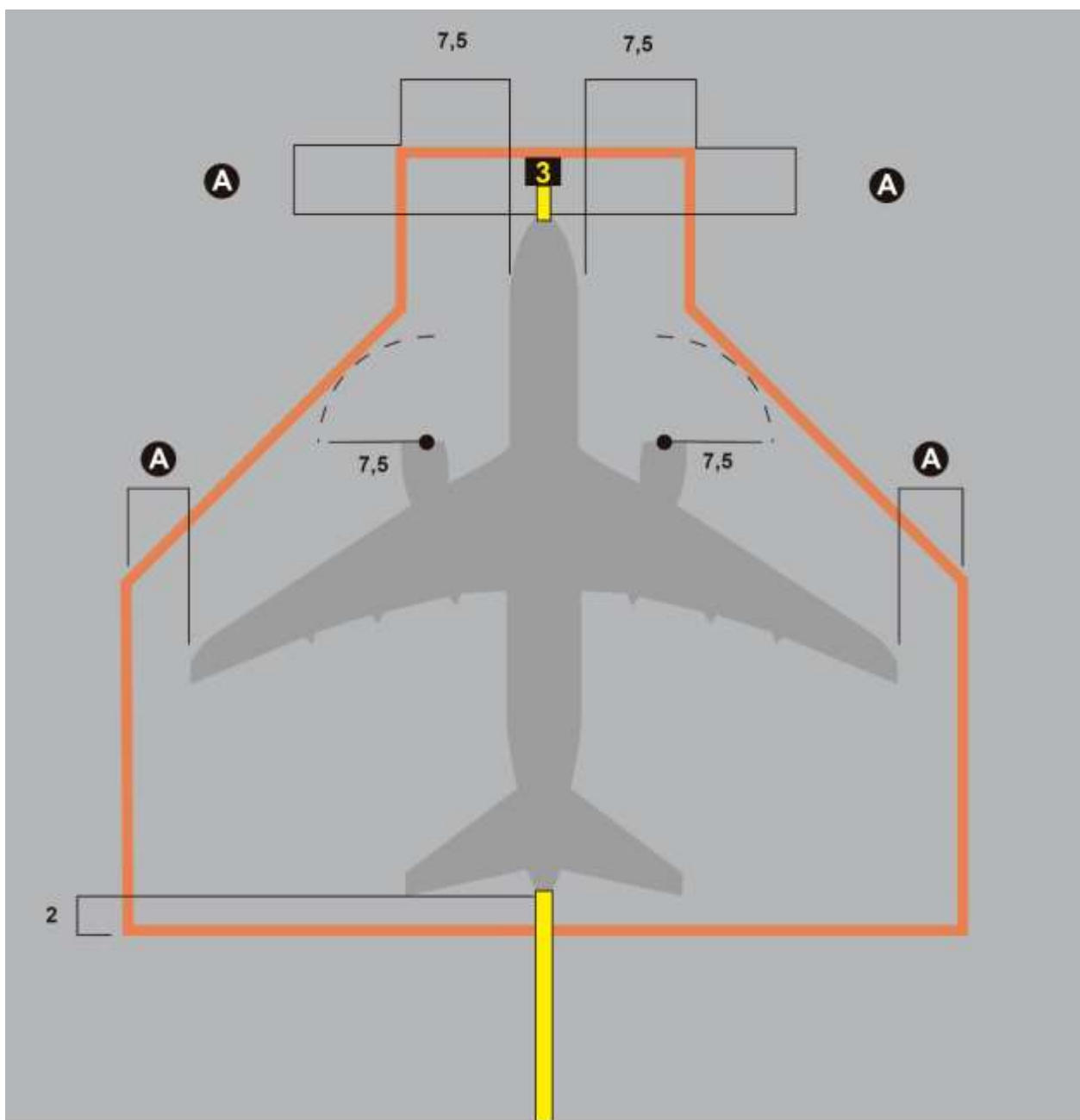
Figura 2-24-1. Márgenes mínimos de seguridad
