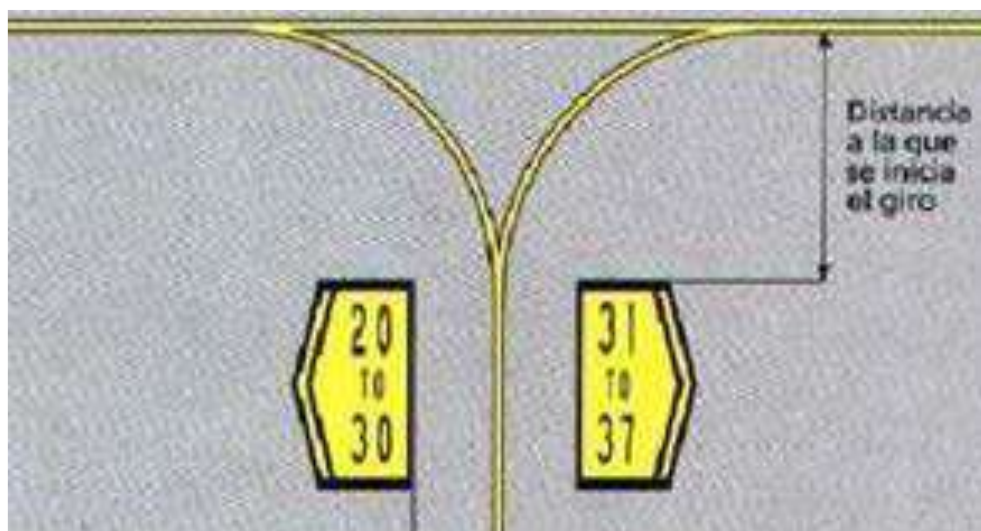
Figura 2-10-2. Ejemplo aplicación de la Señal direccional a puestos de estacionamiento de aeronaves
