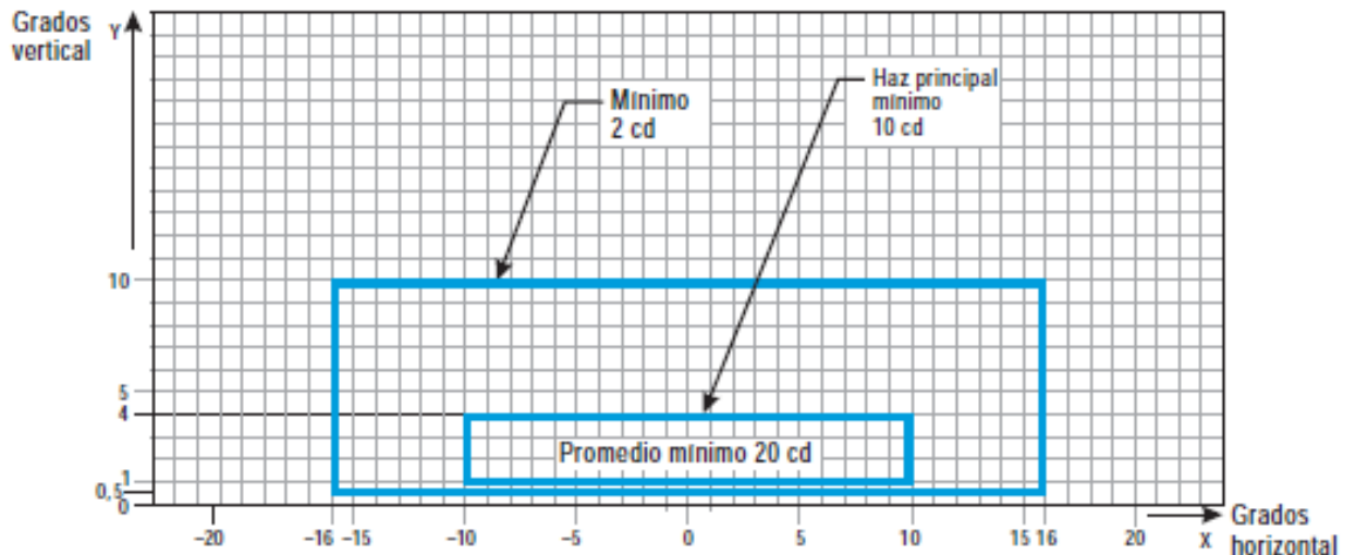
Figura ADJB-15. Diagrama de isocandelas para luces de eje de calle de rodaje (espaciado de 30 metros, 60 metros), de barra de prohibición de acceso y de barra de parada en tramos rectos previstas para ser utilizadas en condiciones de alcance visual en la pista de 350 metros o superior
