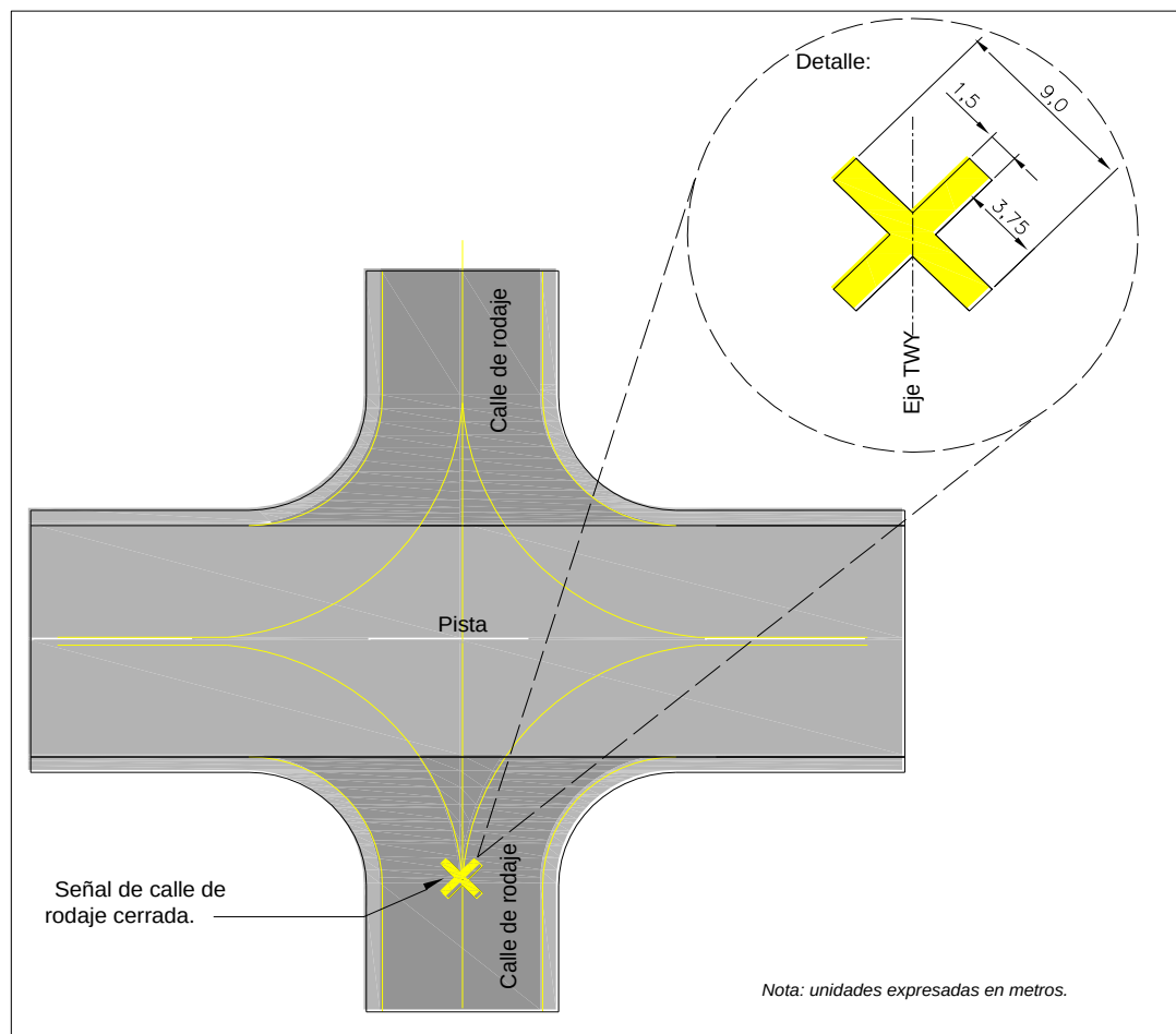
Figura 5-1-2 Señales de calle de rodaje cerradas – emplazamiento respecto a una pista en uso
