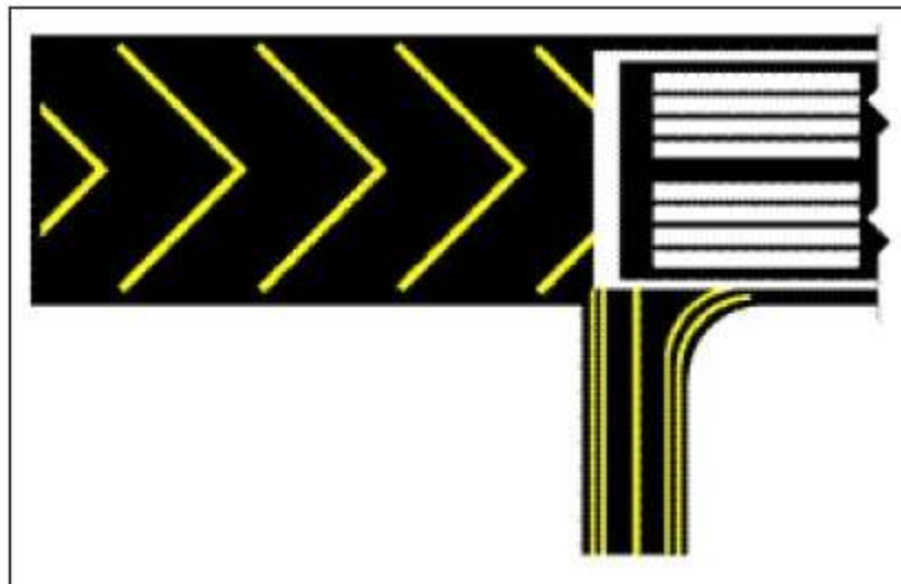
Figura 5-3-2. Configuración de la Señal anterior al umbral
