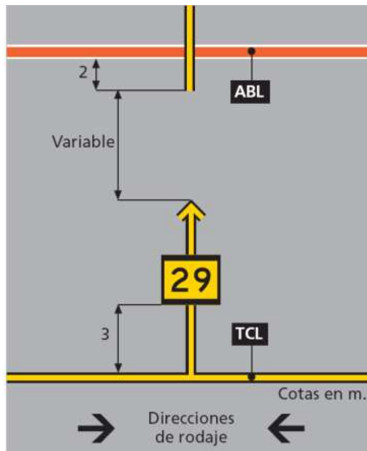
Figura 2-12-3. Identificación de puesto de estacionamiento en la señal de entrada
