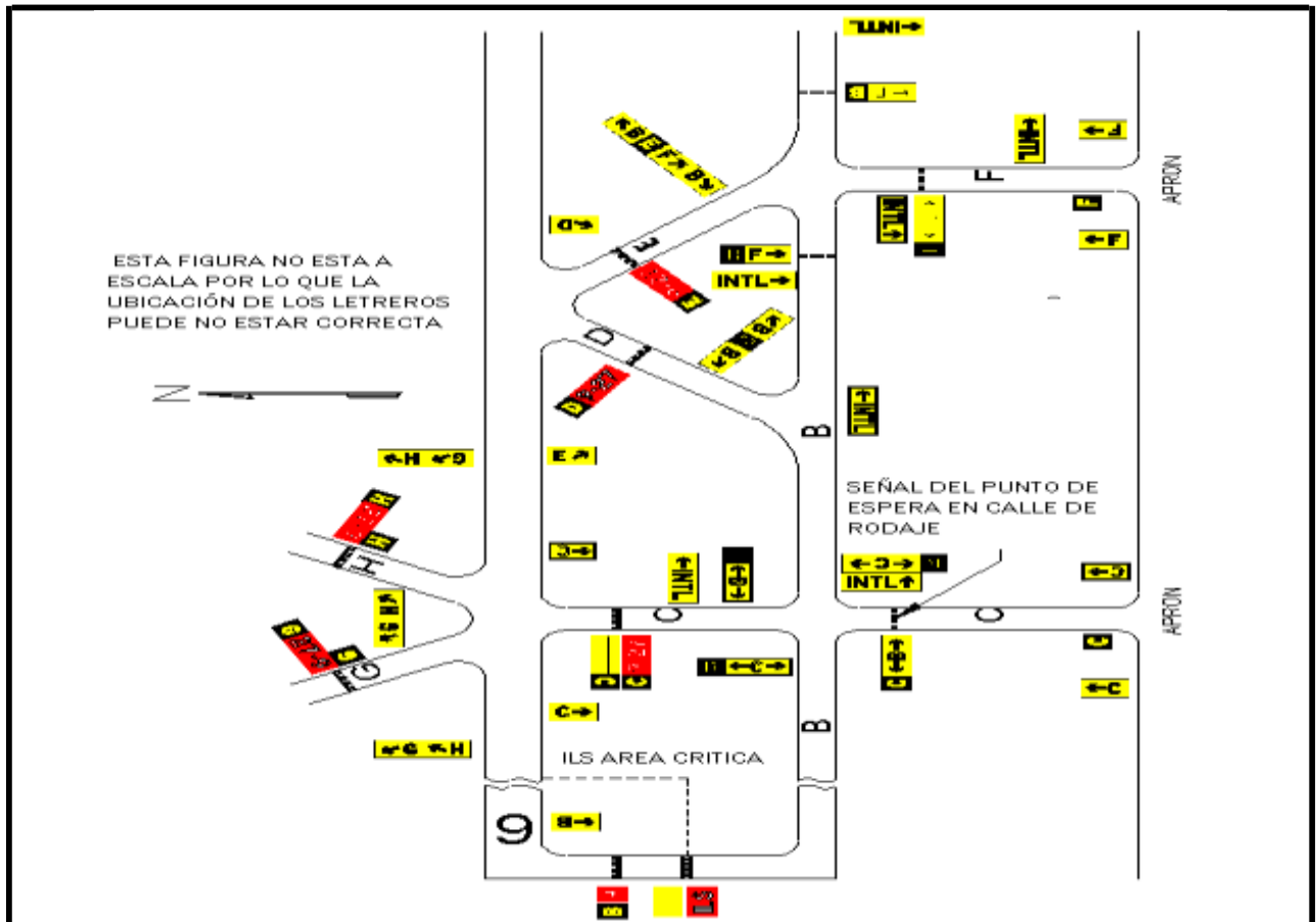
Figura 2-3-3. Caso C - Configuración Letreros
