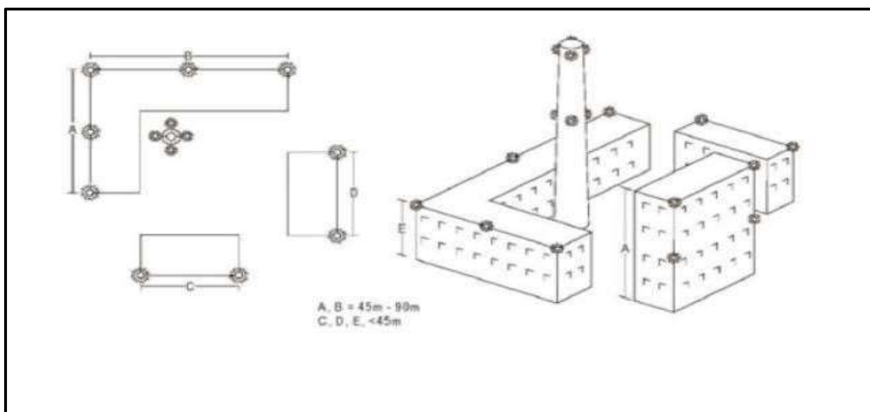
Figura 2-3-7. Ejemplos de iluminación de edificios
