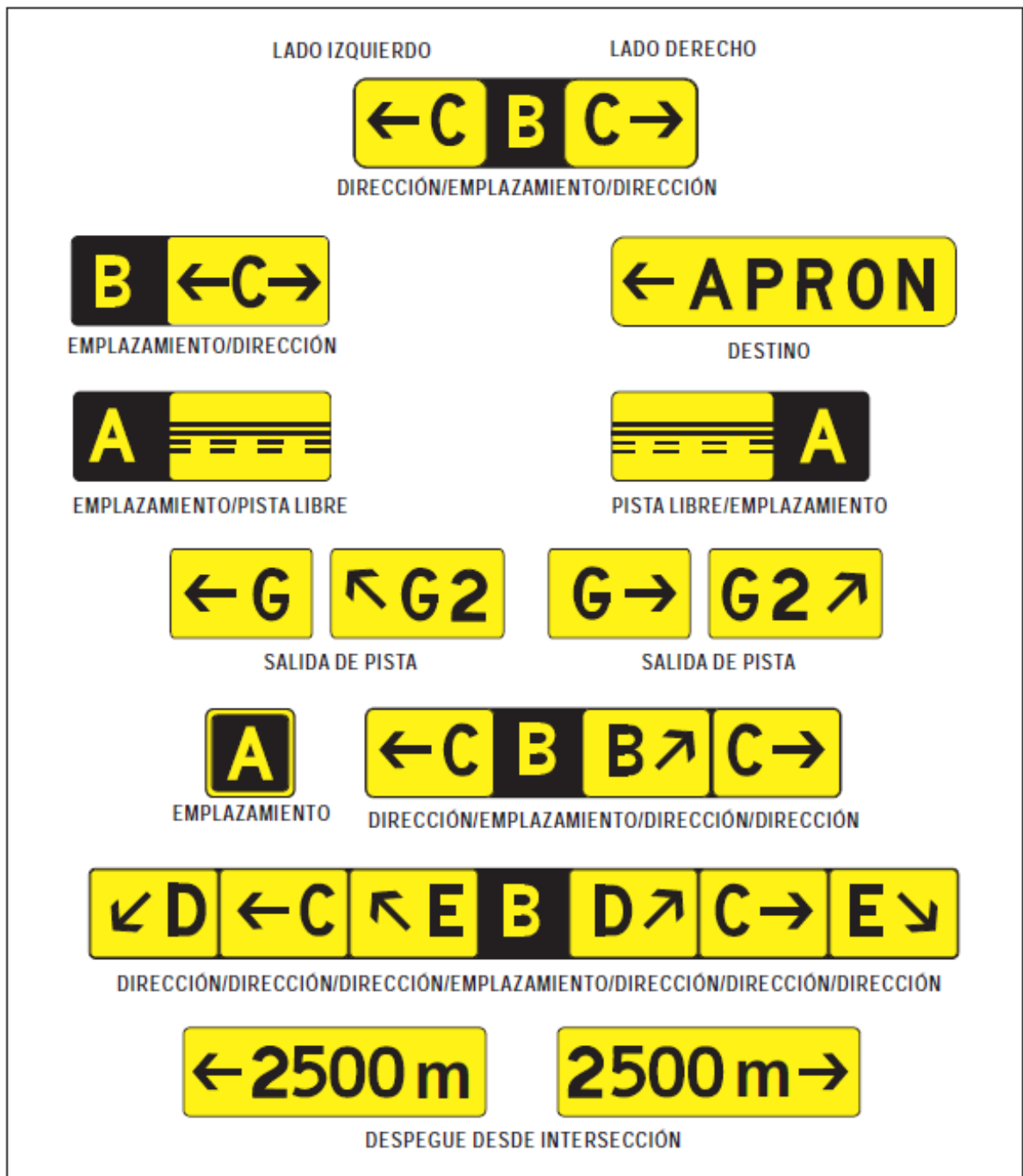
Figura 2-2-2. Letreros de información
