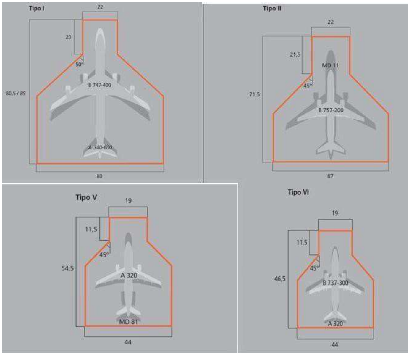
Figura 2-25-2. Tipos básicos de puestos de estacionamiento agrupados en ocho tipos de aeronaves
