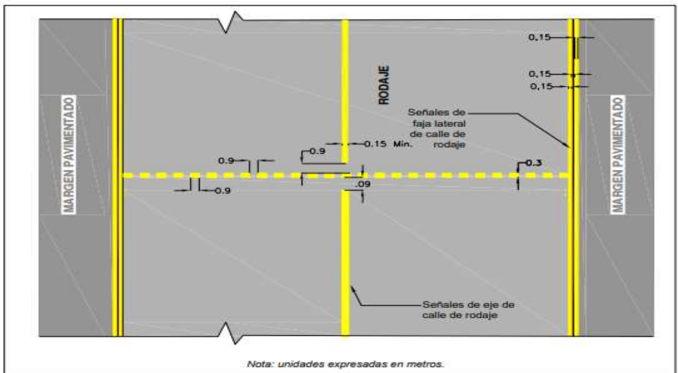
Figura 3-6-2. Señal de punto de espera intermedio.
