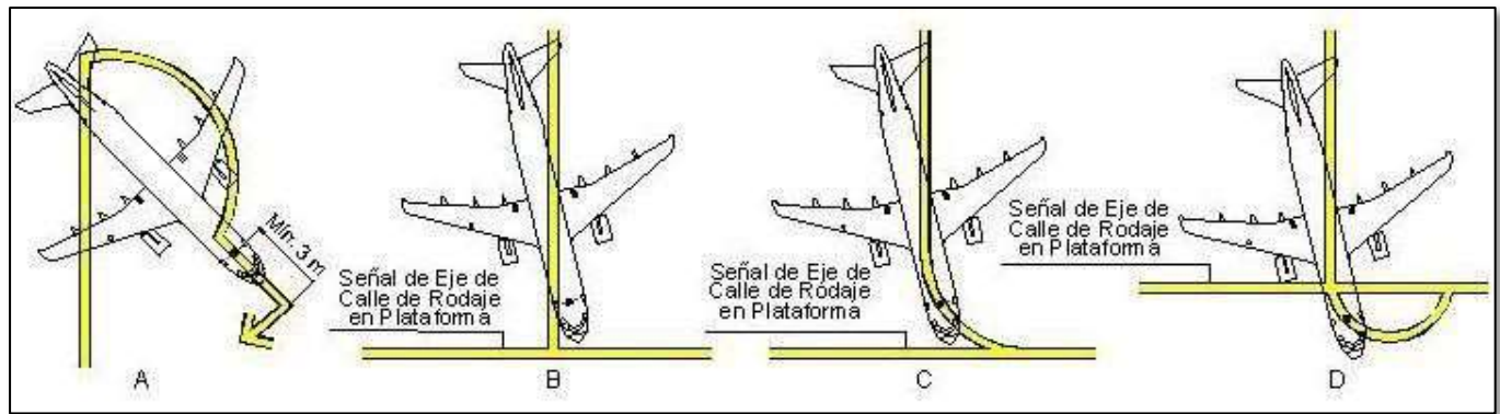
Figura 2-14-2. Señal de salida de puesto de estacionamiento, con giro, recta, simple y desplazada
