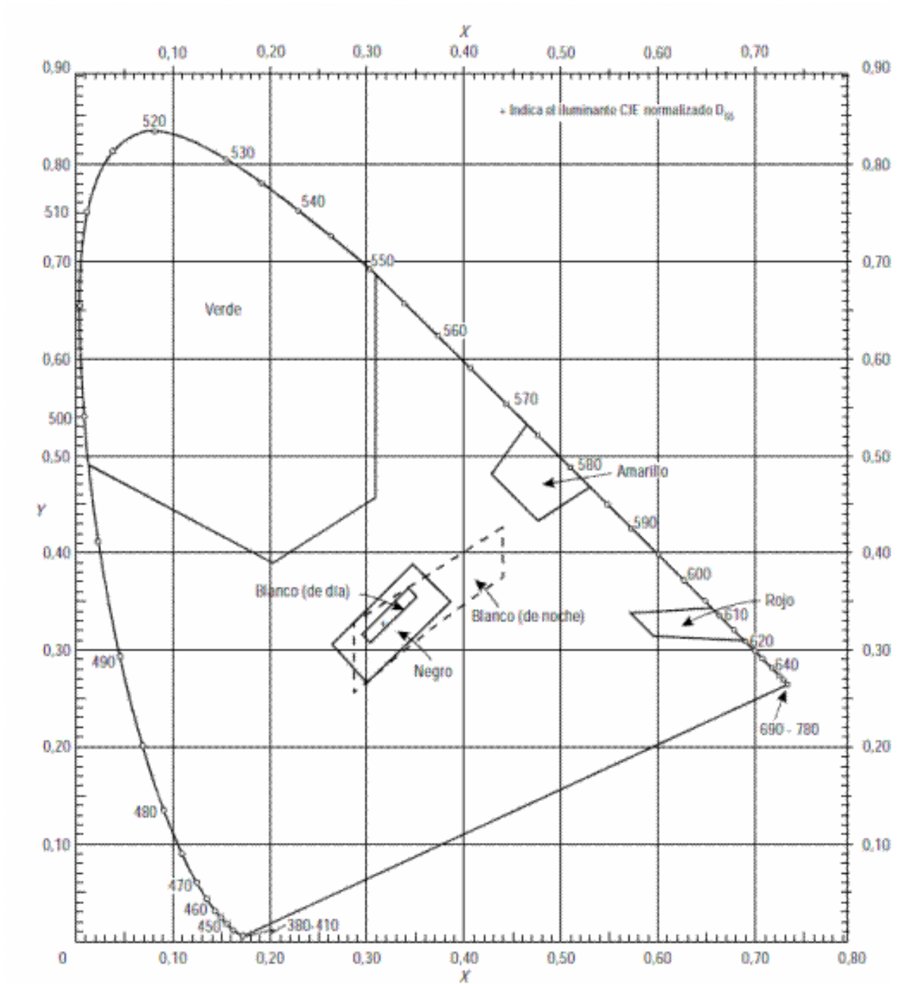
Figura ADJA-3-3. Colores de los letreros y paneles transiluminados (iluminación interna) o luminiscentes
