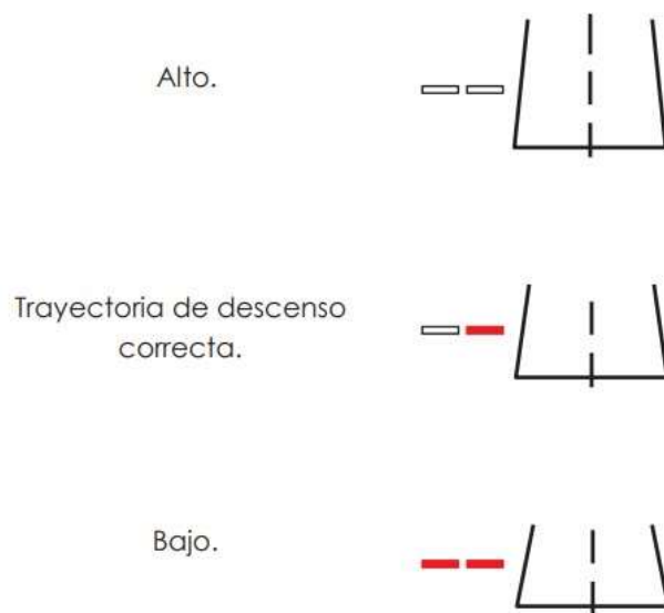
Figura 1-9-2. Visualización correspondiente PAPI y APAPI
