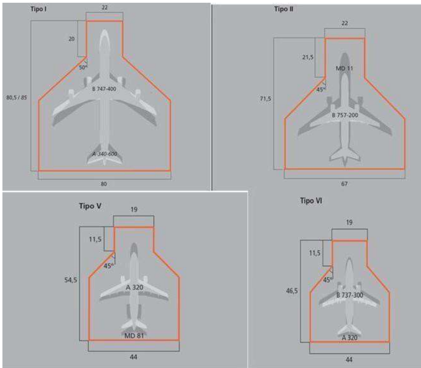
Figura 2-25-3. Agrupación de las aeronaves en 8 tipos para los puestos de estacionamiento
