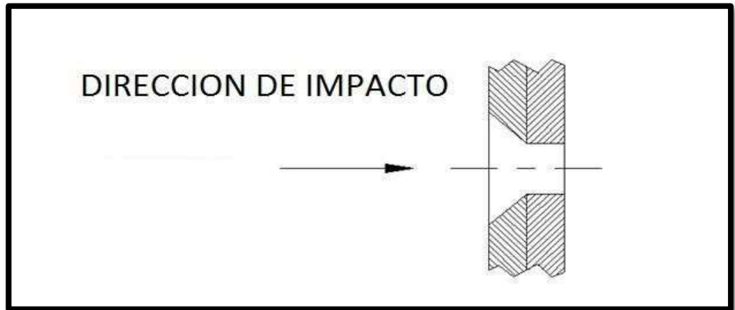
Figura ADJB-7. Ejemplos de sujetadores Frangibles
