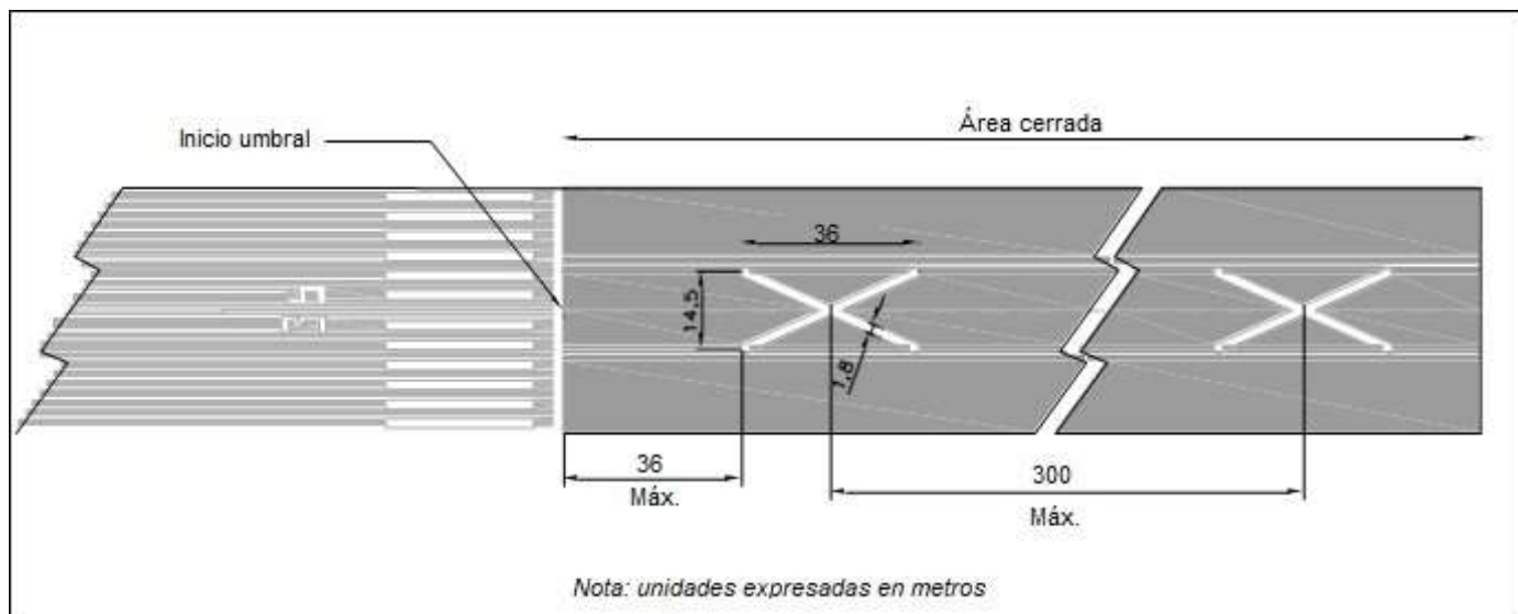
Figura 1-9-1. Señal de zona cerrada en pista
