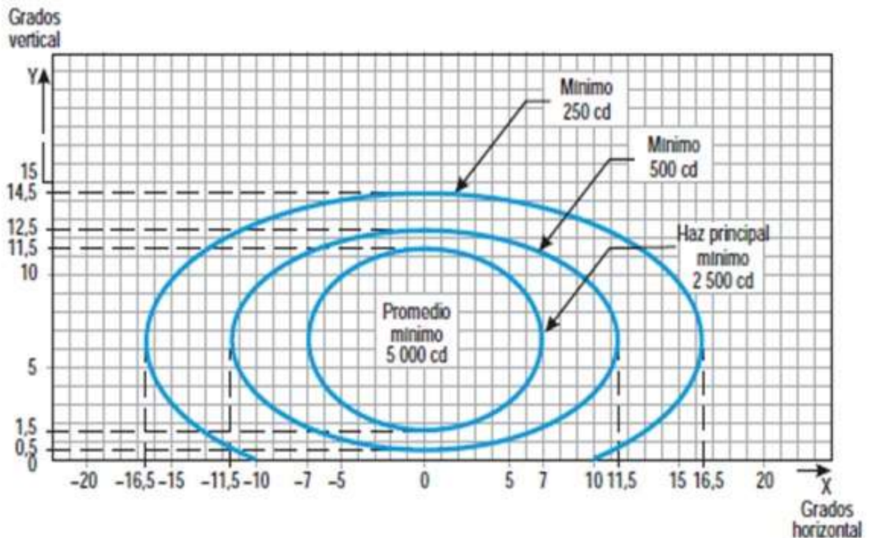
Figura ADJB-2. Diagrama de isocandelas para las luces de la fila lateral de aproximación (luz roja)
