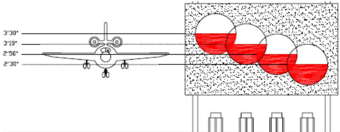
Figura 1-10-1. Reglaje de los ángulos del PAPI no equipada con ILS
