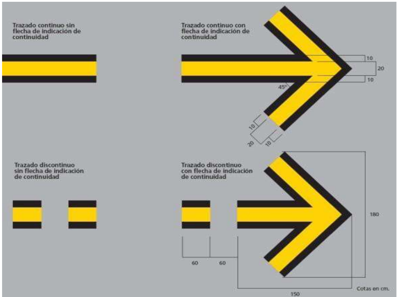
Figura 2-14-1. Señal de salida de puesto de estacionamiento
