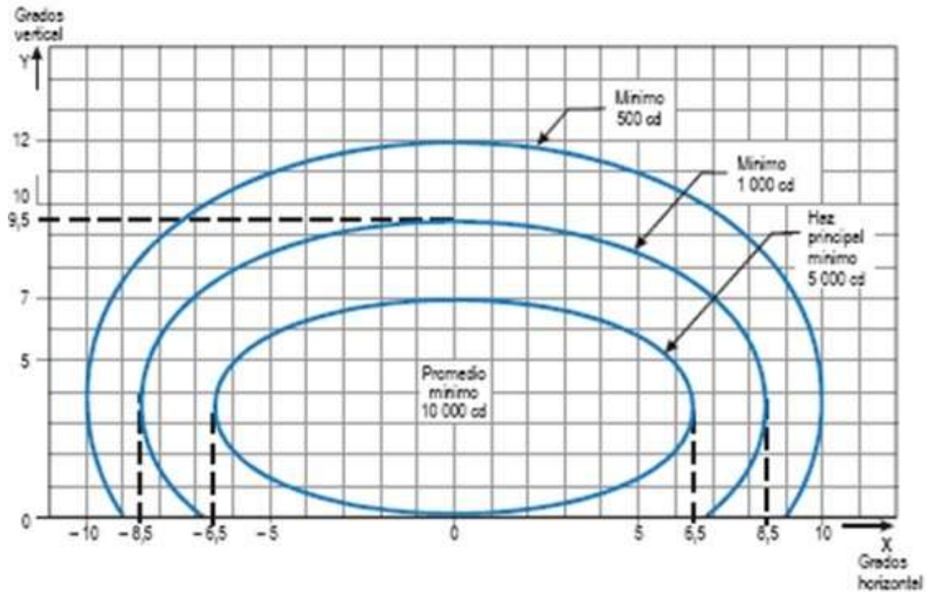
Figura ADJB-10. Diagrama de isocandelas para las luces de borde de pista cuando el ancho de la pista es de (luz blanca)
