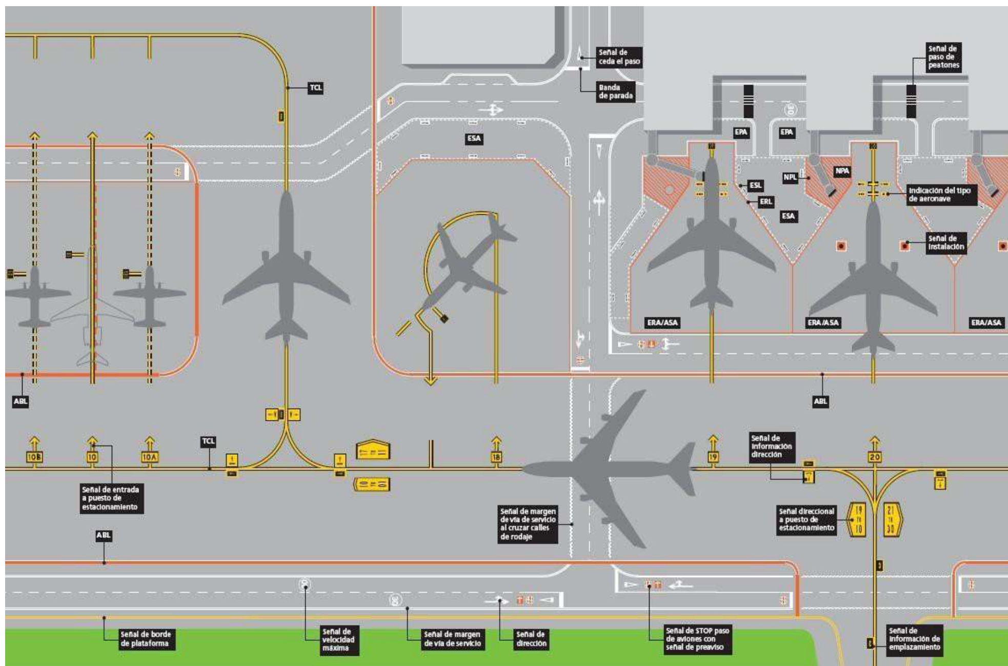
Figura 2-18-2. Vista General de señales
