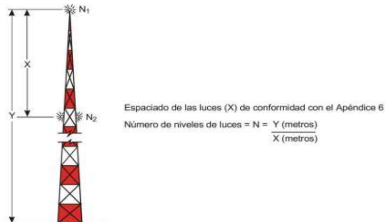
Figura 2-3-2. Ejemplos de señalamiento e iluminación de obstáculos en el caso de estructuras elevadas
