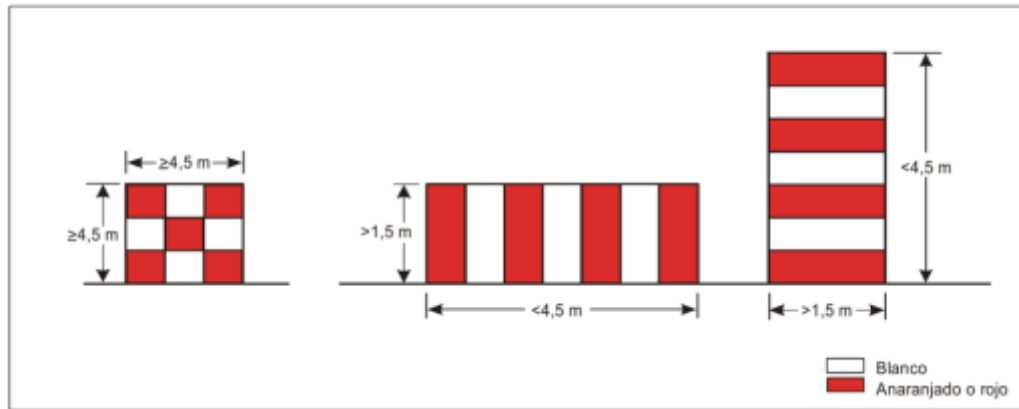
Figura 2-3-1. Configuraciones básicas de la señalización de obstáculos
