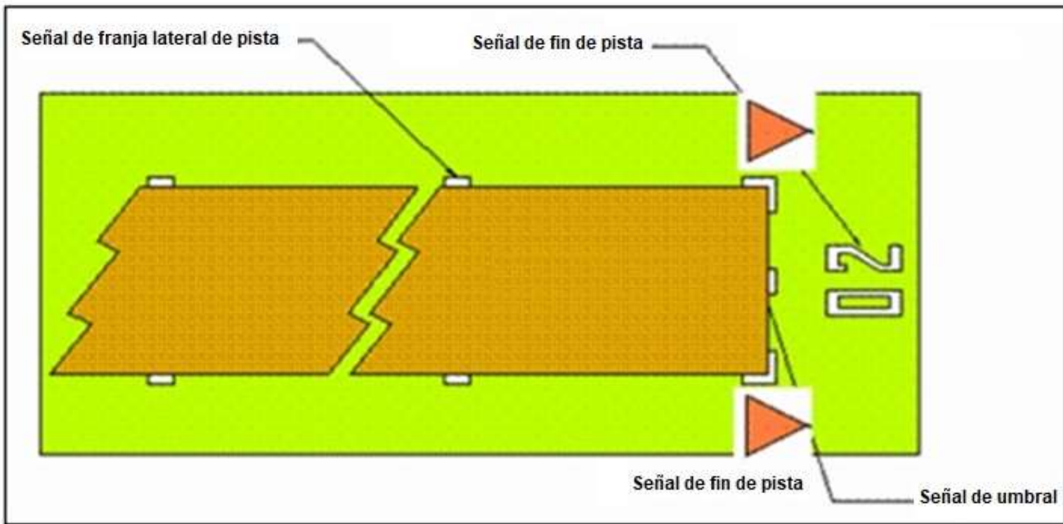
Figura 6-9-2. Emplazamiento de las Señales de fin de pistas no pavimentadas Tipo A
