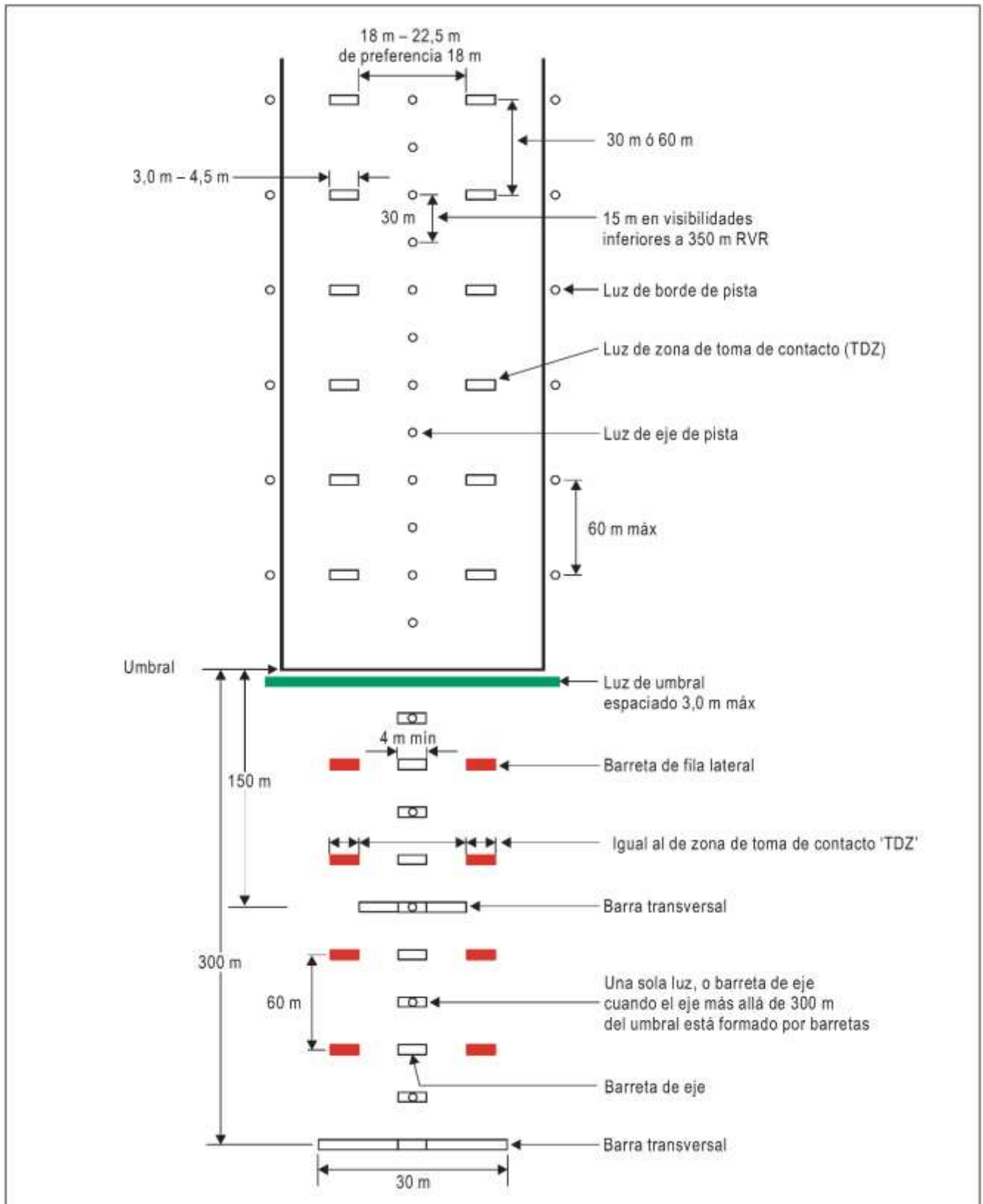
Figura 1-7-2. Iluminación de pista y de los 300 metros internos de la aproximación, en las pistas para aproximaciones de precisión de Categorías II y III
