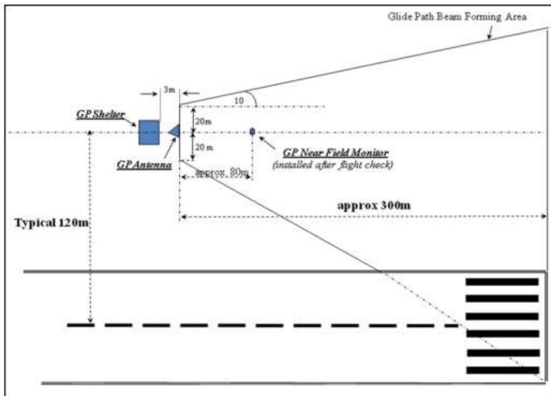
Figura 4-2-2. Instalación de la Senda de Planeo del ILS
