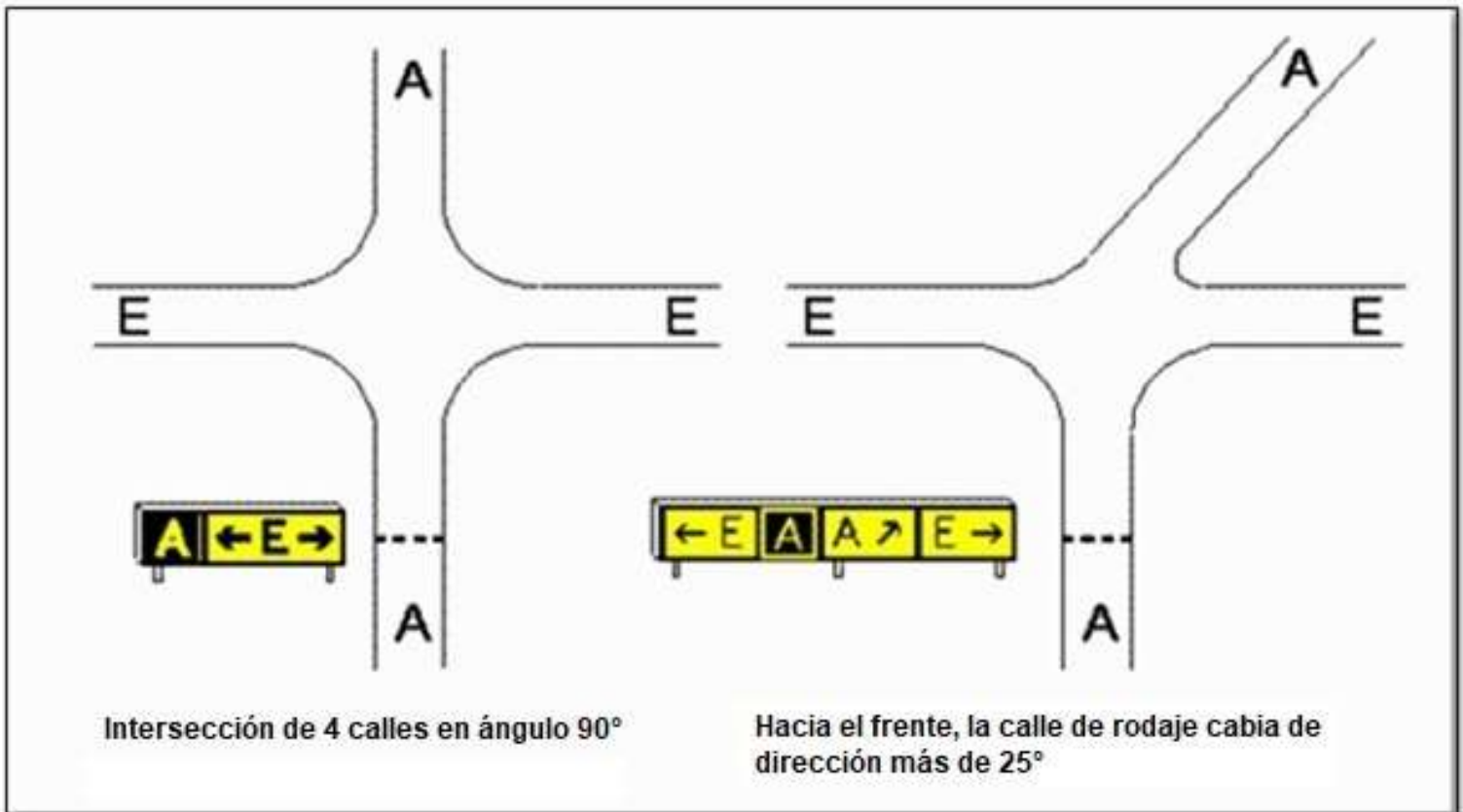
Figura 8-3-2. Caso B - Letreros de información
