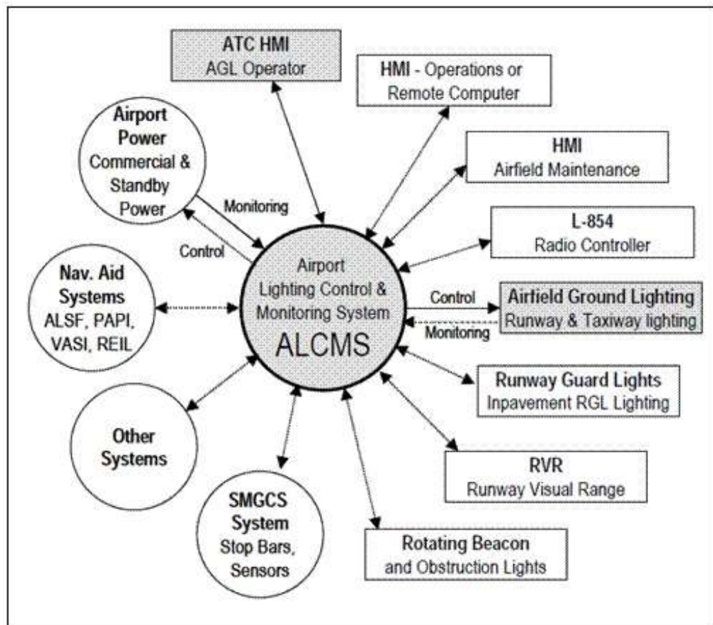
Figura ADJL-1: ALCMS Descripción de las interfaces
