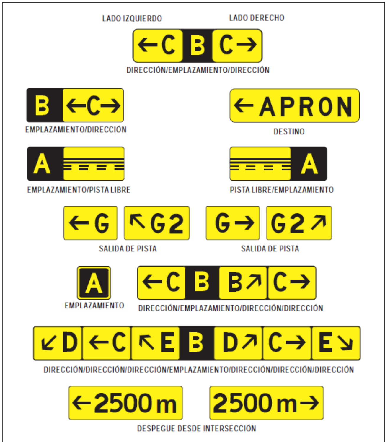
Figura 8-2-2. Letreros de información
