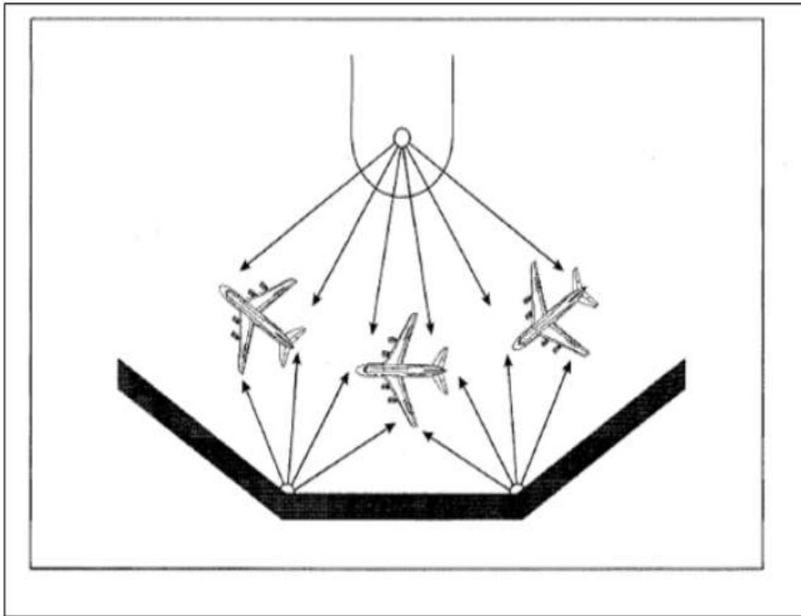
Figura ADJM-6. Disposición y enfoque característicos de las luces de proyectores para estacionamiento en paralelo
