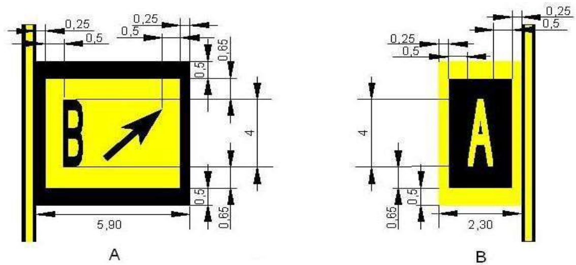
Figura 4-3-1 – Configuración y dimensiones de las señales de información (dirección / emplazamiento) en las calles de rodaje
