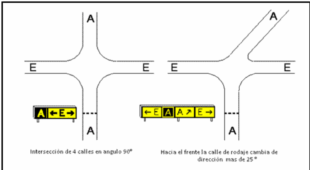
Figura 2-3-2. Caso B - Letreros de información
