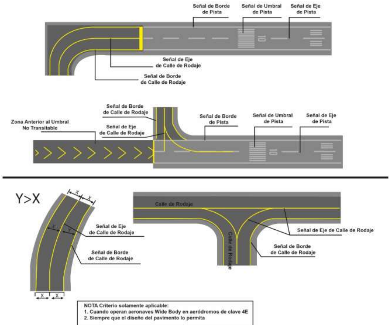
Figura 3-3-4. Ejemplos de Señales de faja lateral y eje de rodajes
