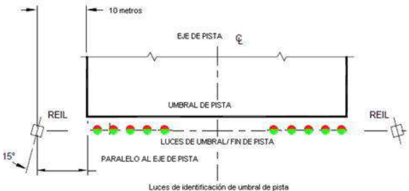
Figura 1-13-1. Luces de Identificación de umbral de pista
