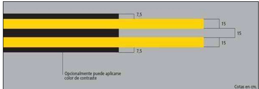
Figura 2-3-1. Señal de borde de plataforma
