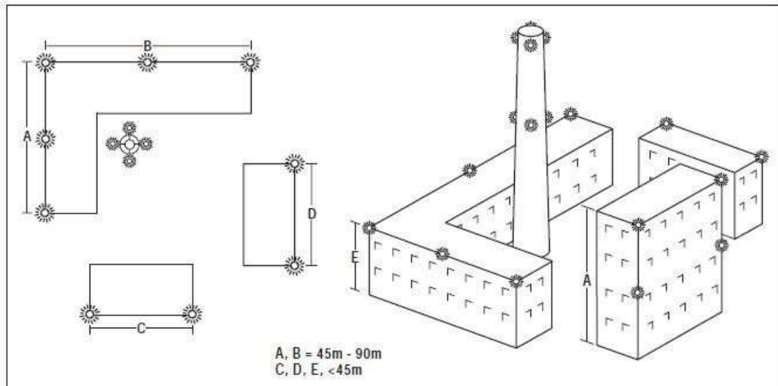
Figura ADJBA 9 Ejemplo de Sistema de Luces de Obstáculo para un Objeto Extenso
