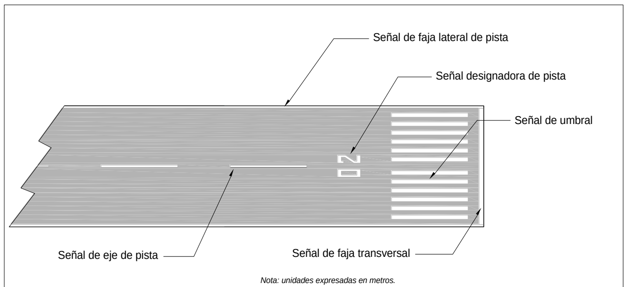
Figura 1-2-1. Señales de Pista
