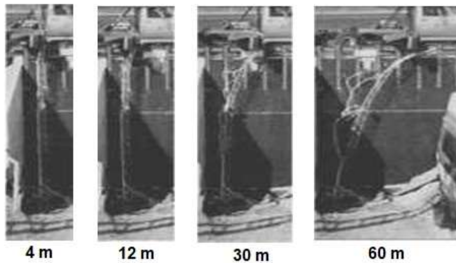
Figura ADJA-2. Eventos de impactos de simulación mediante análisis de elementos finitos (FEA) y de ensayo con modelos de tamaño natural velocidad de impacto 140 km/h; impacto lateral; aparato impactante rígido. Simulación FEA
