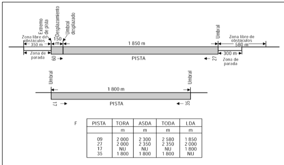
Figura 1-6-2. Determinación de las Distancias Declaradas.
