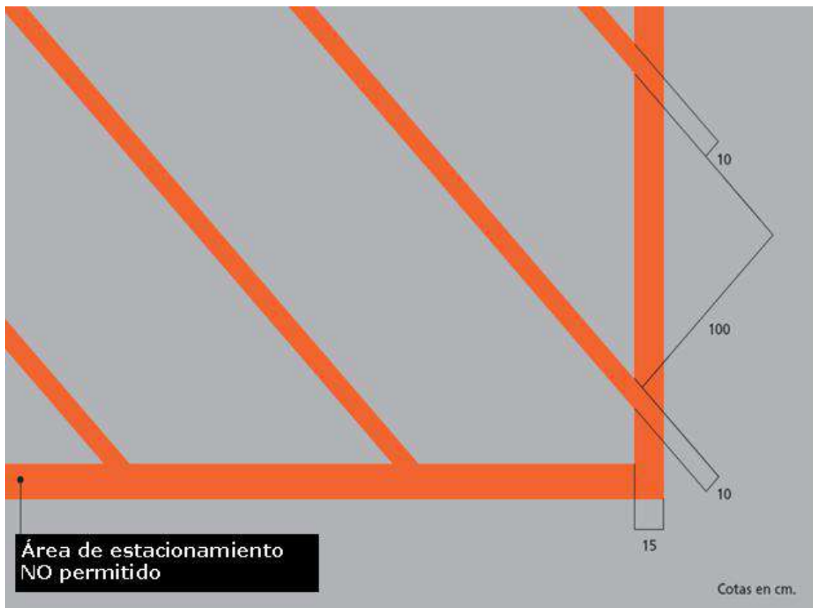
Figura 2-9-1 Señal de área de prohibición de estacionamiento NPL
