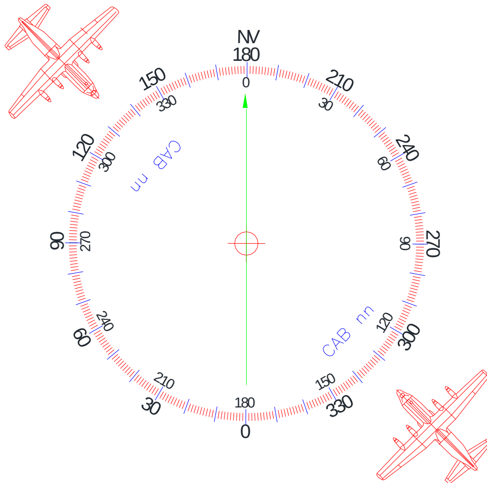
Figura 6-1. Rosa de vientos
