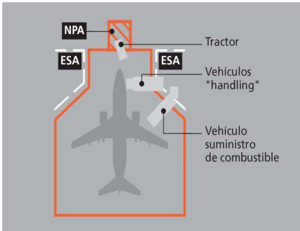
Figura 2-25-4. NPA delante del morro de la aeronave
