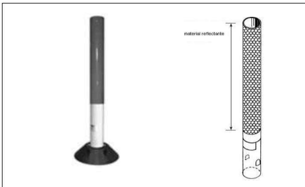
Figura 3-1 Balizas de borde de calle de rodaje
