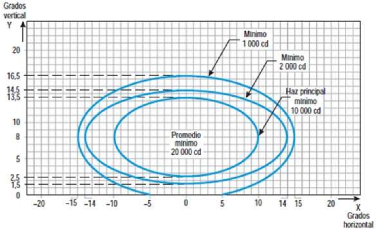
Figura ADJB-1. Diagrama de isocandelas para las luces de eje y barras transversales de aproximación (luz blanca)
