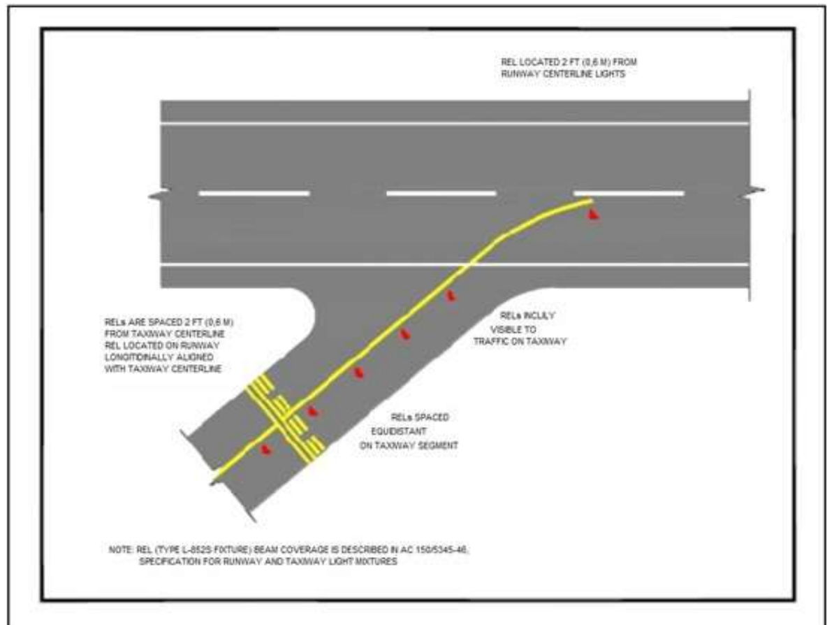
Figura 1-41-3 Sistema REL en ángulo.
