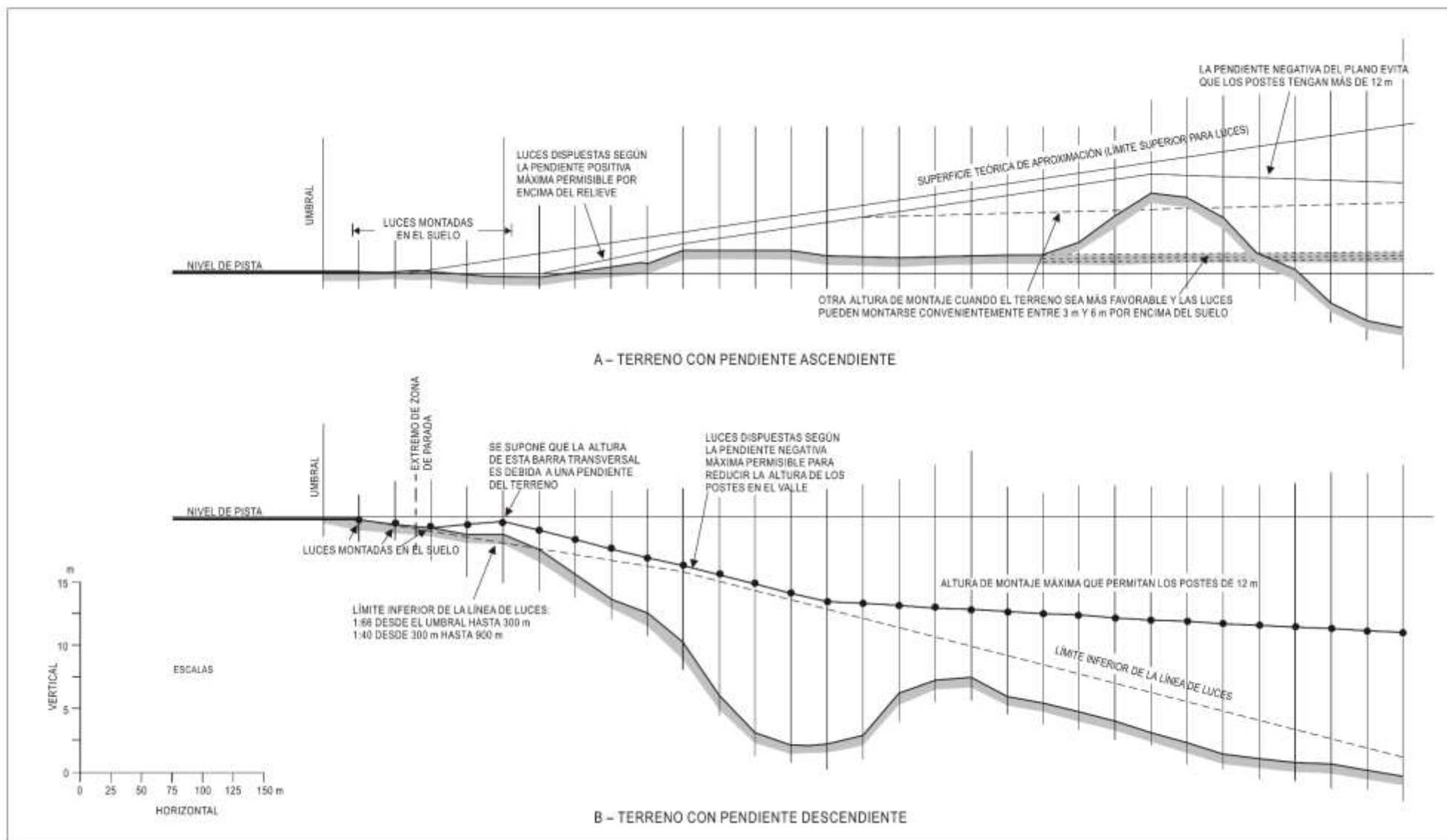
Figura ADJF-4. Tolerancias verticales de instalación
