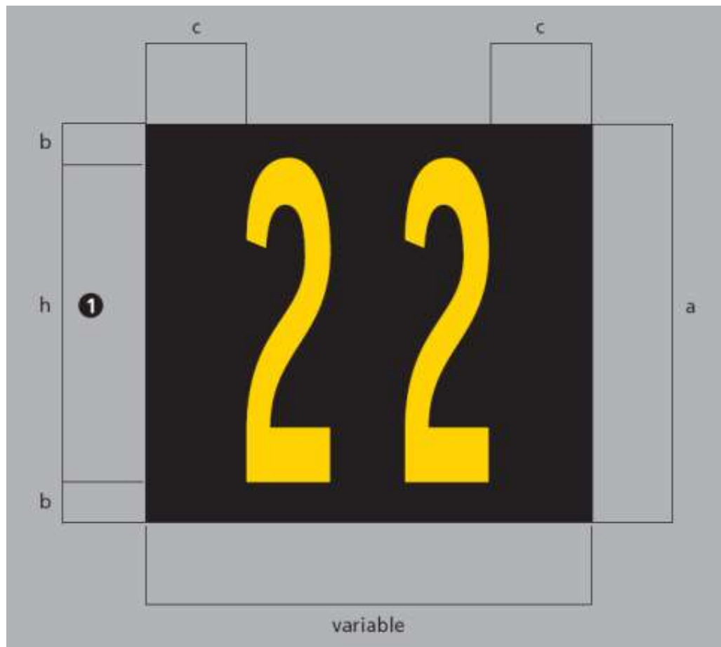
Figura 2-19-1 Señal de designación del puesto de estacionamiento
