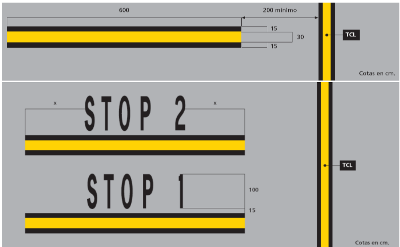
Figura 2-18-1. Señal de Barra de Parada
