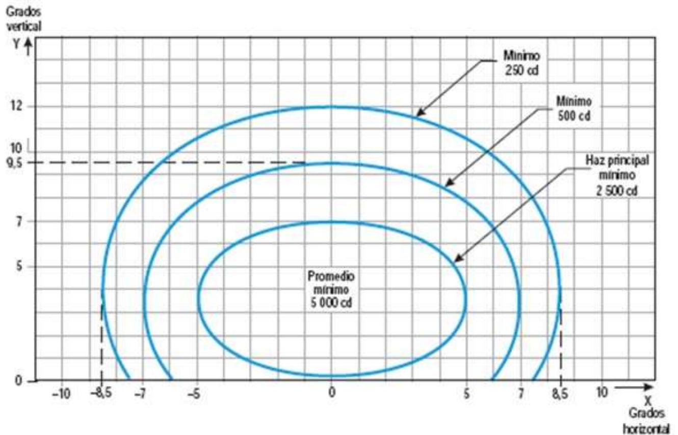
Figura ADJB-6. Diagrama de isocandelas para las luces de eje de pista con espaciado longitudinal de 30 metros (luz blanca) y luces indicadoras de calle de salida rápida (luz amarilla)
