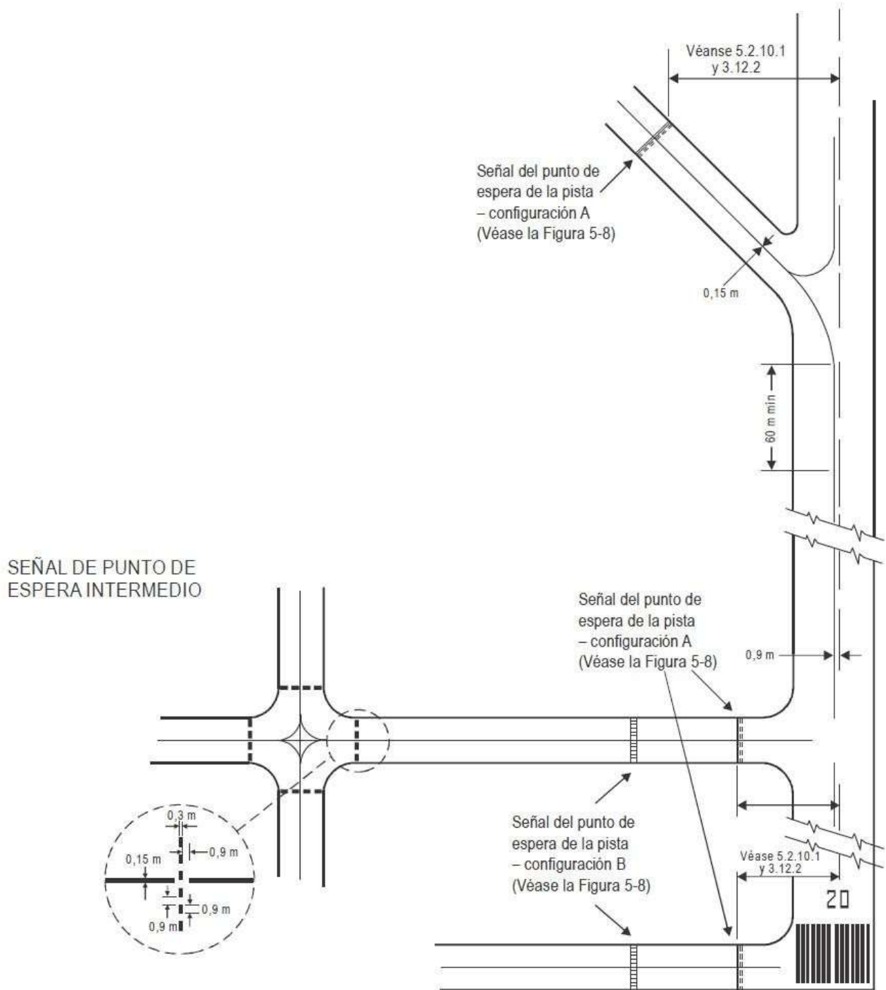
Figura 3-5-1. Grupo de señales de las calles de rodaje
