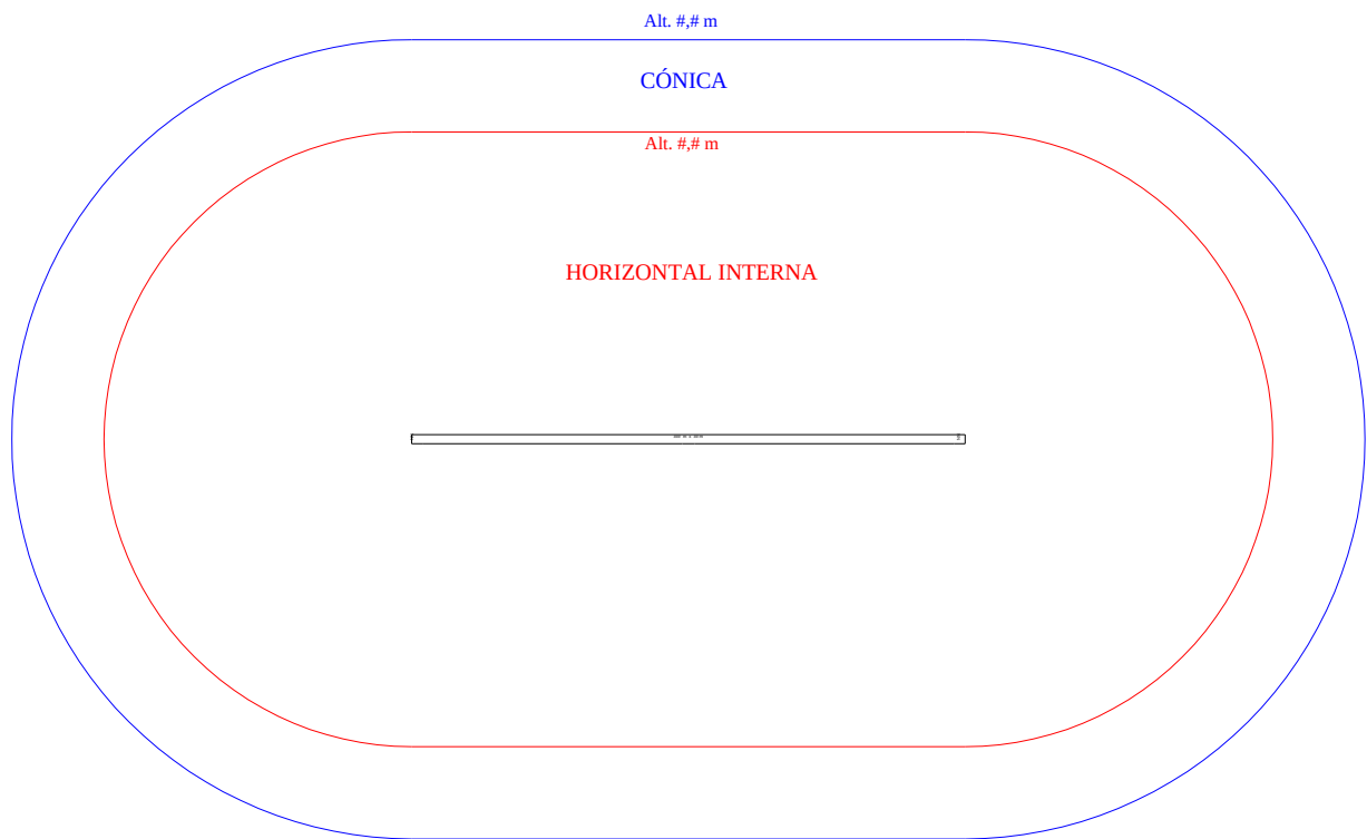
Figura 6-15. Superficie Cónica
