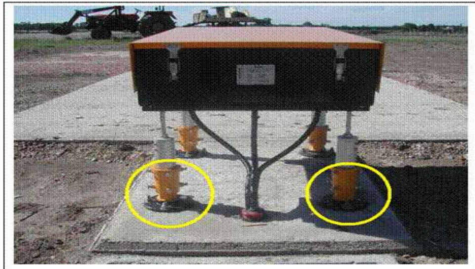
Figura ADJB-8. Ejemplos de cuplas Frangibles en las instalaciones del PAPI
