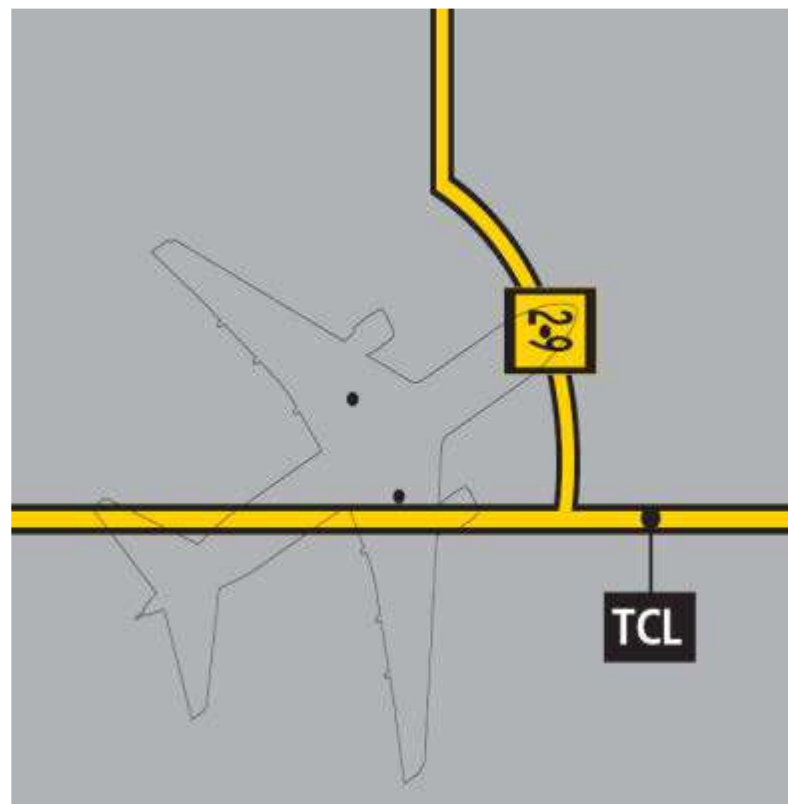
Figura 2-11-3. Señal de entrada a puestos de estacionamiento de aeronaves, desplazada.
