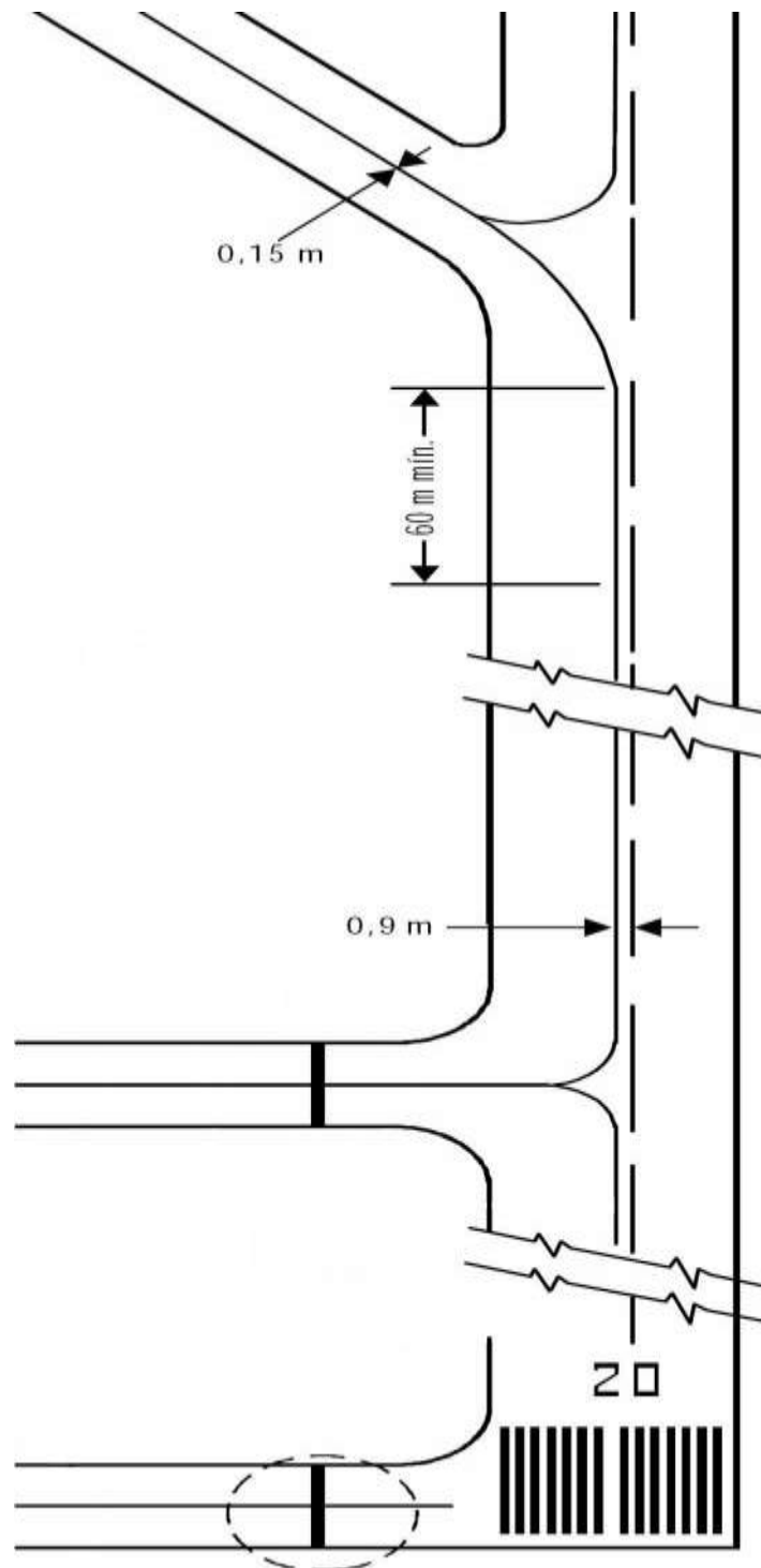
Figura 3-1-1. Señal de eje de calle de rodaje
