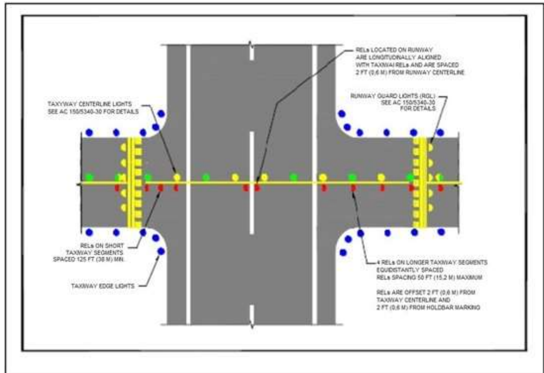
Figura 1-41-2 Sistema REL en ángulo 90°
