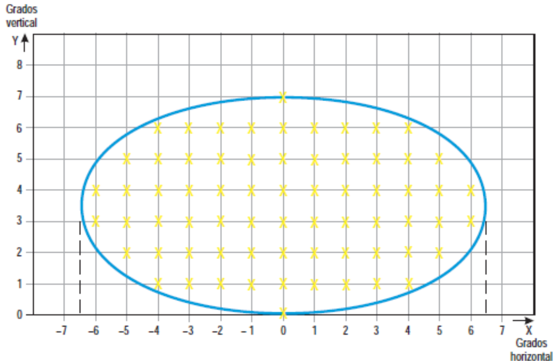
Figura ADJB-11. Puntos de cuadrícula para el cálculo de la intensidad media de luces de aproximación y de pista
