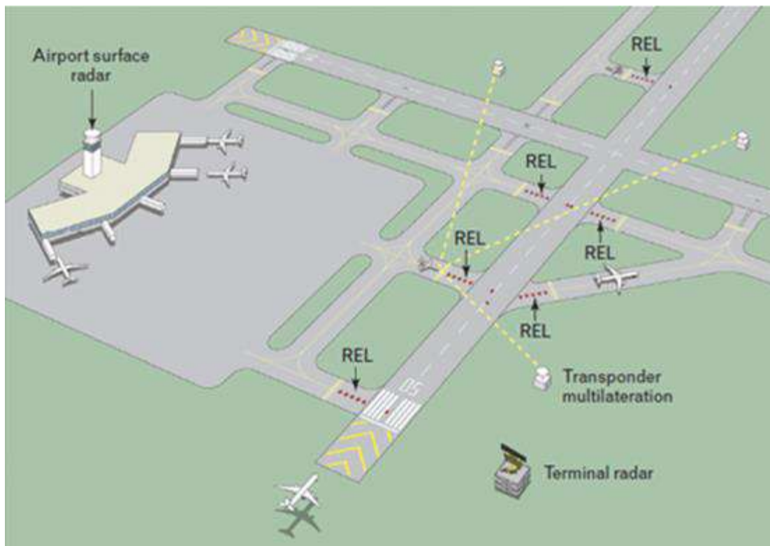
Figura 1-41-1 Sistema autónomo de advertencia de incursión en la pista (ARIWS) Emplazamiento
