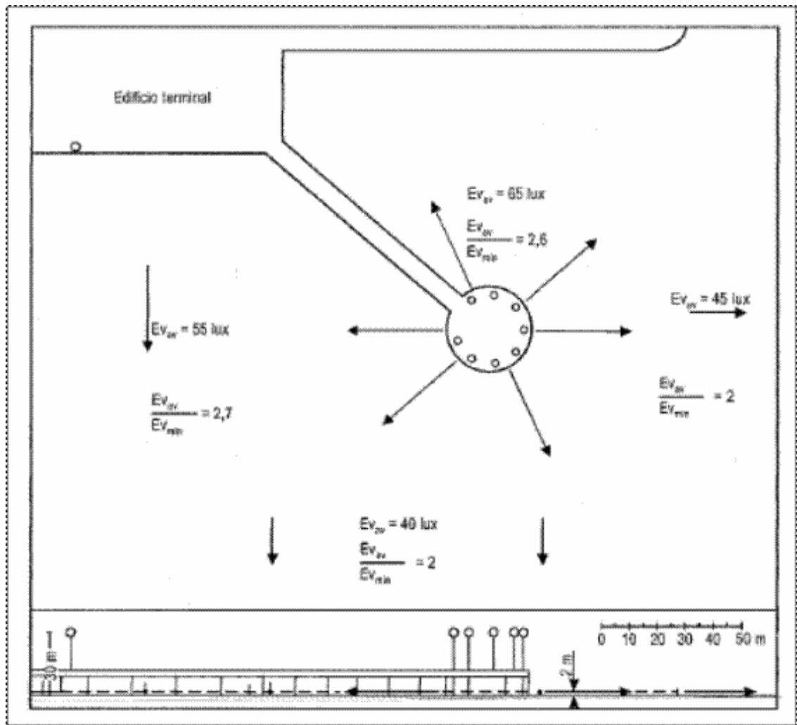
Figura ADJM-5. Promedio característico de luminancia vertical a 2 metros de altura (Ejemplo B)
