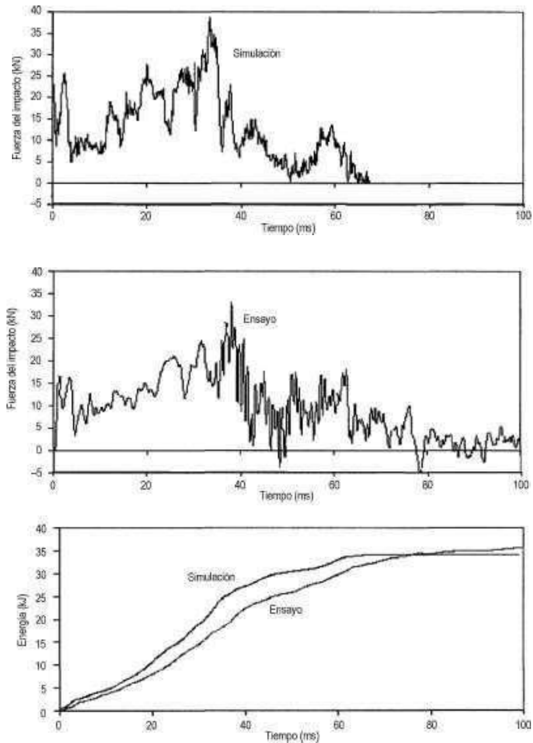
Figura ADJA-5. Fuerza y energía del impacto — velocidad del impacto 140 km/h; impacto en el ápice; masa máxima 5,44 kg; aparato impactante rígido
