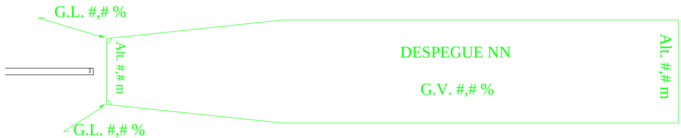
Figura 6-12. Superficie de Despegue
