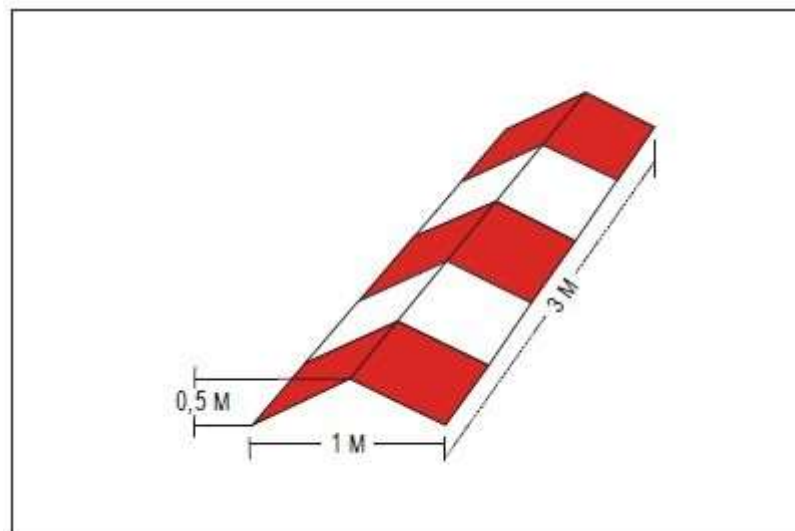
Figura 9-1 Balizas delimitadoras
