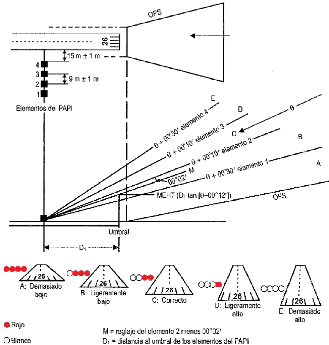
Figura 1-10-5. Disposición de los elementos del APAPI
