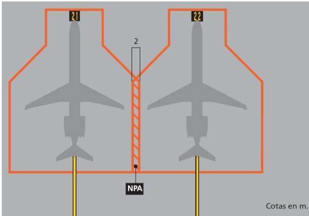
Figura 2-26-1. Solape de puestos de estacionamiento
