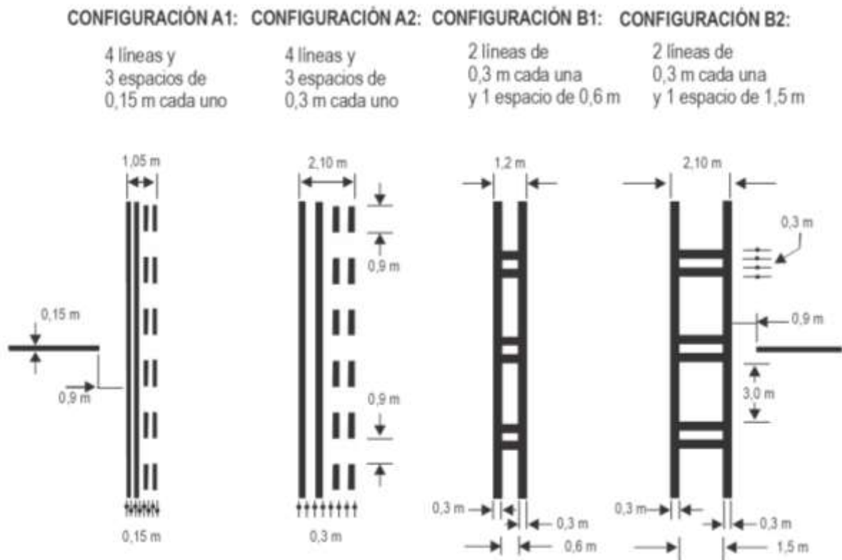
Figura 3-5-2. Señales del punto de espera de la pista
