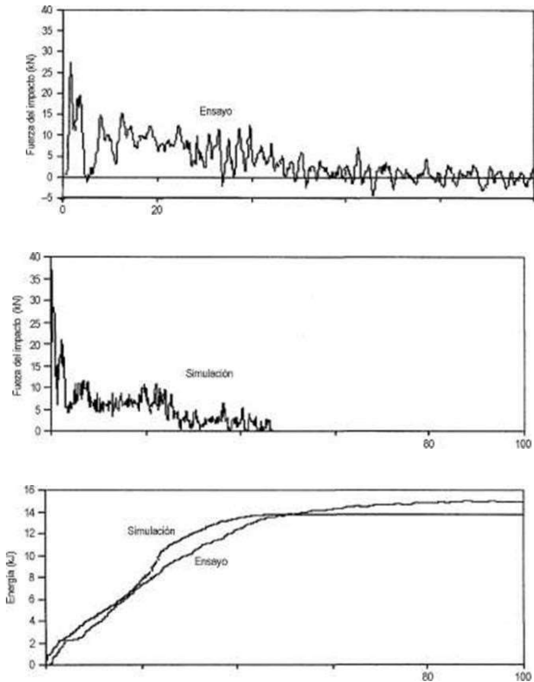
Figura ADJA-4. Fuerza y energía del impacto — velocidad del impacto 140 km/h; impacto lateral; aparato impactante rígido
