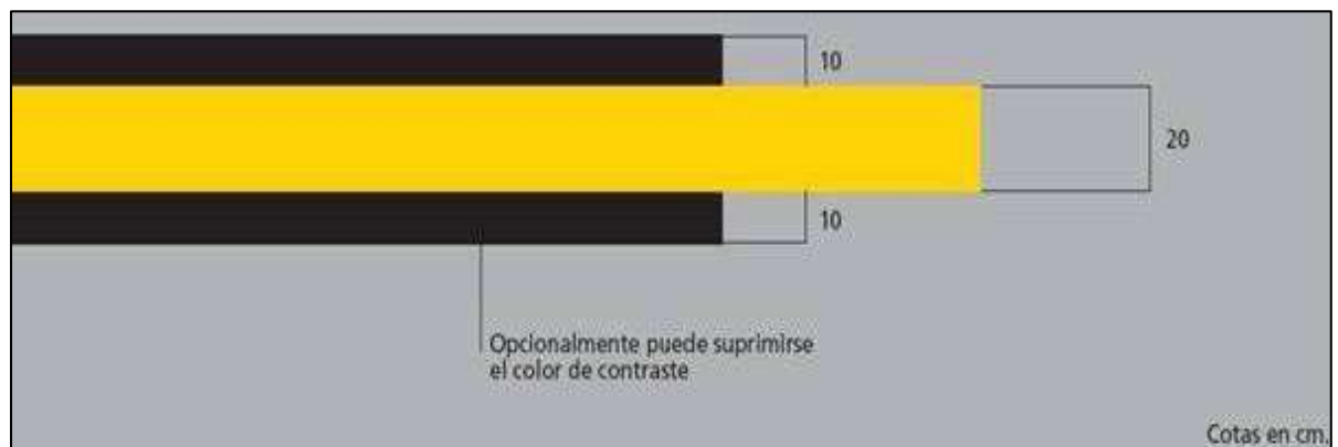
Figura 2-2-1. Señal de eje de calle de rodaje en plataforma (TCL)
