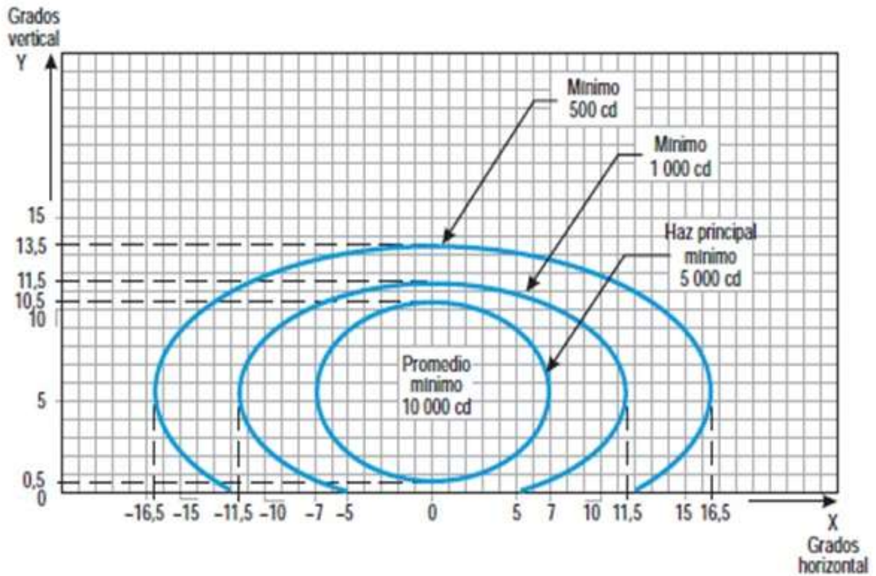
Figura ADJB-4. Diagrama de isocandelas para las luces de barra de ala de umbral (luz verde)
