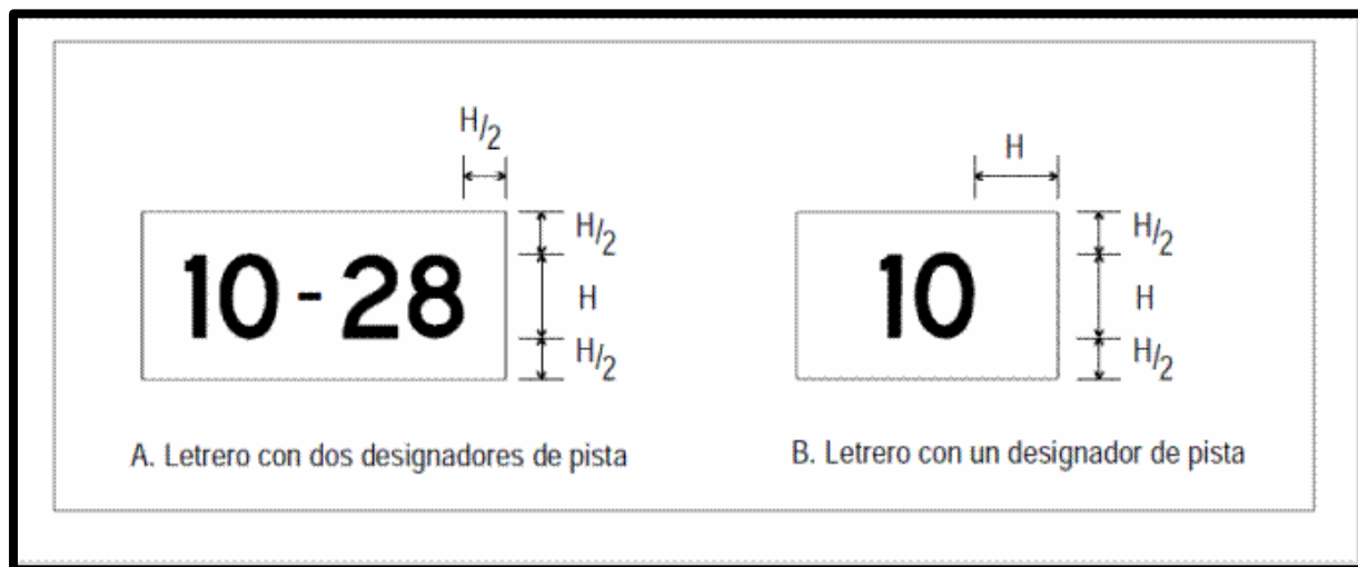
Figura ADJD-7. Dimensiones de los letreros
