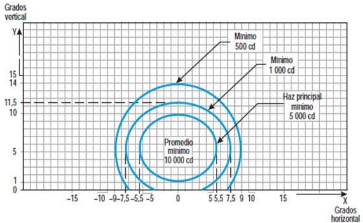
Figura ADJB-3. Diagrama de isocandelas para las luces de umbral (luz verde)
