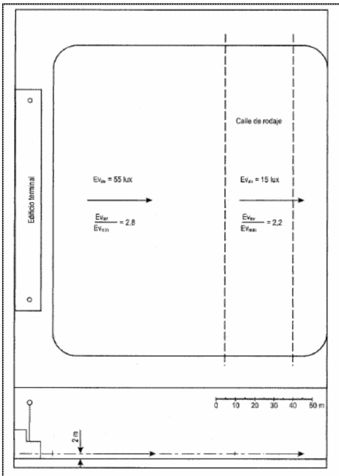
Figura ADJM4. Promedio característico de luminancia vertical a 2 metros de altura (Ejemplo A)
