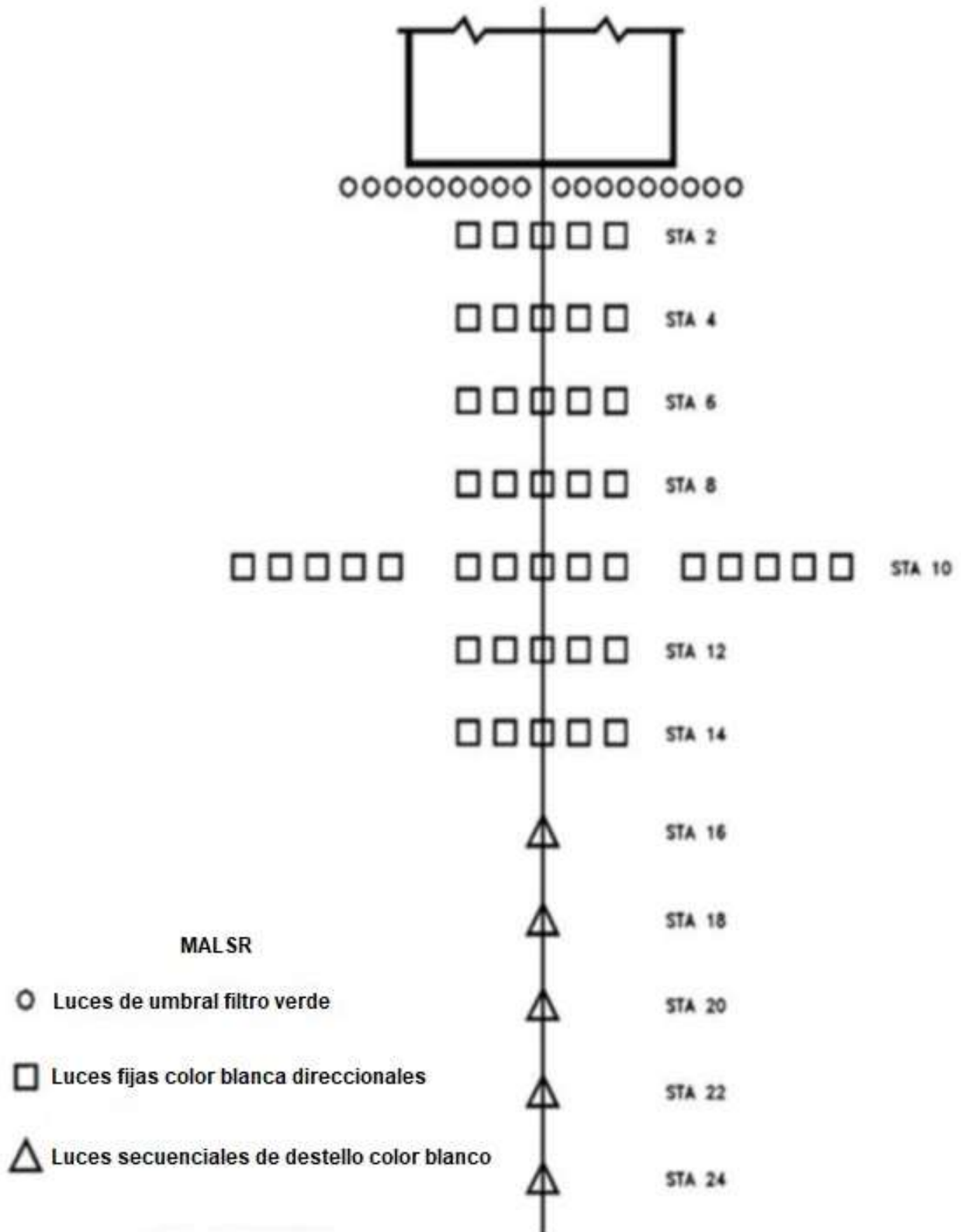
Figura 1-6-1. Diagrama esquemático del Sistema MALSR CAT I
