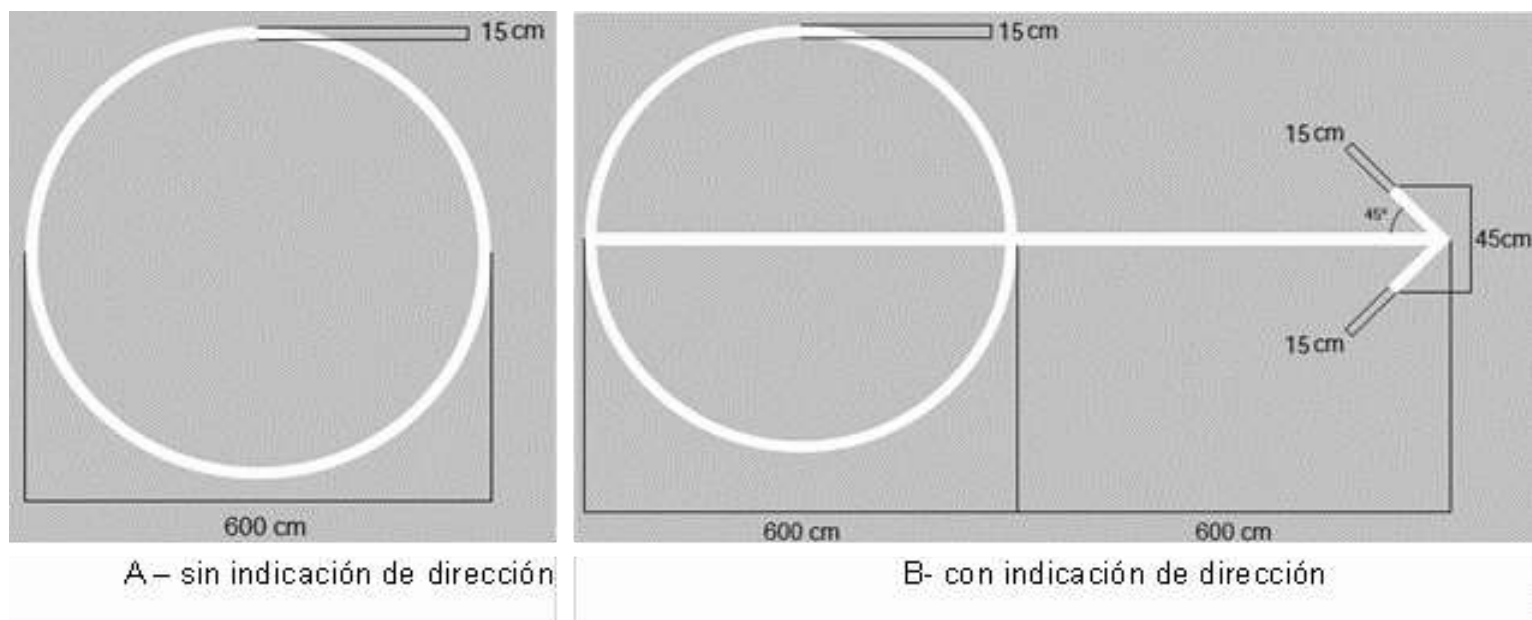
Figura 3-7-1. Señal de punto de verificación del VOR en el aeródromo
