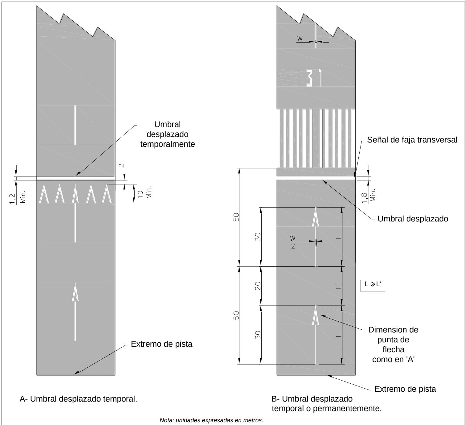
Figura 1-4-1. Señales de umbral desplazado
