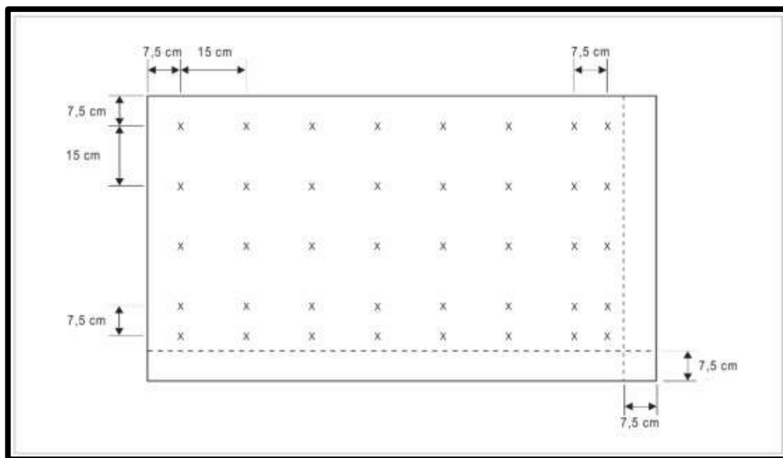
Figura ADJD-1. Puntos de retícula para calcular el promedio de luminancia de un letrero
