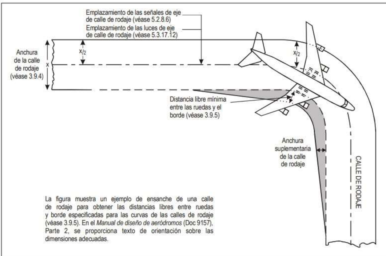
Figura 1-19-2 Curva de la calle de rodaje
