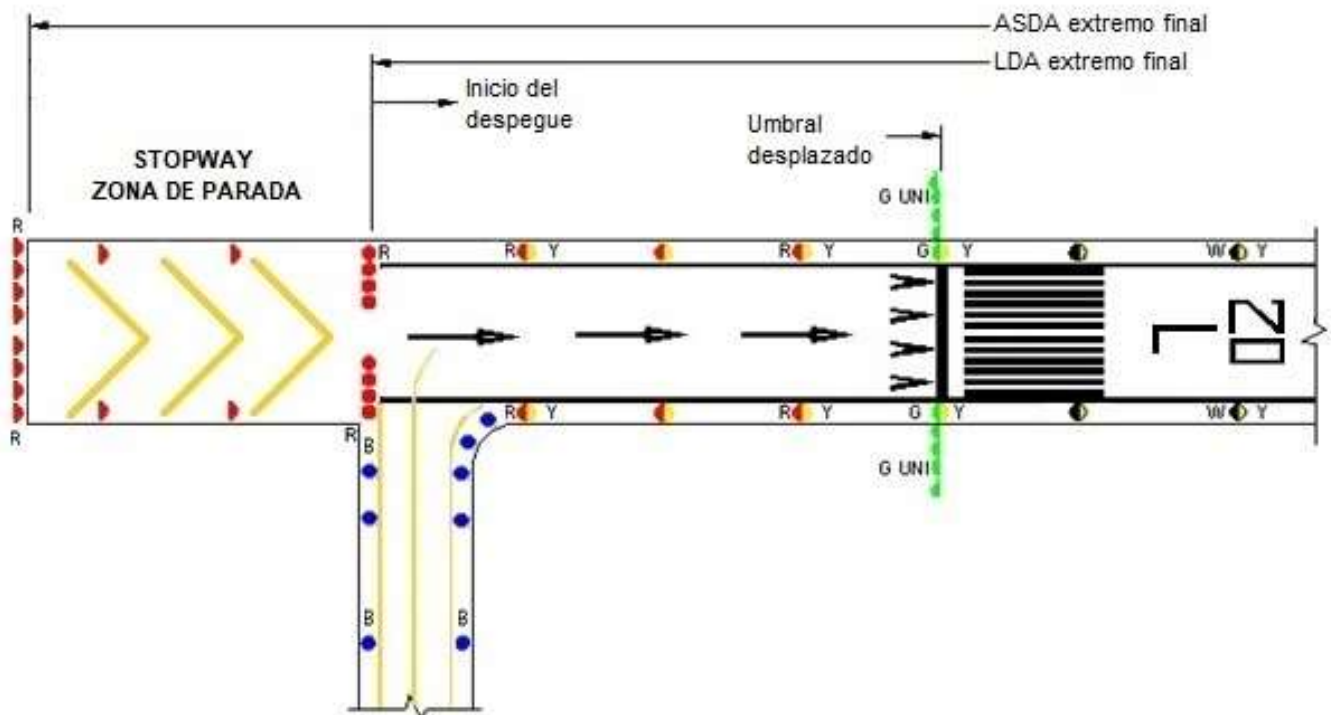
Figura 1-17-3. Disposición de las luces pista y luces de zona de parada
