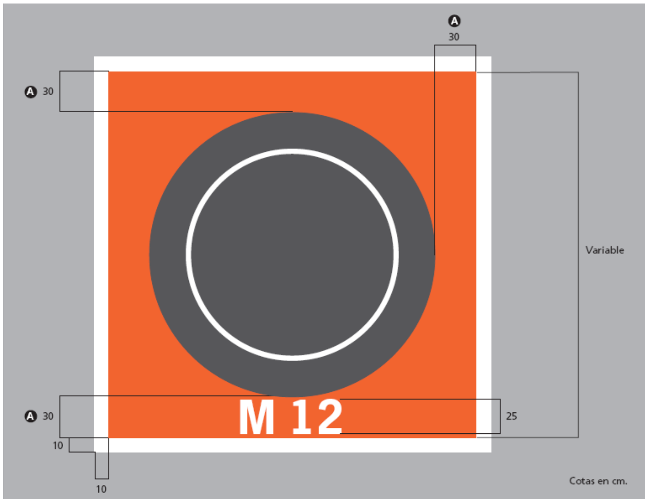
Figura 2-22-1. Señal de instalación en plataforma
