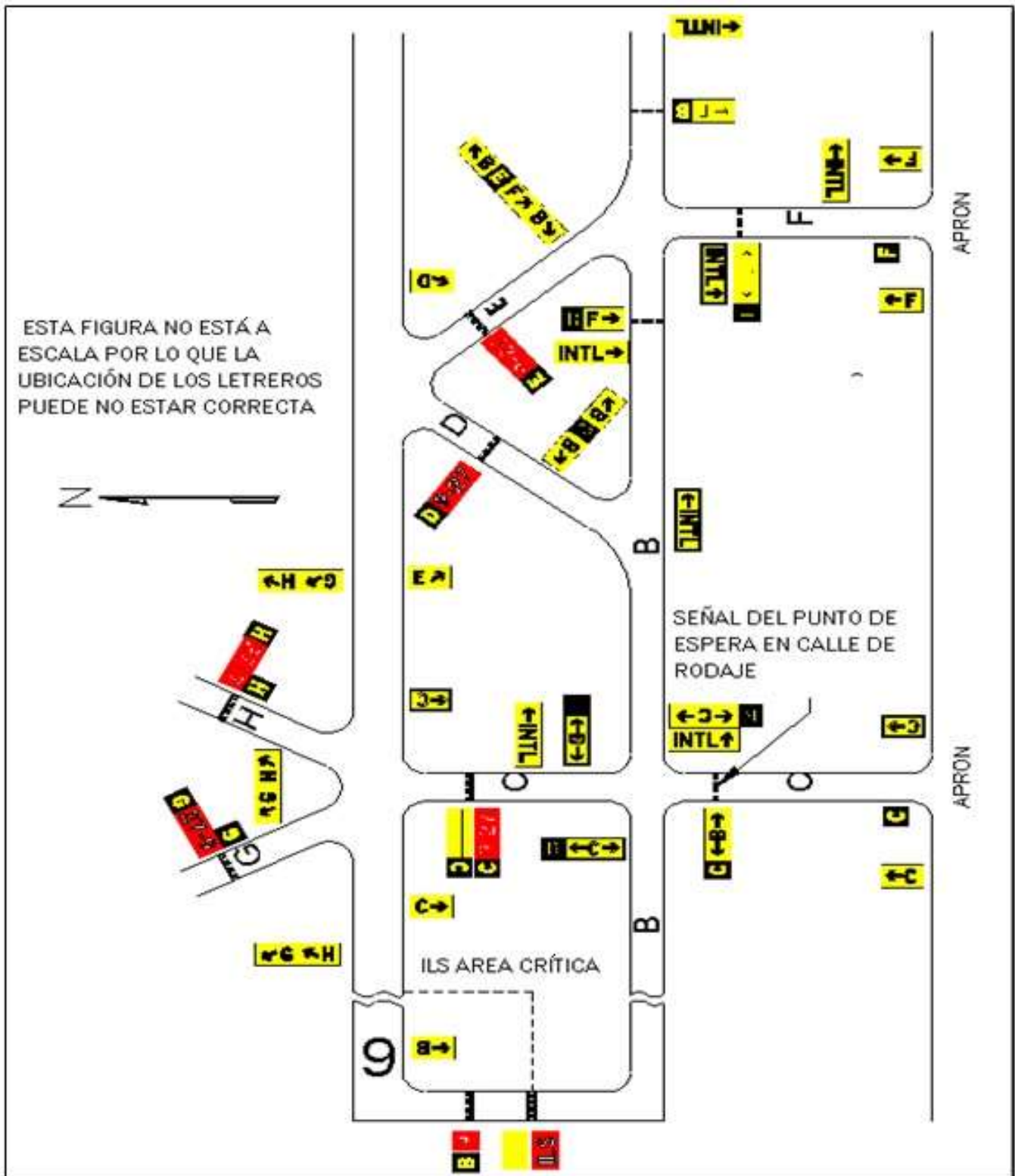
Figura 8-3-3. Caso C - Configuración Letreros
