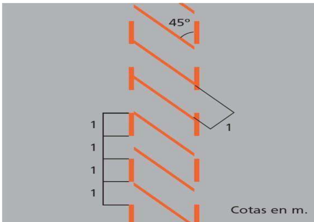
Figura 2-26-2. En caso de solape, la NPL será discontinua
