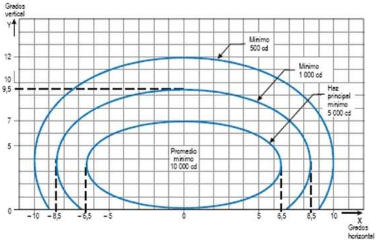
Figura ADJB-9. Diagrama de isocandelas para las luces de borde de pista cuando el ancho de la pista es de 45 metros (luz blanca)
