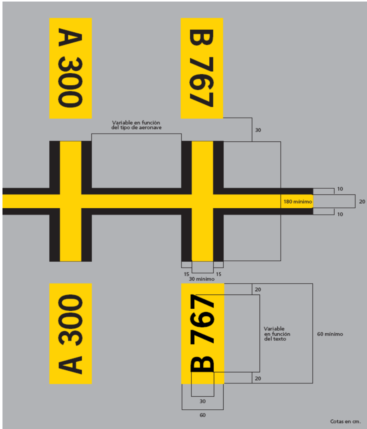
Figura 2-21-1. Barra de rueda de proa e indicación del tipo de aeronave
