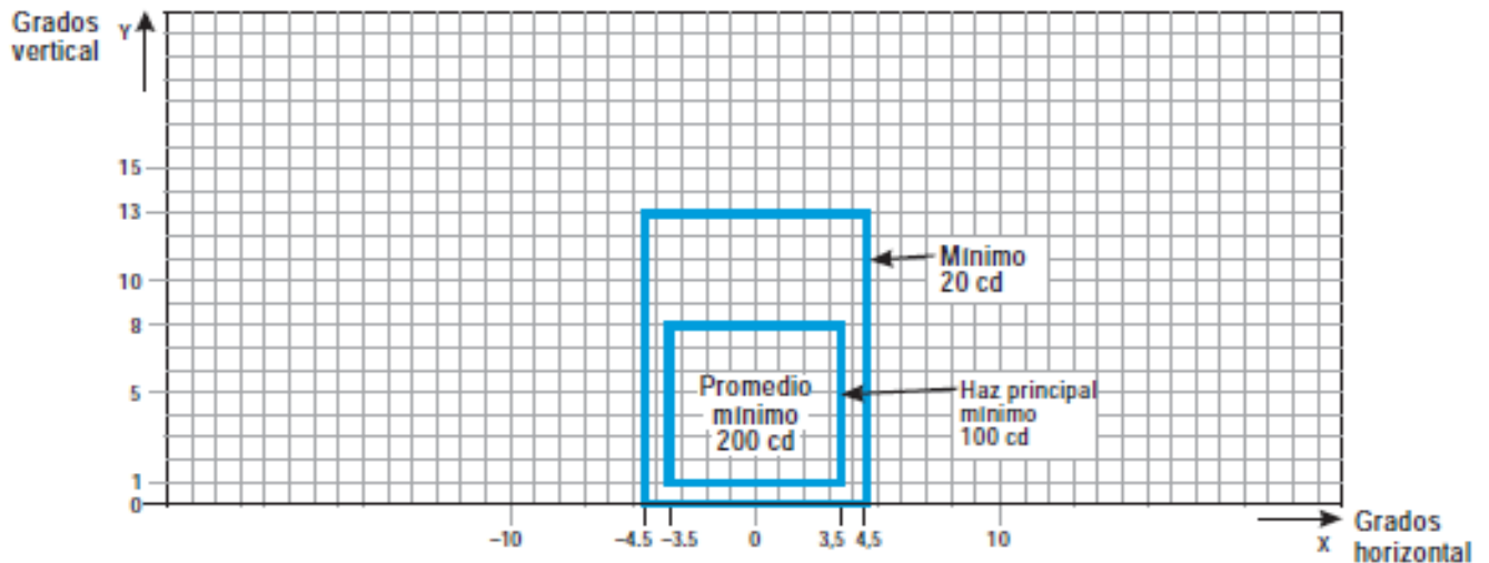
Figura ADJB-13. Diagrama de isocandelas para luces de eje de calle de rodaje espaciado de 15 metros), de barra de prohibición de acceso y de barra de parada en tramos rectos previstas para ser utilizadas en condiciones de alcance visual en la pista inferior a un valor de 350 m
