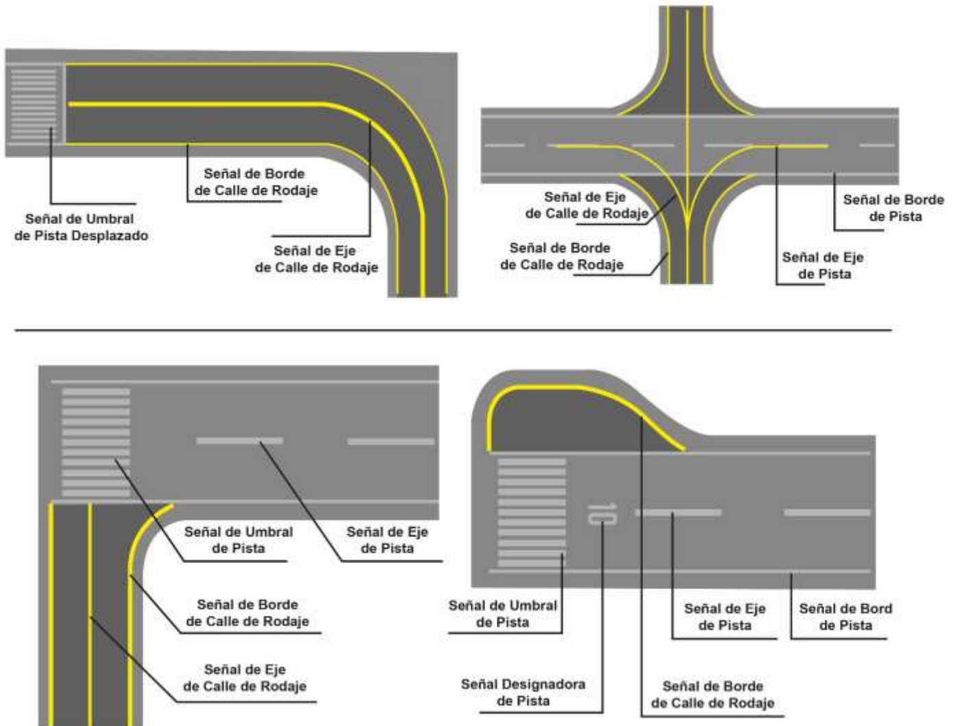
Figura 3-3-3. Ejemplos de Señales de faja lateral y eje de rodajes.
