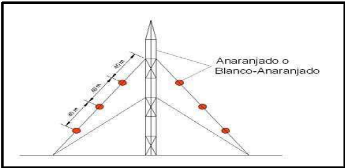
Figura 4-4. Señalamiento de las riendas para la erección de los mástiles de líneas de tensión con esferas de colores
