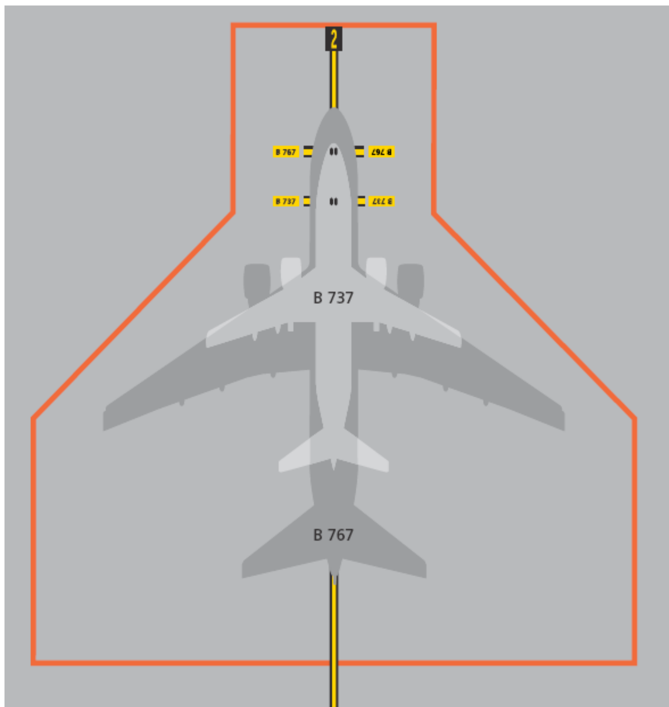
Figura- 2-25-1. Flota usuaria de cada puesto de estacionamiento
