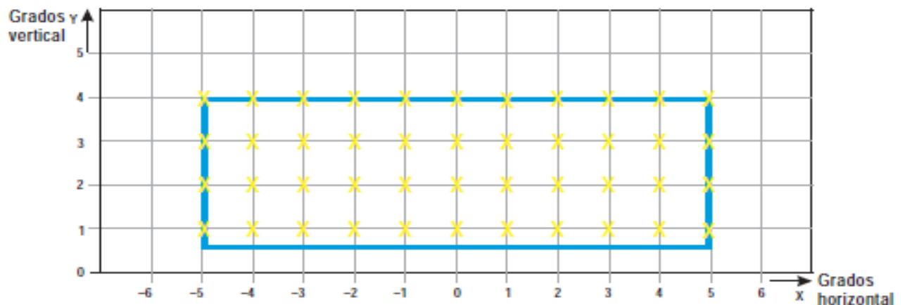
Figura ADJB-21. Puntos de cuadrícula para el cálculo de la intensidad media de luces de eje de calle de rodaje y de luces de barra de parada
