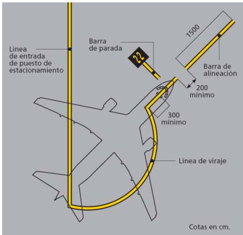
Figura 2-20-2. Señal de Barra de alineación
