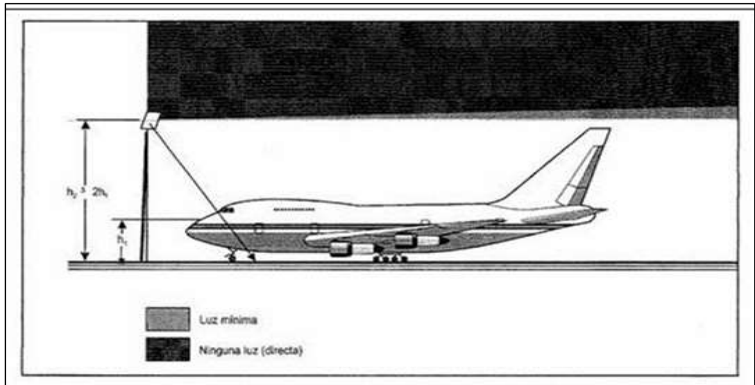
Figura ADJM-2. Altura de montaje para evitar el deslumbramiento
