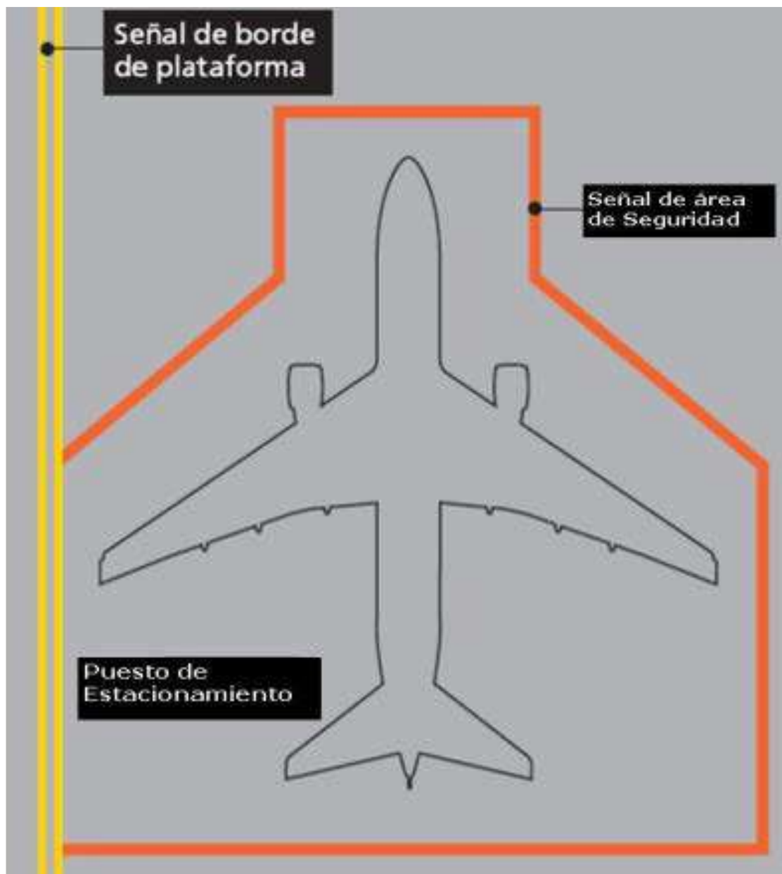
Figura 2-6-1. Área de Restricción de Equipos ERA/Área de Seguridad de la Aeronave ASA
