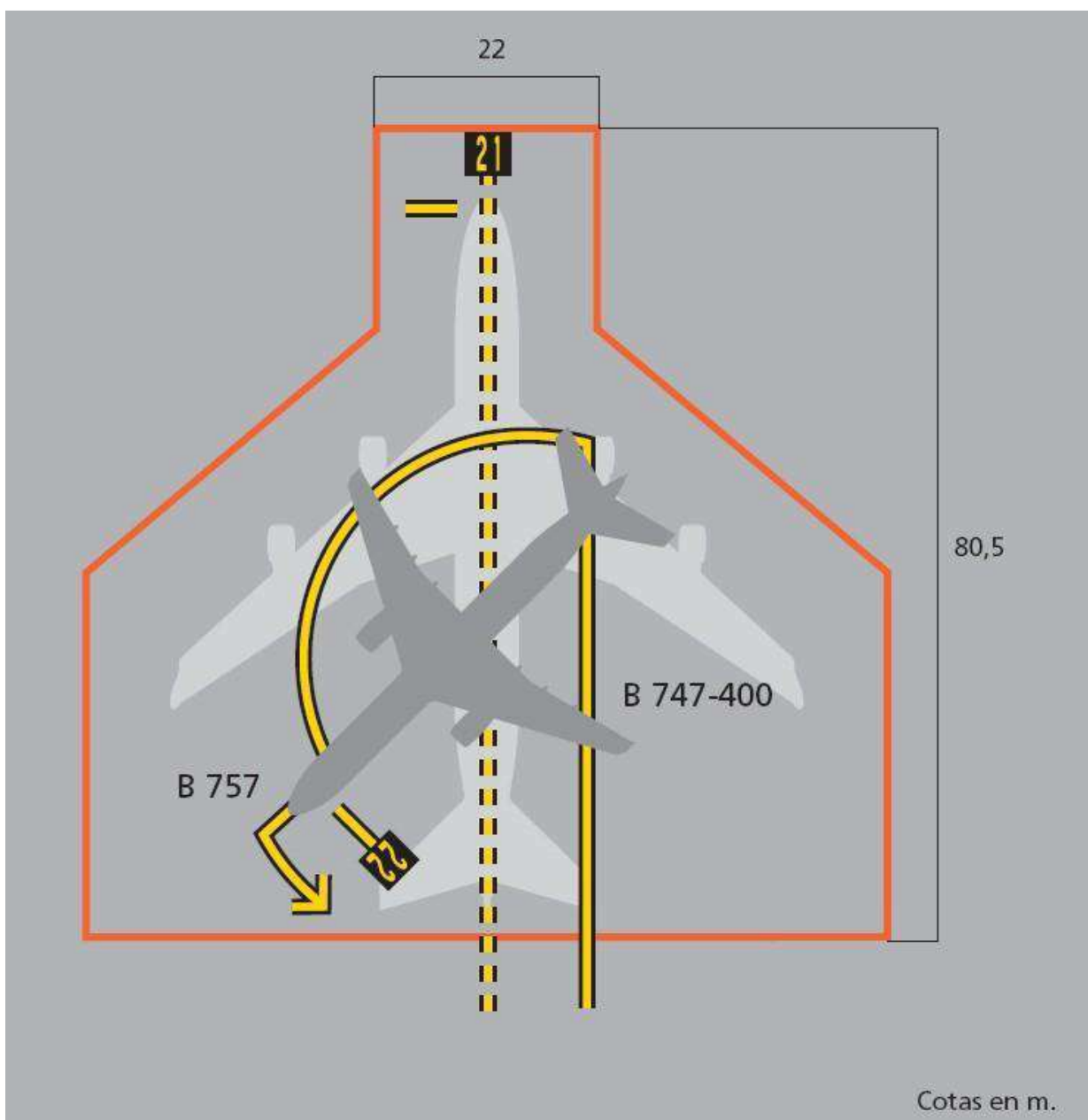
Figura 2-26-6. Estacionamientos superpuestos para distintos tipos de aeronaves.
