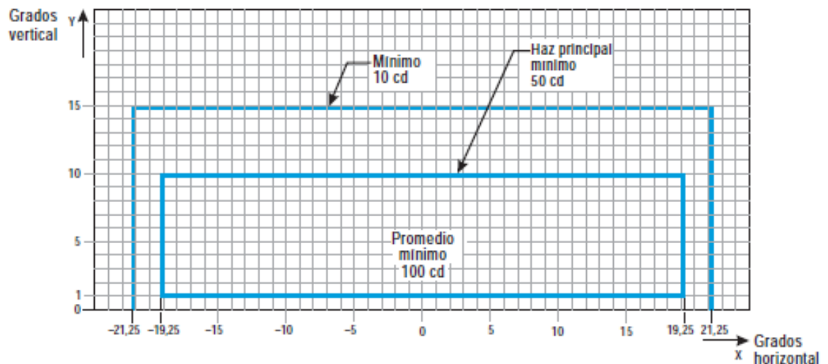
Figura ADJB-14. Diagrama de isocandelas para luces de eje de calle de rodaje (espaciado de 7,5 metros), de barra de prohibición de acceso y de barra de parada en tramos curvos para ser utilizado en condiciones de alcance visual en la pista inferior a un valor de 350 m
