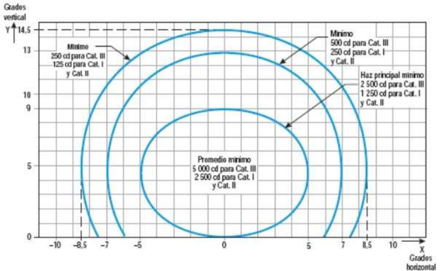
Figura ADJB-7. Diagrama de isocandelas para las luces de eje de pista con espaciado longitudinal de 15 metros (luz blanca) y luces indicadoras de calle de salida rápida (luz amarilla)
