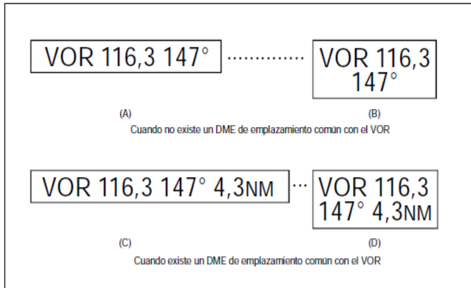
Figura 8-4-1. Letreros de punto de verificación del VOR en el aeródromo
