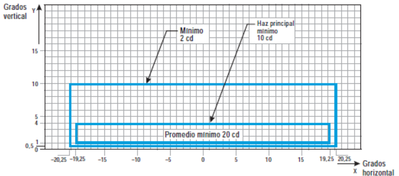
Figura ADJB-16. Diagrama de isocandelas para luces de eje de calle de rodaje (espaciado de 7,5 metros, 15 metros, 30 metros), de barra de prohibición de acceso y de barra de parada en tramos curvos previstas para ser utilizadas en condiciones de alcance visual en la pista de 350 metros o superior
