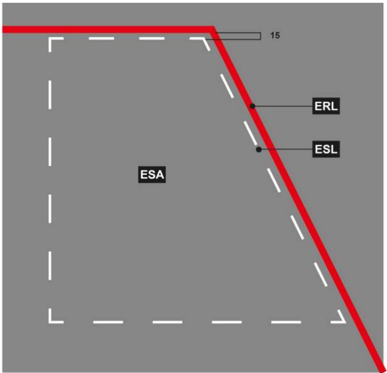
Figura 2-7-2. Señal de área de estacionamiento de equipos ESA
