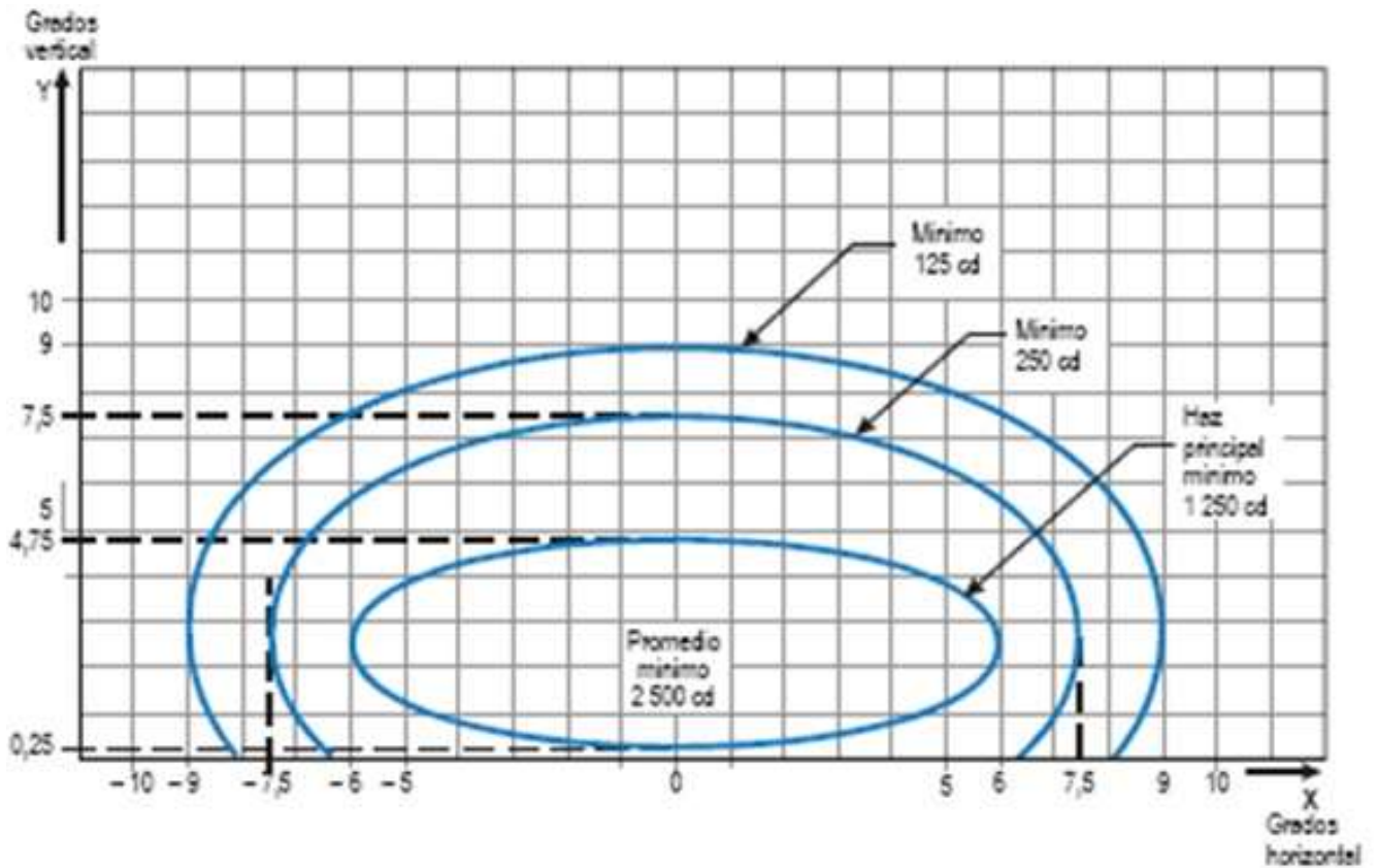
Figura ADJB-8. Diagrama de isocandelas para las luces de extremo de pista (luz roja)
