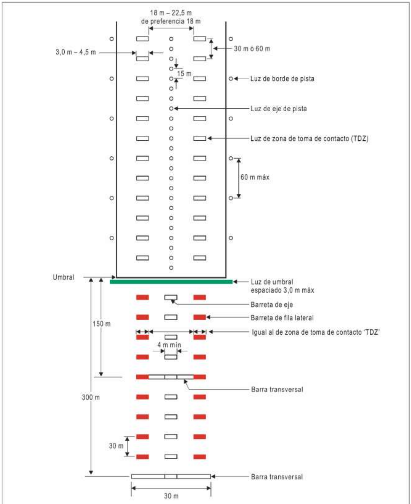
Figura 1-7-1. Iluminación de pista y de los 300 metros internos de la aproximación en las pistas para aproximaciones de precisión de Categorías II y III
