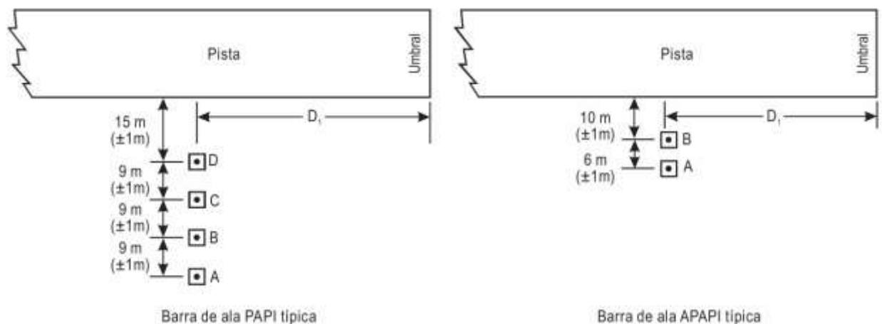
Figura 1-9-3. Emplazamiento del PAPI y APAPI
