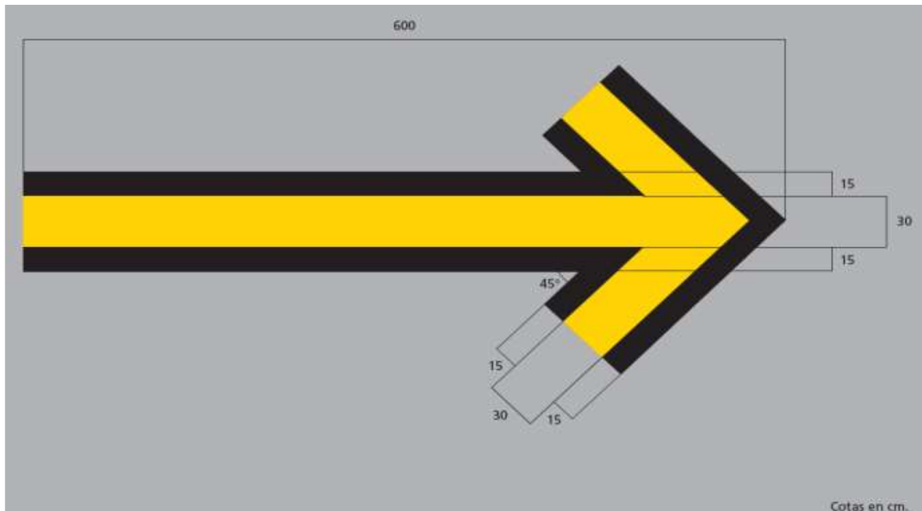
Figura 2-15-1. Señal de Barra de viraje
