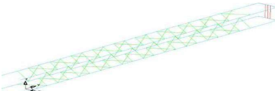
Torre de iluminación de aproximación — estructura reticular de fibra de vidrio
