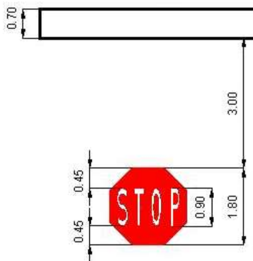
Figura 4-1-1 Señal de detención. Características y emplazamiento
