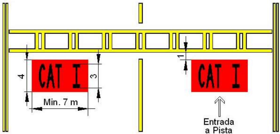
Figura 4-2-2. Señales con instrucciones obligatorias en el punto de espera intermedio de una pista de categoría 1
