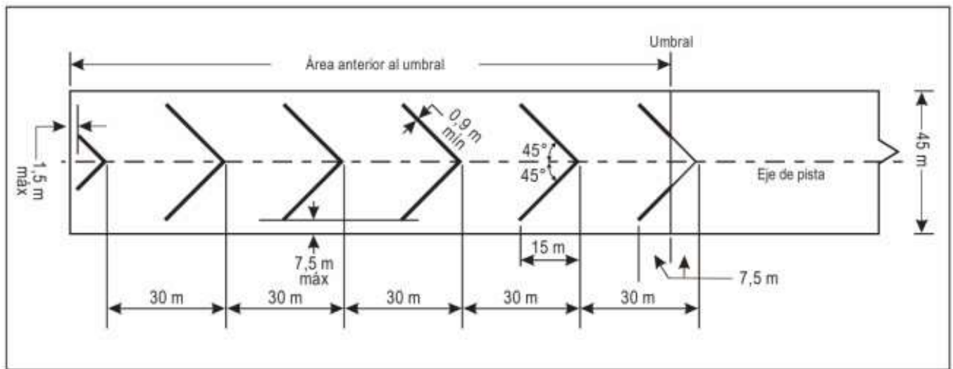
Figura 1-9-2. Señal anterior al umbral
