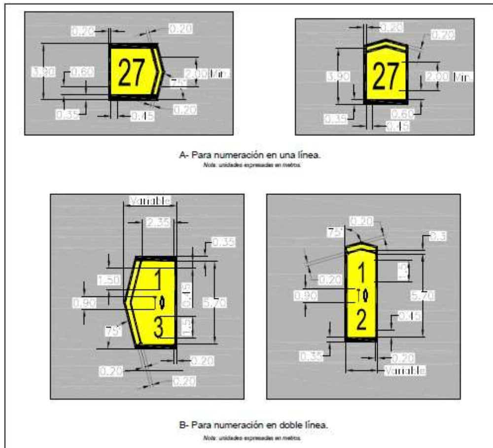
Figura 2-10-1. Señal direccional a puestos de estacionamiento de aeronaves
