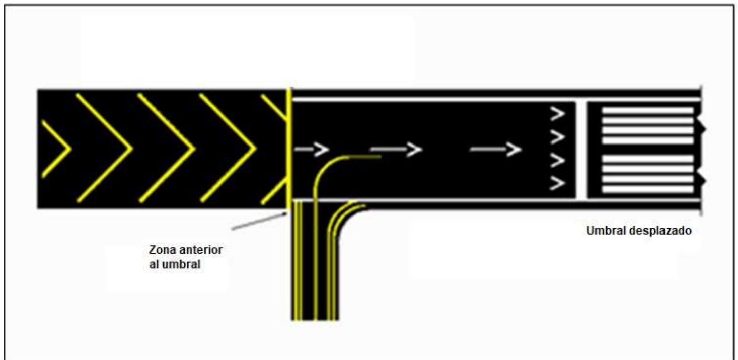
Figura 5-3-3. Señal anterior al umbral con umbral desplazado
