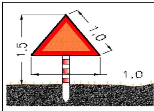
Figura 6-9-1 Detalle de las balizas de final de pistas no pavimentadas
