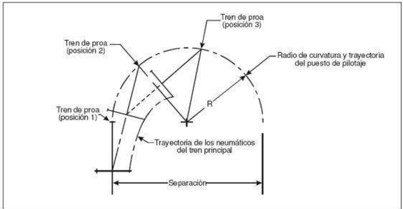
Figura 3-4-2. Solución gráfica de un viraje de 180
