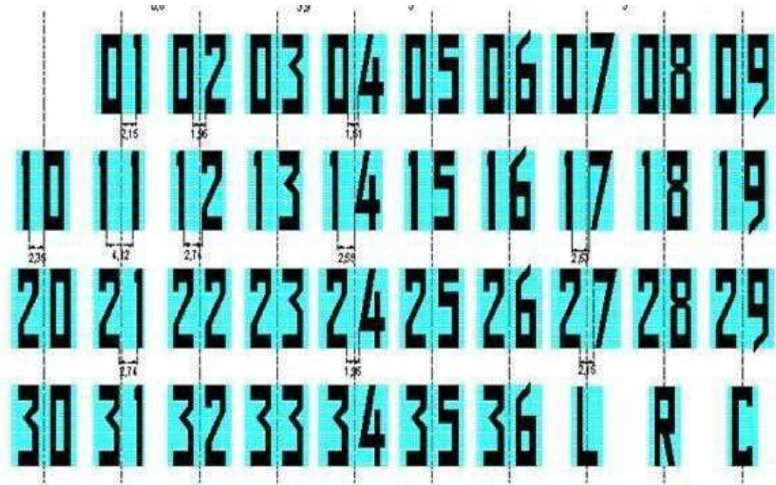
Figura 1-2-3. Caracteres para la Señal Designadora de Pista de dos números
