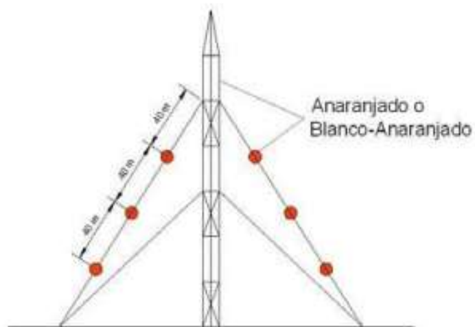
Figura 4-4. Señalamiento de las riendas para la erección de los mástiles de líneas de tensión con esferas de colores
