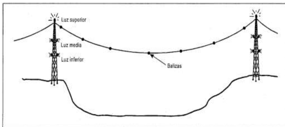
Figura ADJB-1. Ejemplos de sistemas de luces de obstáculo de elevada intensidad en torres para soporte de cables suspendidos
