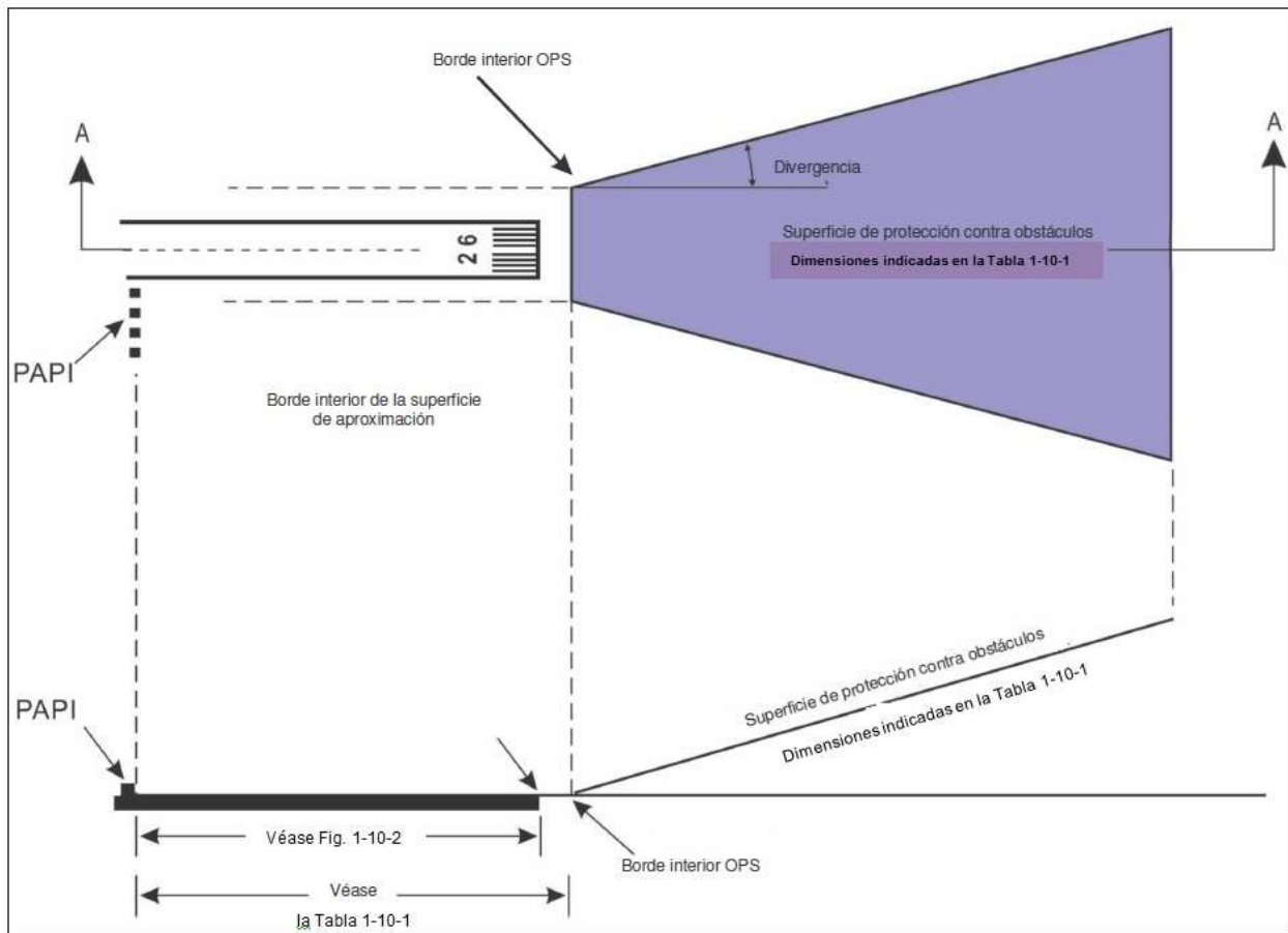
Figura 1-10-3. Superficie de protección contra obstáculos para los sistemas visuales indicadores de pendiente de aproximación
