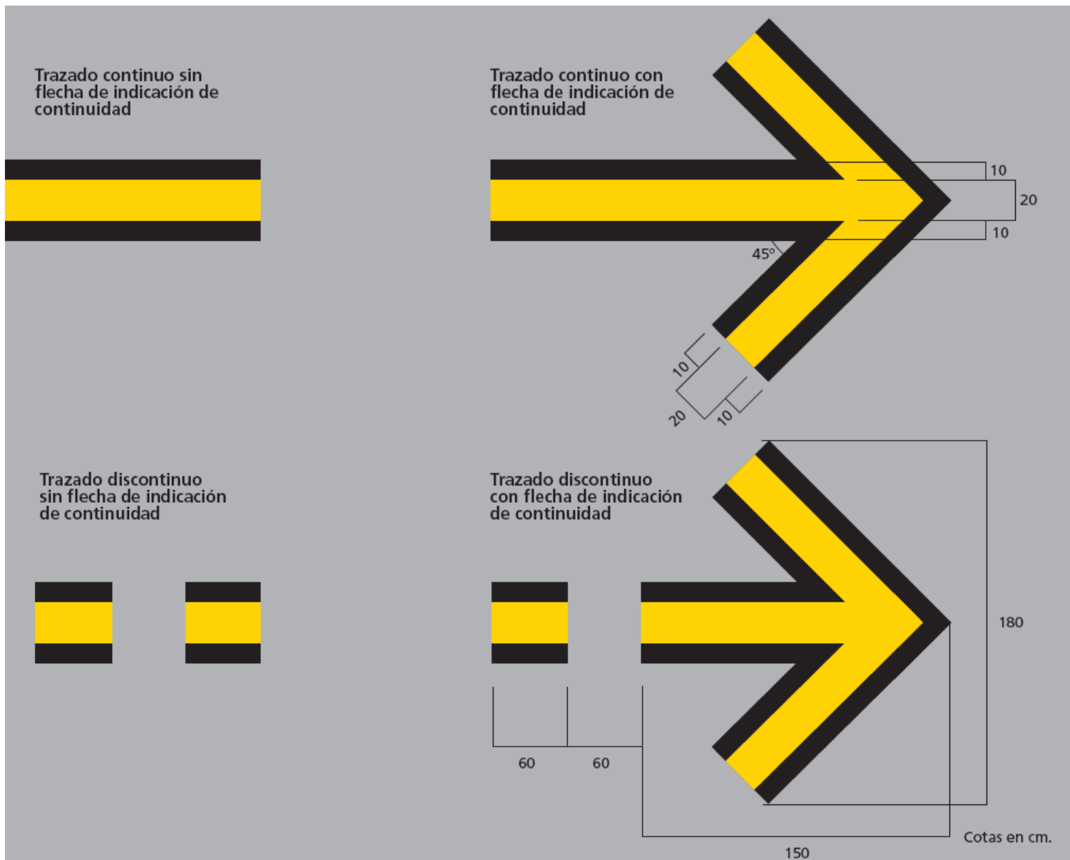
Figura 2-11-1. Señal de entrada a puestos de estacionamiento de aeronaves
