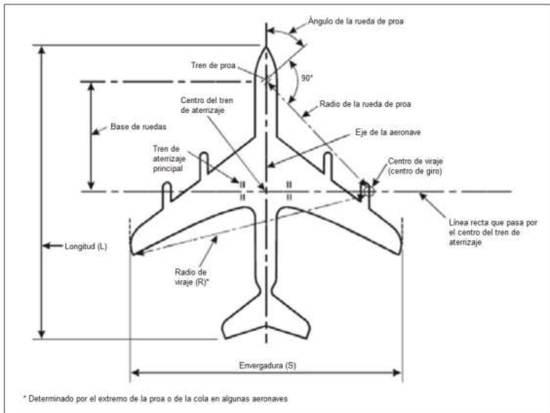
Figura 1-19-1 Base de ruedas
