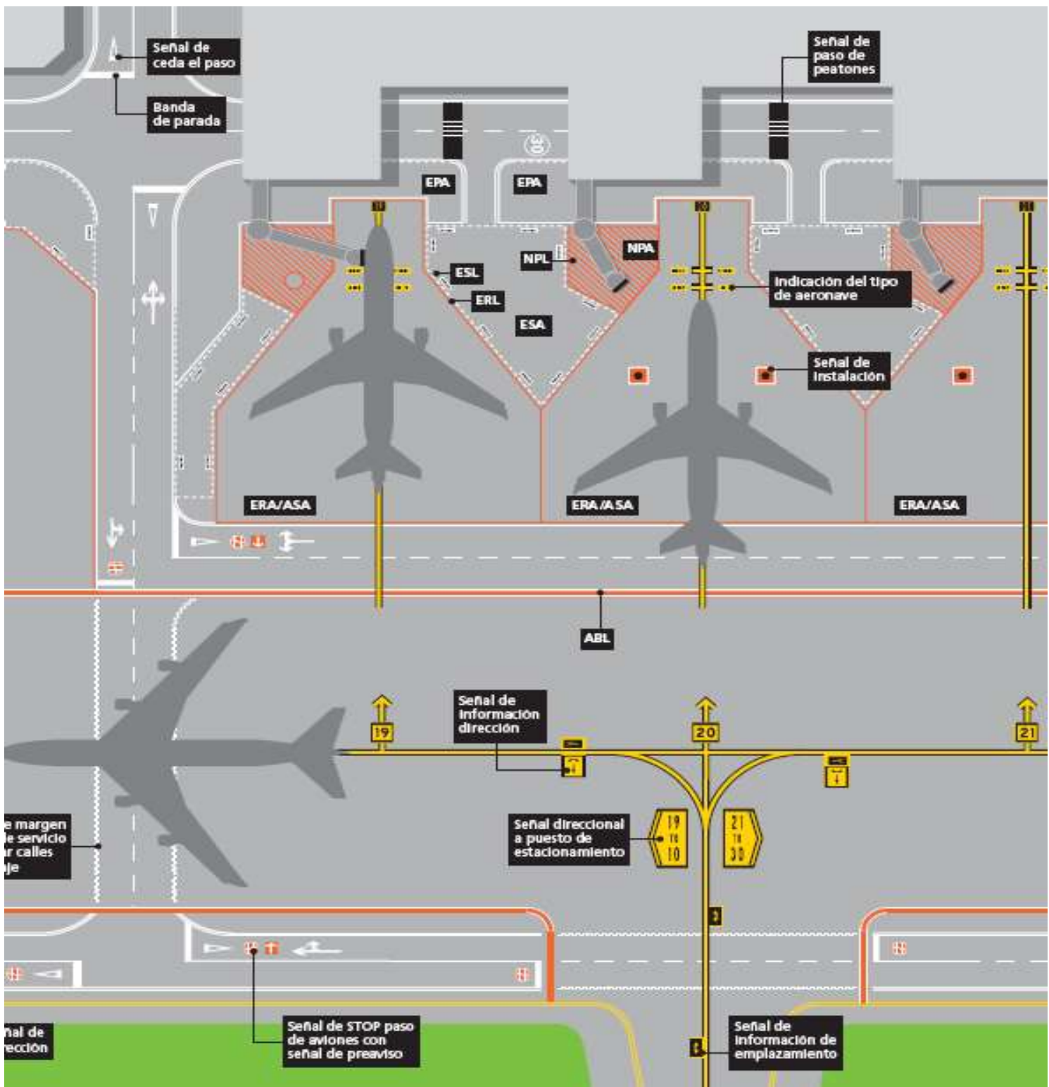
Figura 2-27-2. Sendas en la plataforma para el movimiento de personas.
