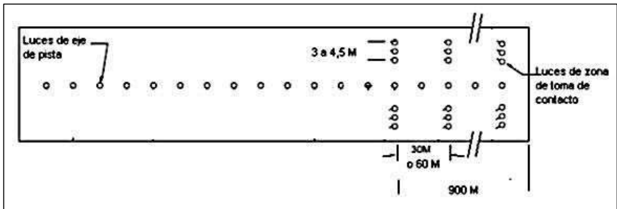
Figura 1-19-1. Luces de toma de contacto
