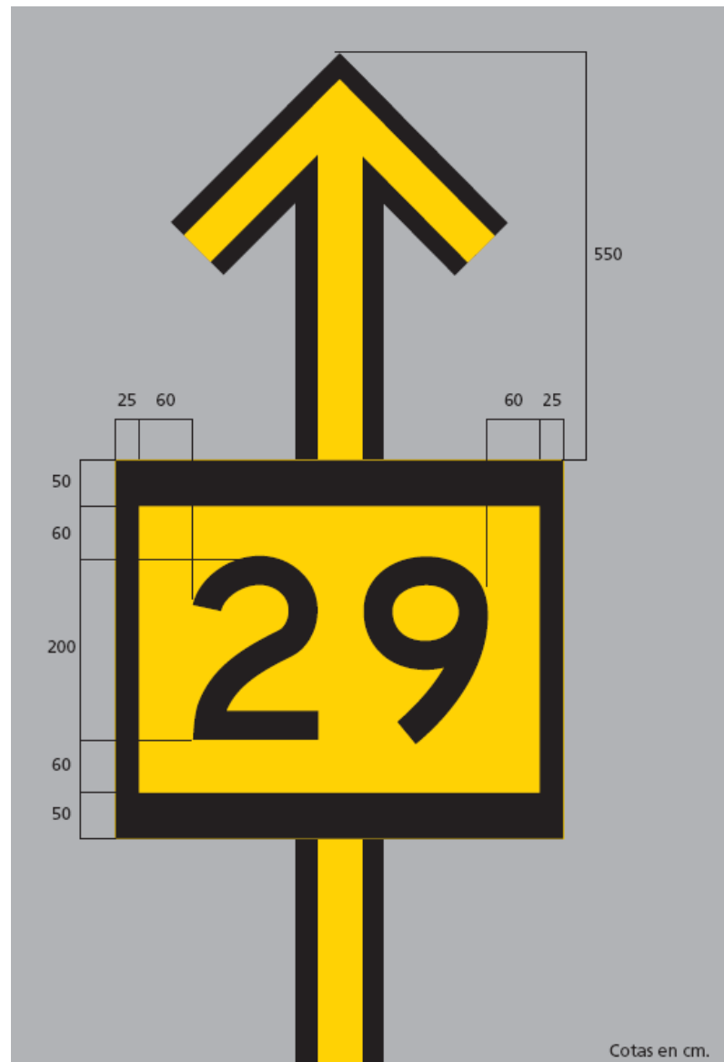
Figura 2-12-4. Identificación de puesto de estacionamiento con dos direcciones de rodajes hacia el puesto
