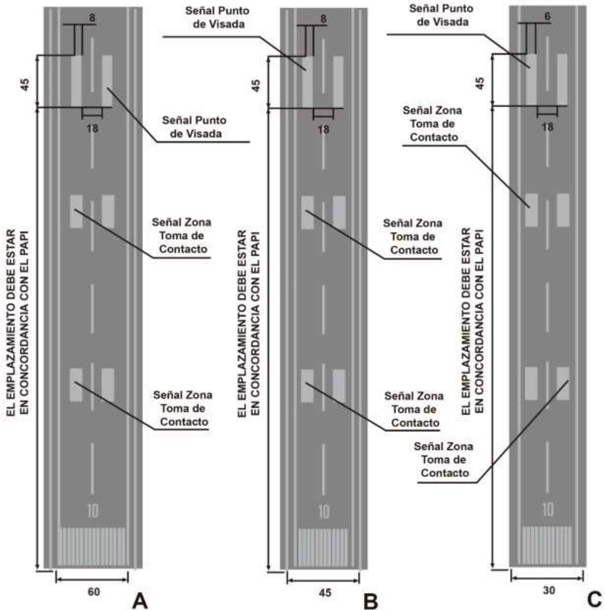
Figura 1-5-2. Señales de punto de visada y de zona de toma de contacto (Ilustradas para una pista de 60 metros, 45 metros y 30 metros de ancho)
