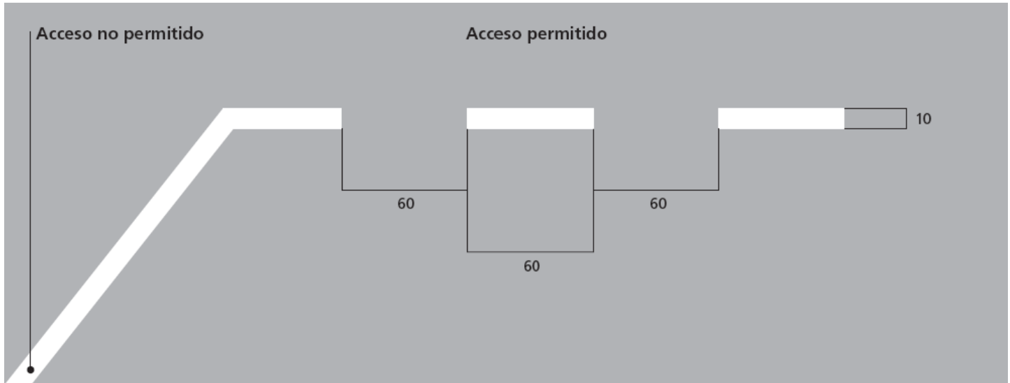
Figura 2-7-1. Señal de área de espera de equipos ESL
