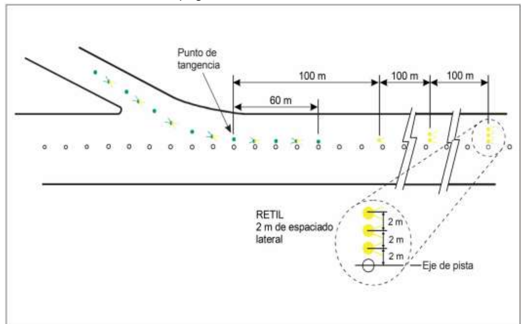
Figura 1-20-1. Luces indicadoras de calle de salida rápida (RETIL)
