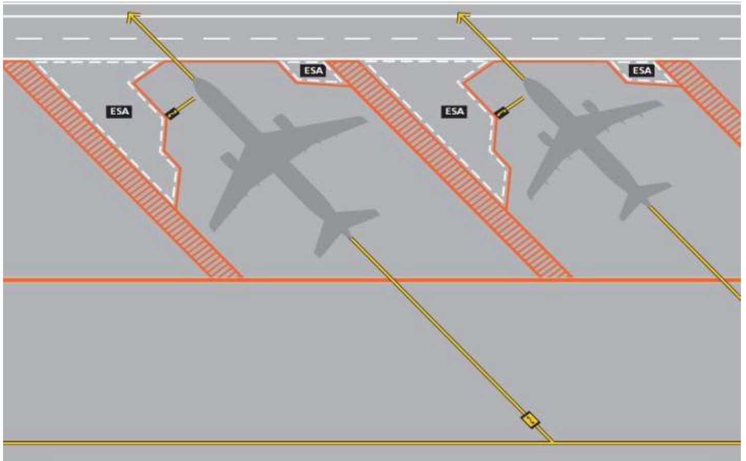
Figura 2-26-4. Ejemplo de Solución de solape para diferentes tipos de aeronave
