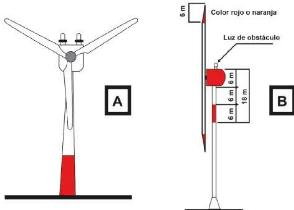
Figura 3-1. Señalización de turbinas eólicas
