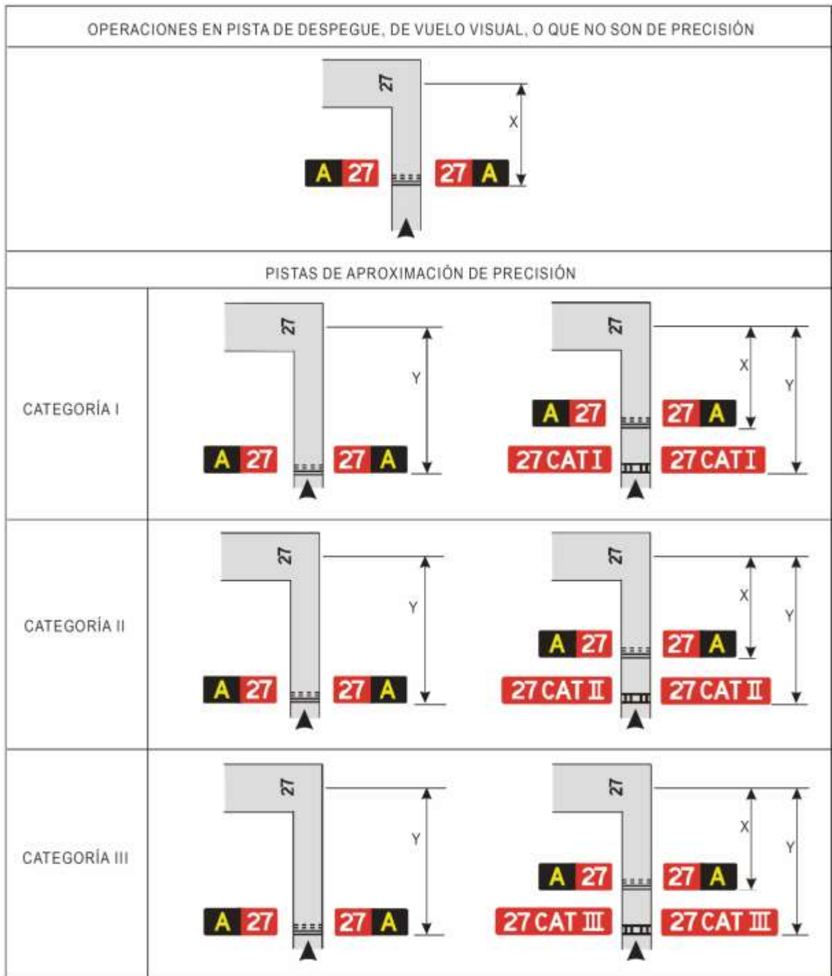
Figura 2-2-3. Ejemplos de la ubicación de los letreros en las intersecciones de calle de rodaje/pista
