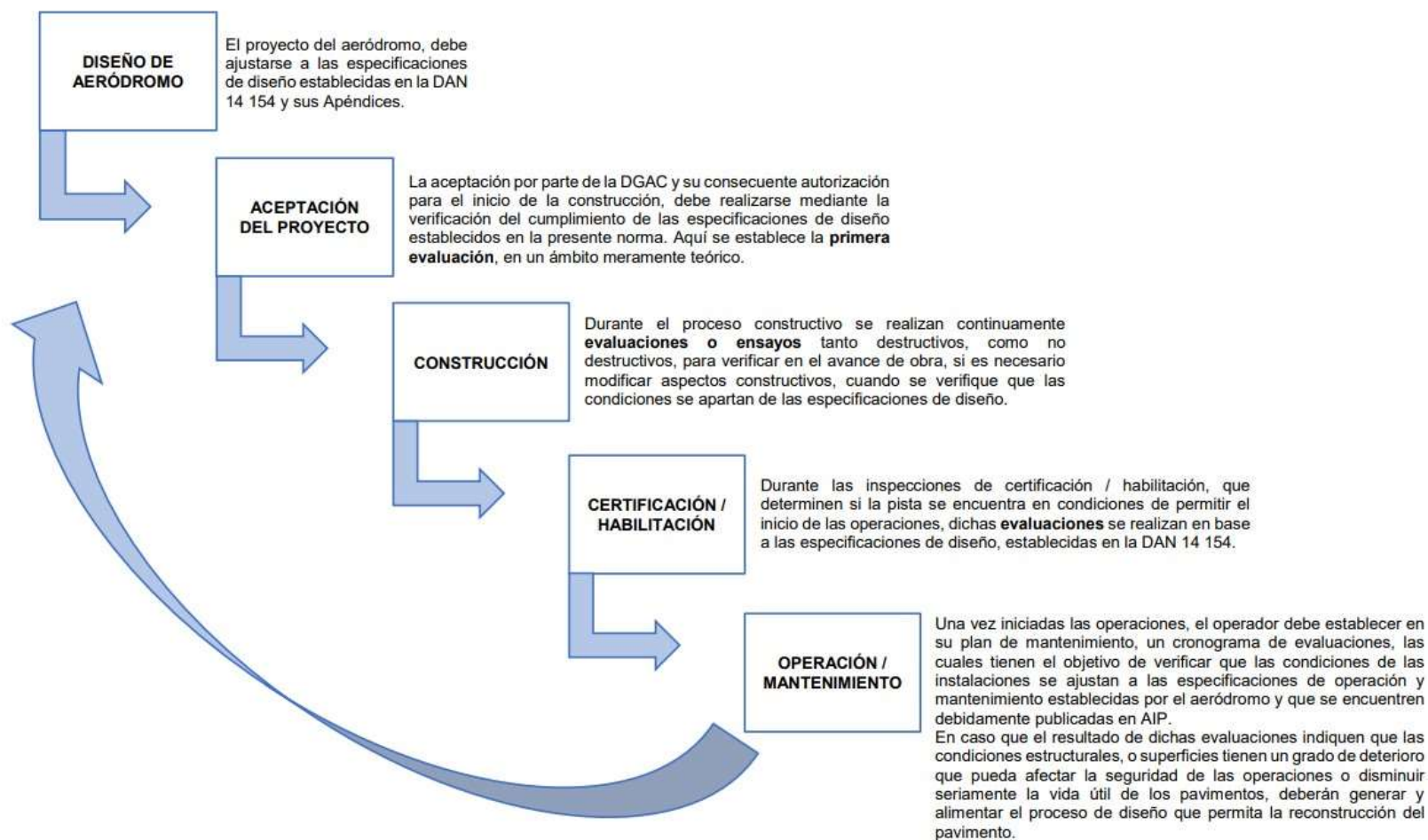
Figura 1-1. Diagrama de vida de un pavimento
