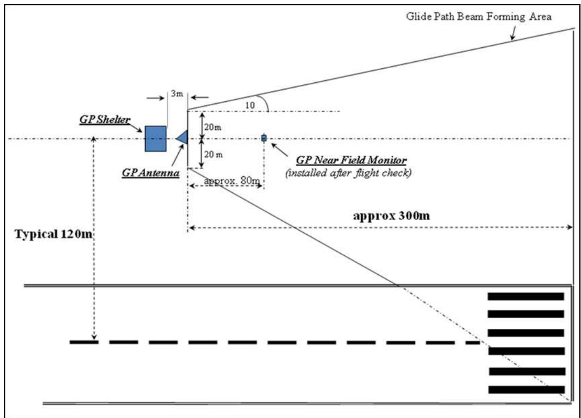
Figura 3-7-2. Área del Guide Slope (ILS)
