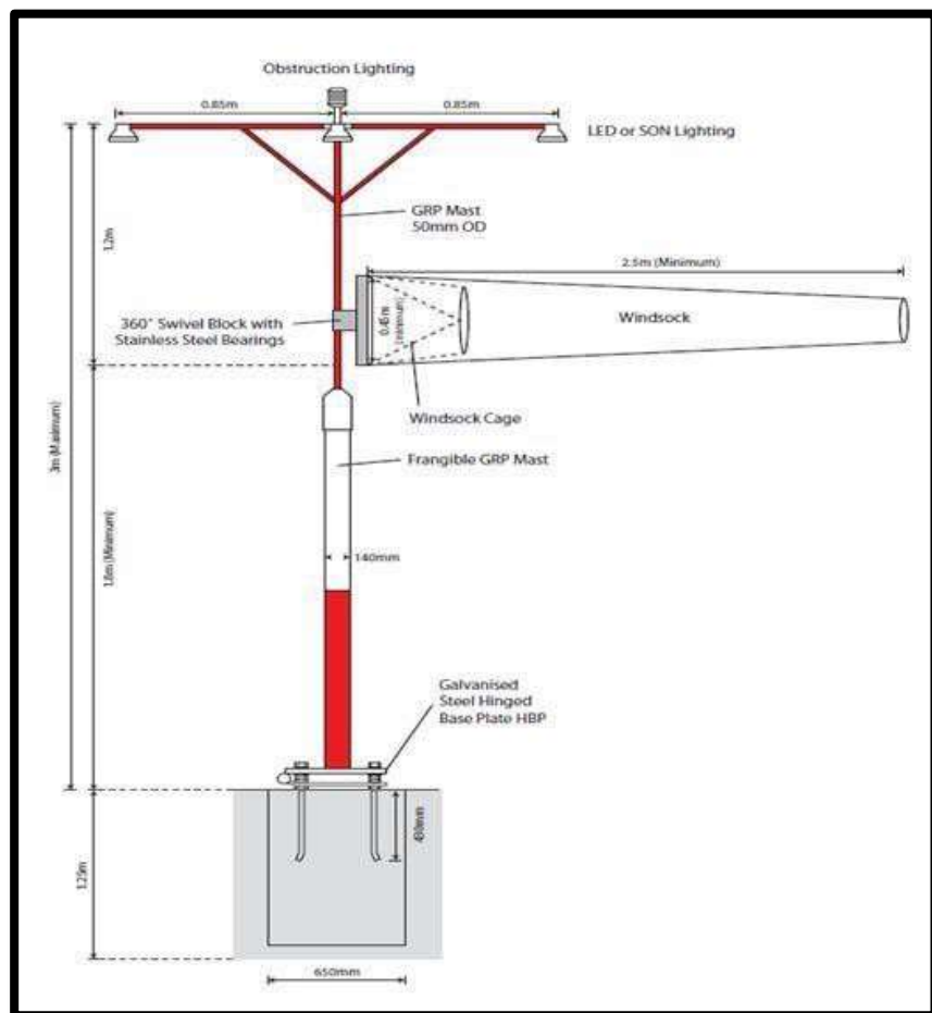
Figura ADJB-2. Mástiles para manga veletas
