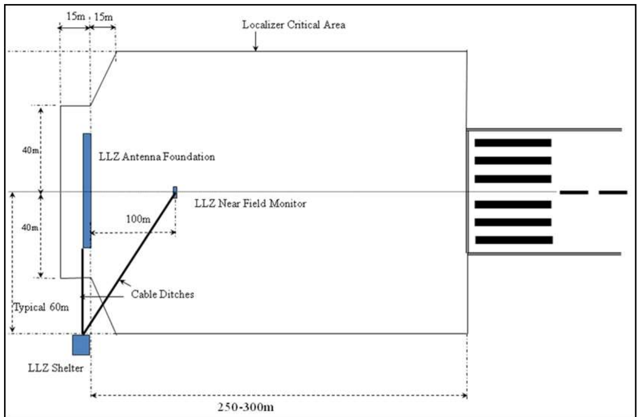
Figura 3-7-1. Área del localizador (ILS)
