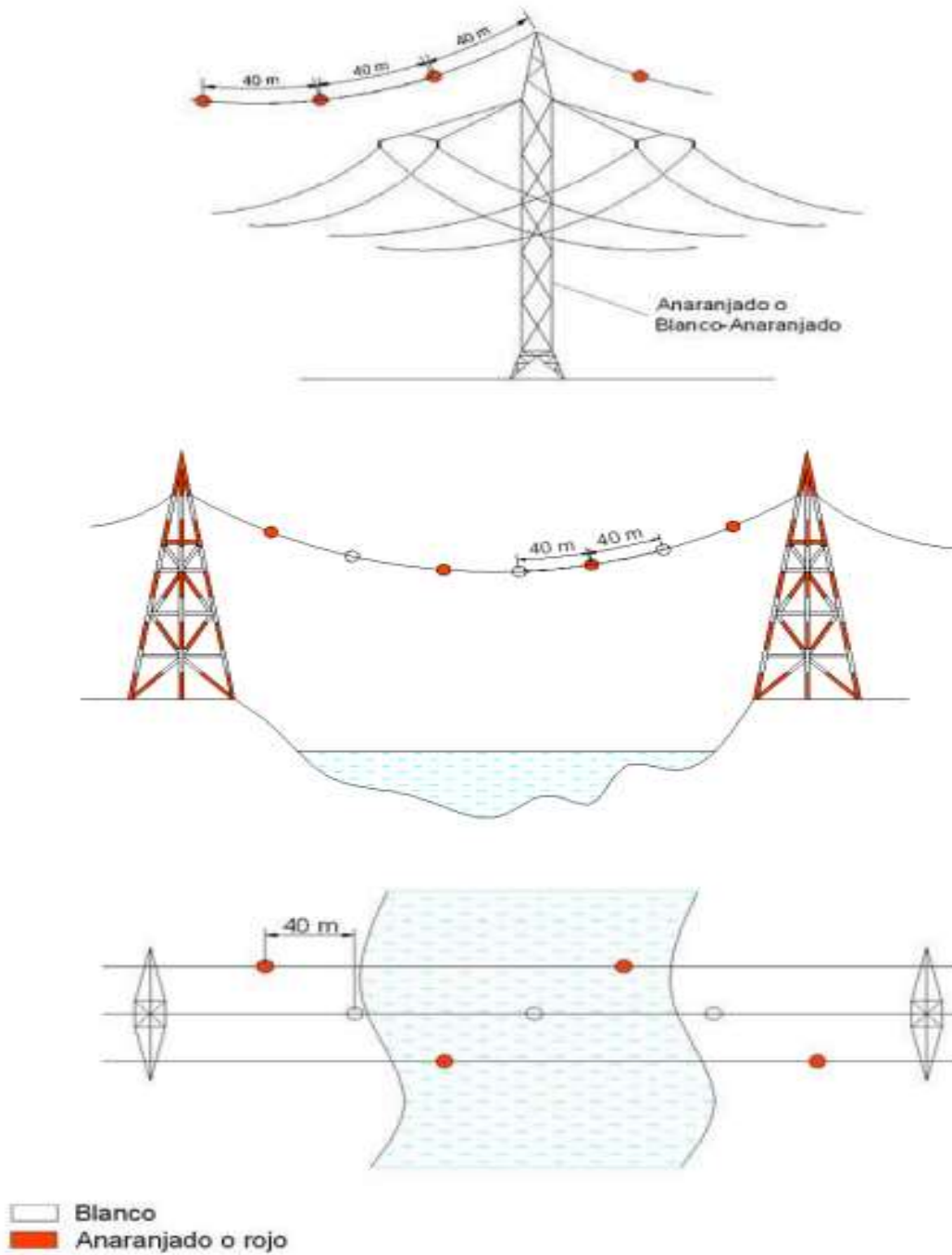
Figura 4-1. Señalamiento de líneas eléctricas
