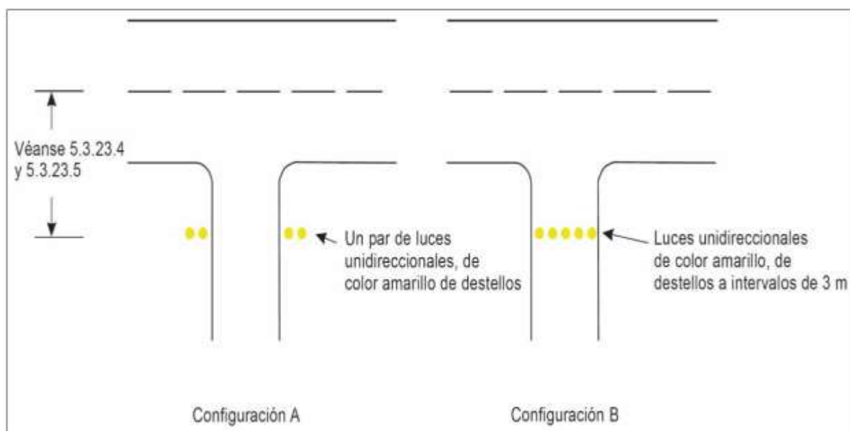
Figura 1-31-1. Luces de protección de pista
