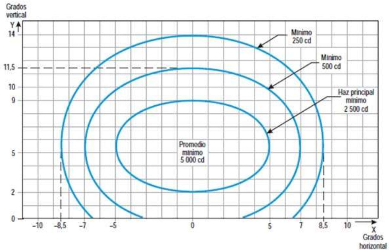
Figura ADJB-5. Diagrama de isocandelas para las luces de toma de contacto (luz blanca)
