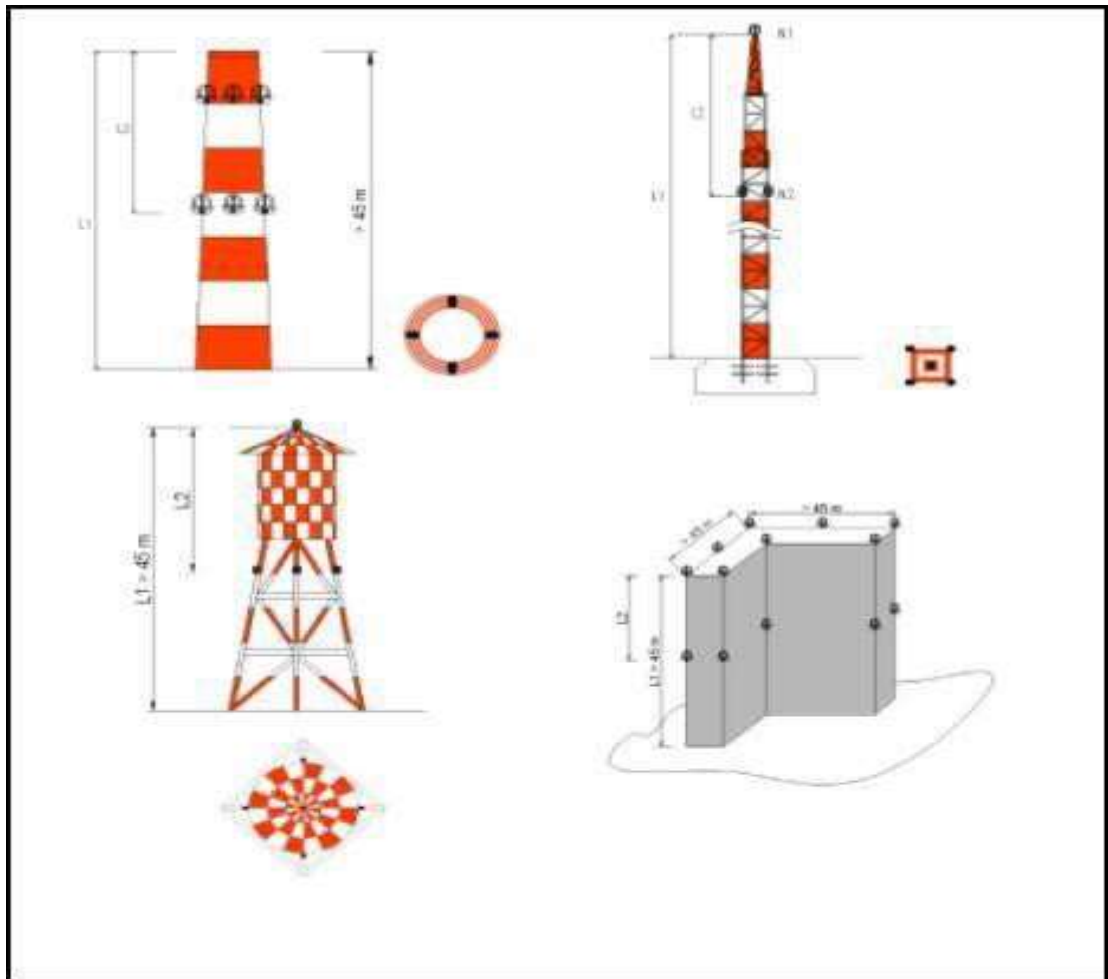
Figura 2-3-5. Ejemplos de iluminación de obstáculos/estructuras >45 m
