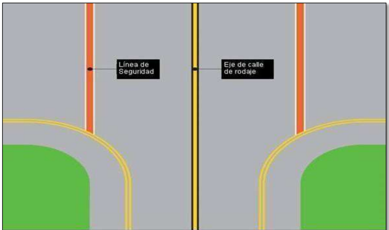
Figura 2-5-2. Línea de seguridad en plataforma ABL y contraste del color
