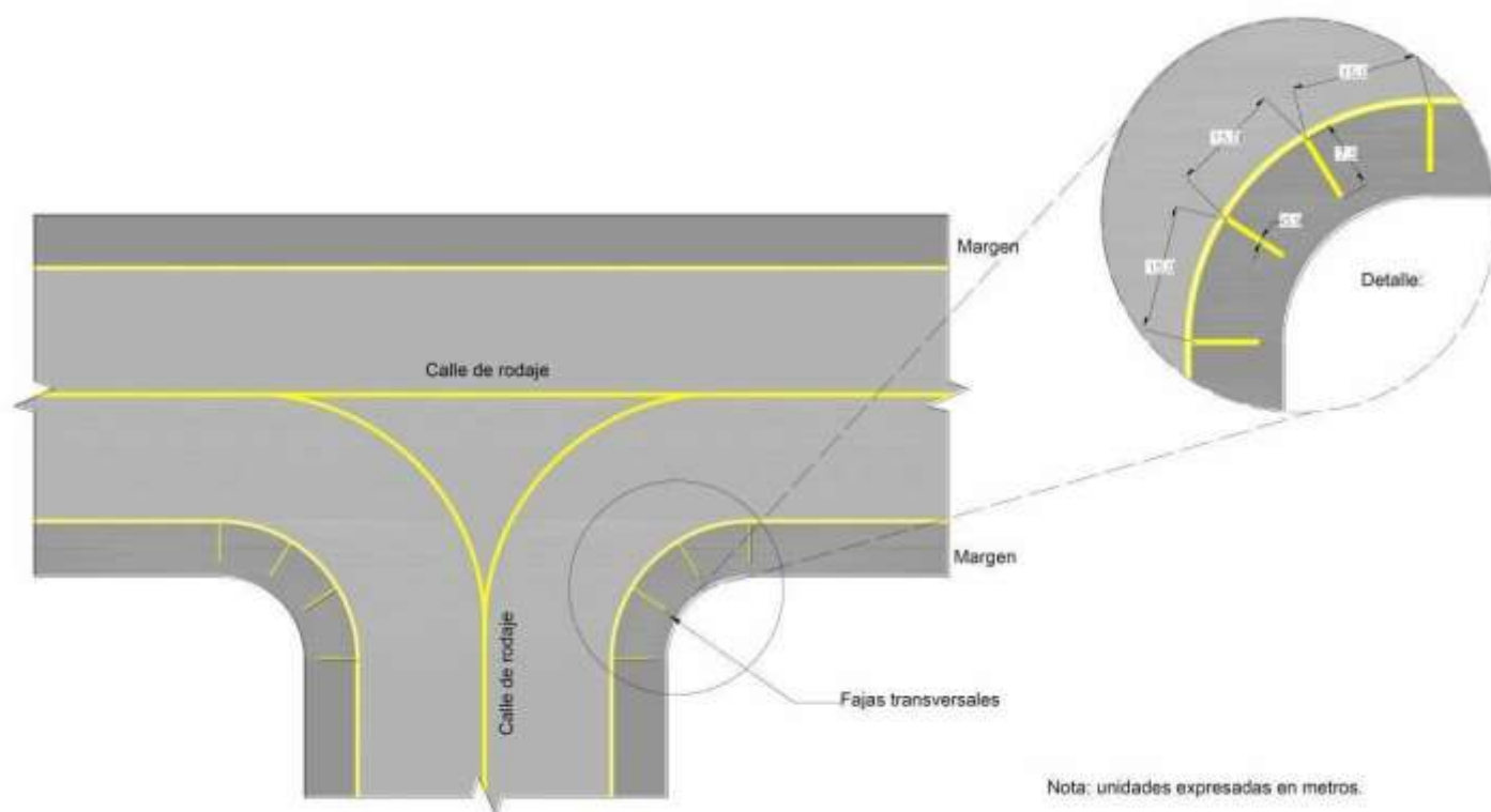
Figura 5-2-1. Señal de faja transversal de calle de rodaje
