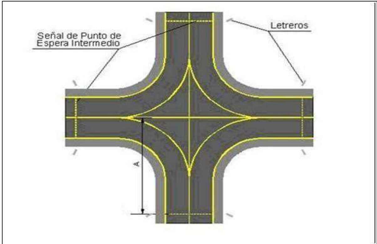
Figura 3-6-1 Señal de punto de espera intermedio.
