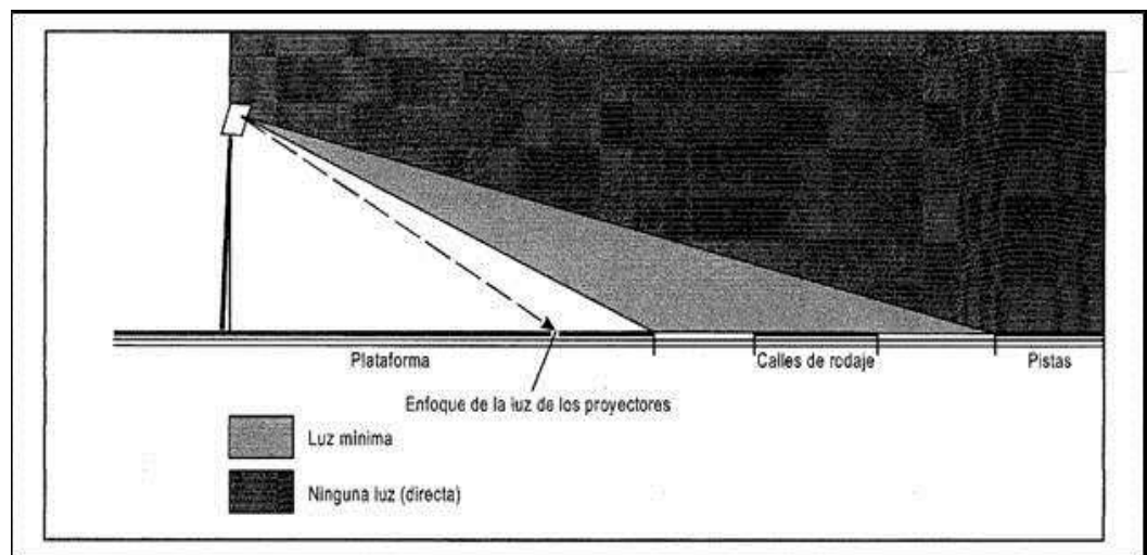
Figura ADJM-1. Enfoque de las luces para evitar el deslumbramiento
