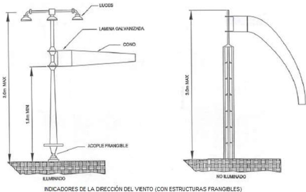
Figura 7-2. Estructuras frangibles
