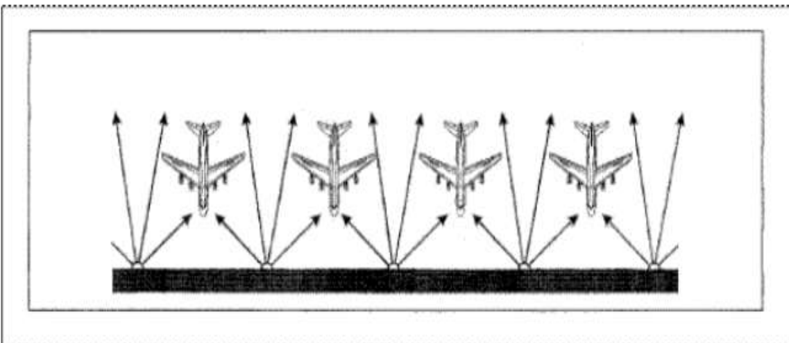
Figura ADJM-7. Disposición y enfoque característicos de las luces de proyectores para estacionamiento con la proa hacia adentro
