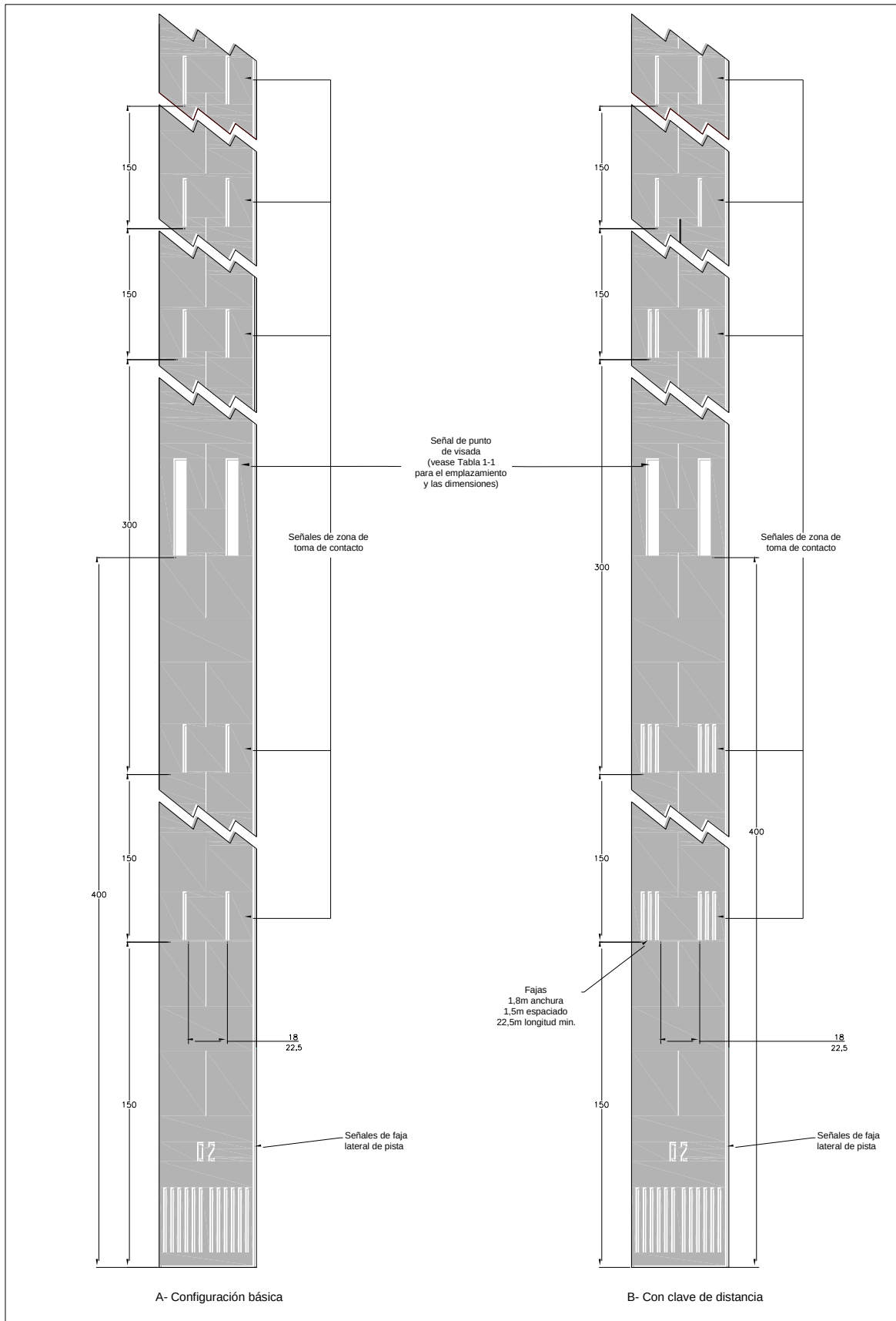
Figura 1-5-1. Señales de punto de visada y de zona de toma de contacto (ilustradas para una pista de 2.400 metros de longitud o más)
