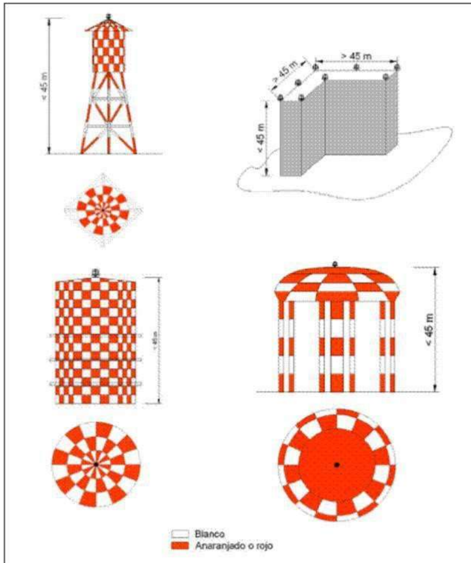
Figura 2-3-4. Ejemplos de iluminación de obstáculos/estructuras <45 m
