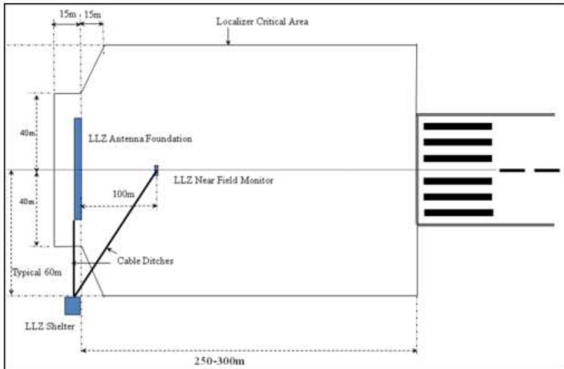
Figura 4-2-1. Instalación del Localizador del ILS
