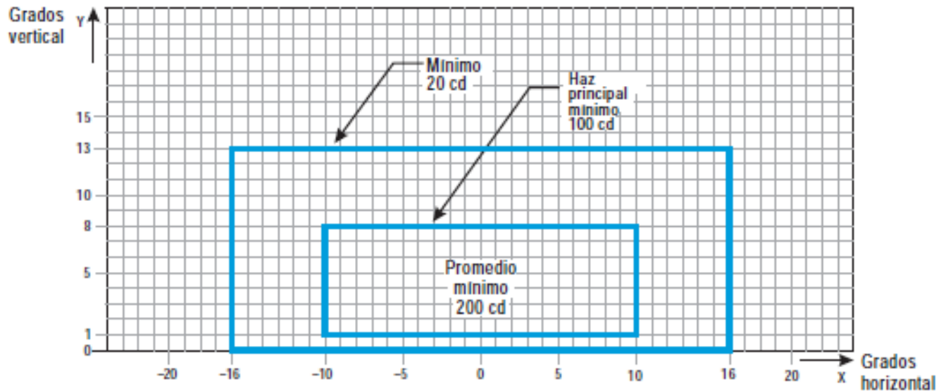
Figura ADJB-12. Diagrama de isocandelas para luces de eje de calle de rodaje (espaciado de 15 metros), de barra de prohibición de acceso y de barra de parada en tramos rectos previstas para ser utilizadas en condiciones de alcance visual en la pista inferior a un valor de 350 metros cuando pueda haber grandes desplazamientos y para luces de protección de pista de baja intensidad, configuración B
