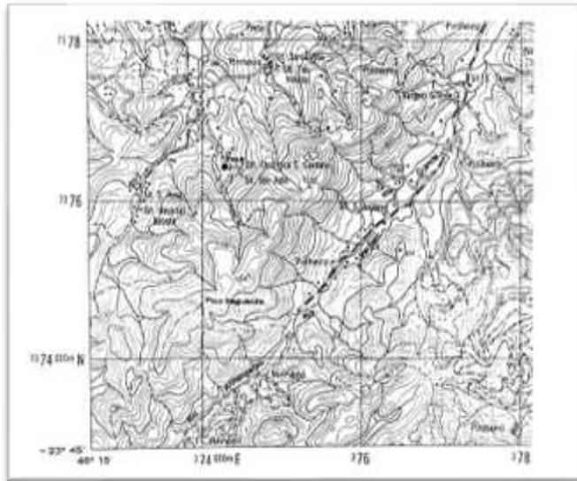
Figura 6-4. Cuadrícula UTM
