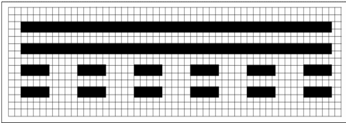
Figura ADJD-3A Ejemplo - Letrero de pista libre
