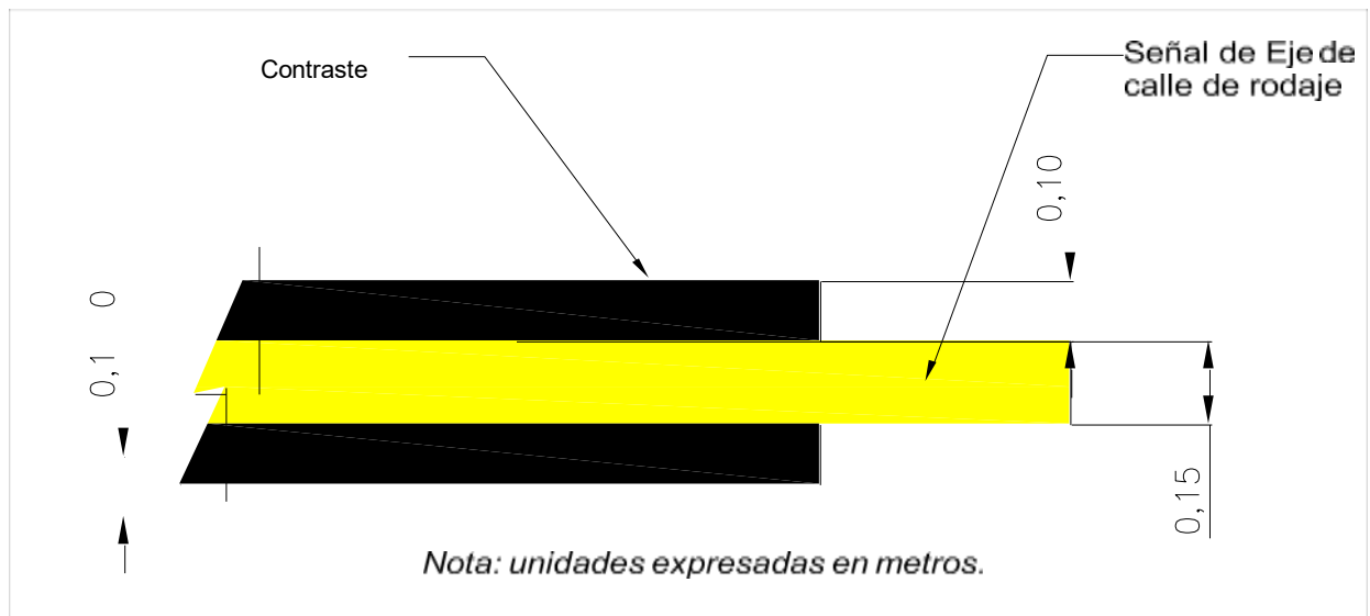
Figura 3-1-3. Señal de eje de calle de rodaje - Detalle
