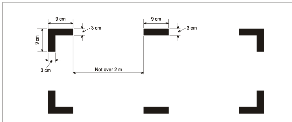
SEÑALAMIENTO DE LAS ZONAS DE PENETRACIÓN DEL FUSELAJE
