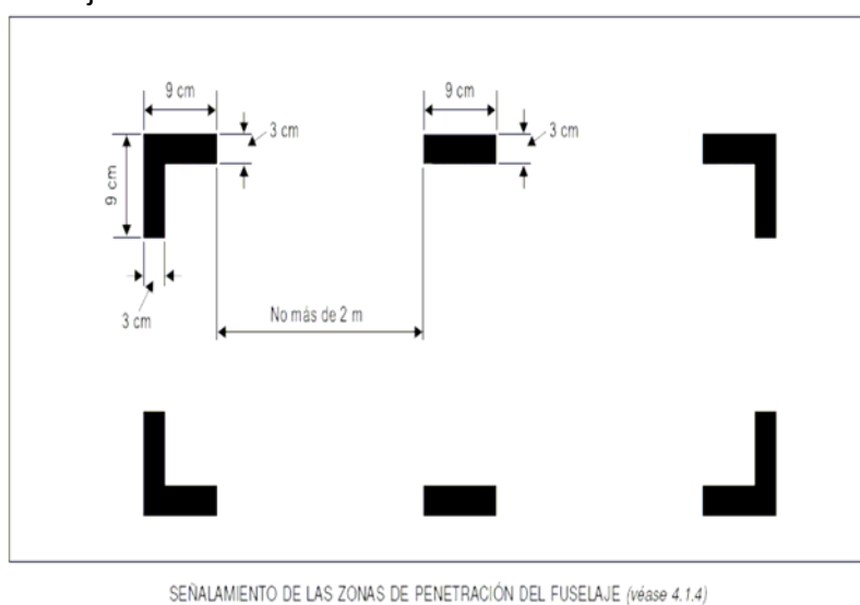
SEÑALAMIENTO DE LAS ZONAS DE PENETRACIÓN DEL FUSELAJE (véase 4.1.4)
