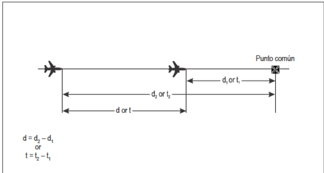
Figura 7-27. Cálculo de la distancia/tiempo longitudinal entre aeronaves — derrota idéntica, mismo sentido [véase 7.4.3.11.5 a)]
