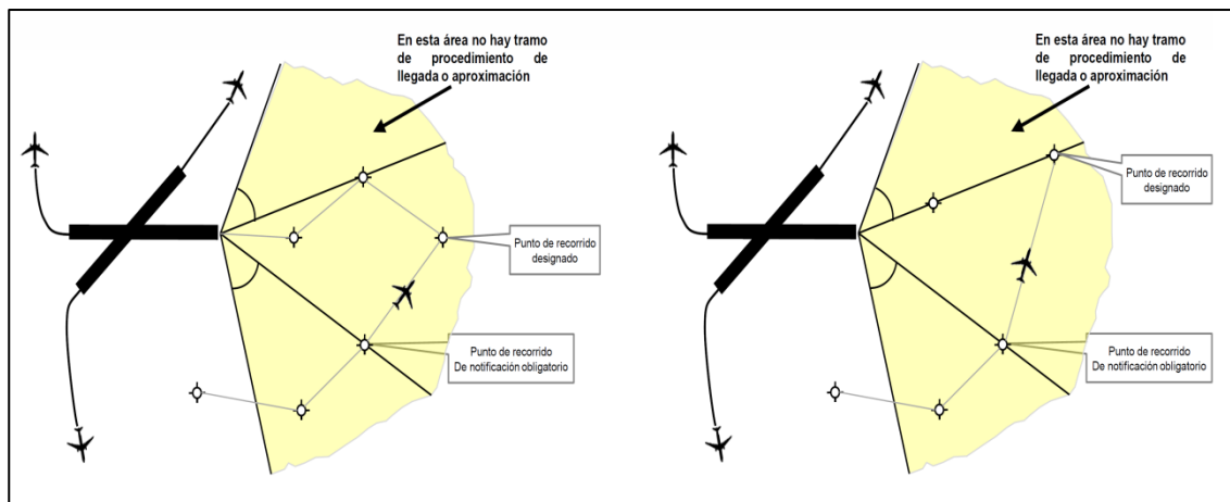
Figura 7-37a Área de protección de llegada
