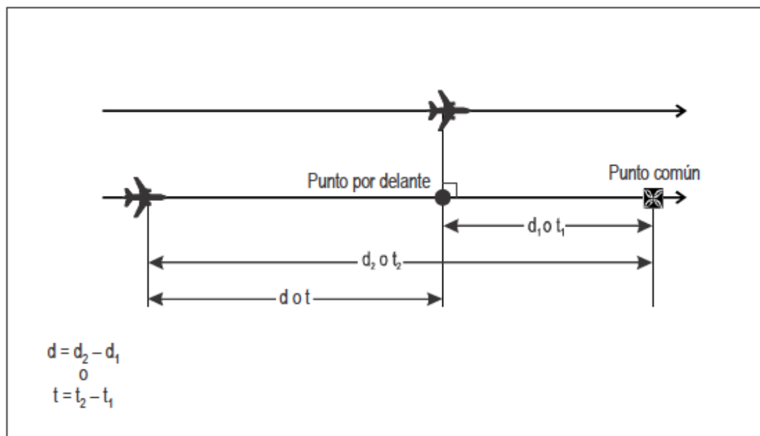
Figura 7-32. Cálculo de la distancia/tiempo longitudinal entre aeronaves — derrota paralelas [véase 7.4.3.11.5 c)]
