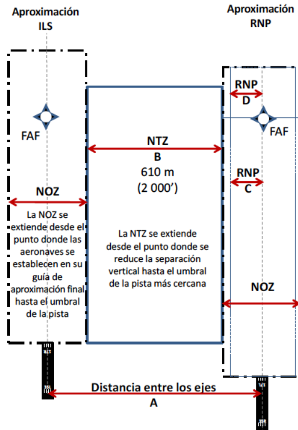
Figura 6-1 Distancia entre los ejes, NTZ y NOZ
