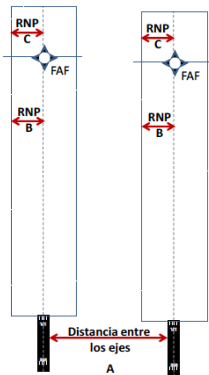
Figura 6-2 Valor RNP y distancia entre los ejes de las pistas
