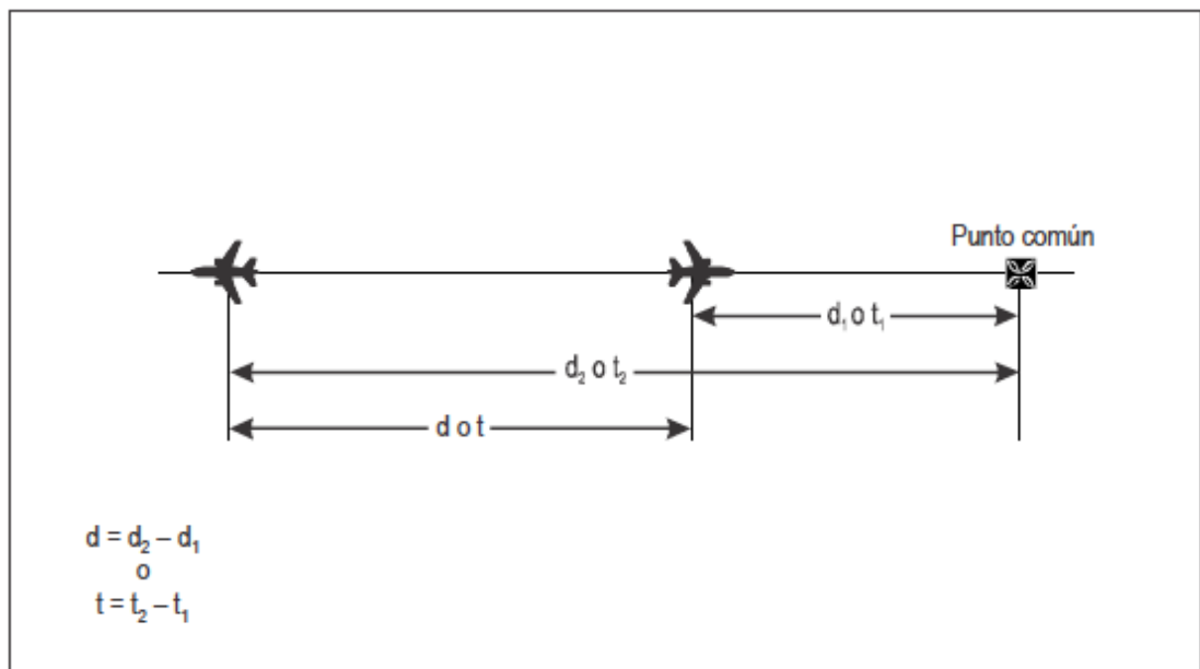
Figura 7-28. Cálculo de la distancia/tiempo longitudinal entre aeronaves — derrota idéntica, sentido opuesto [véase 7.4.3.11.5 a)]
