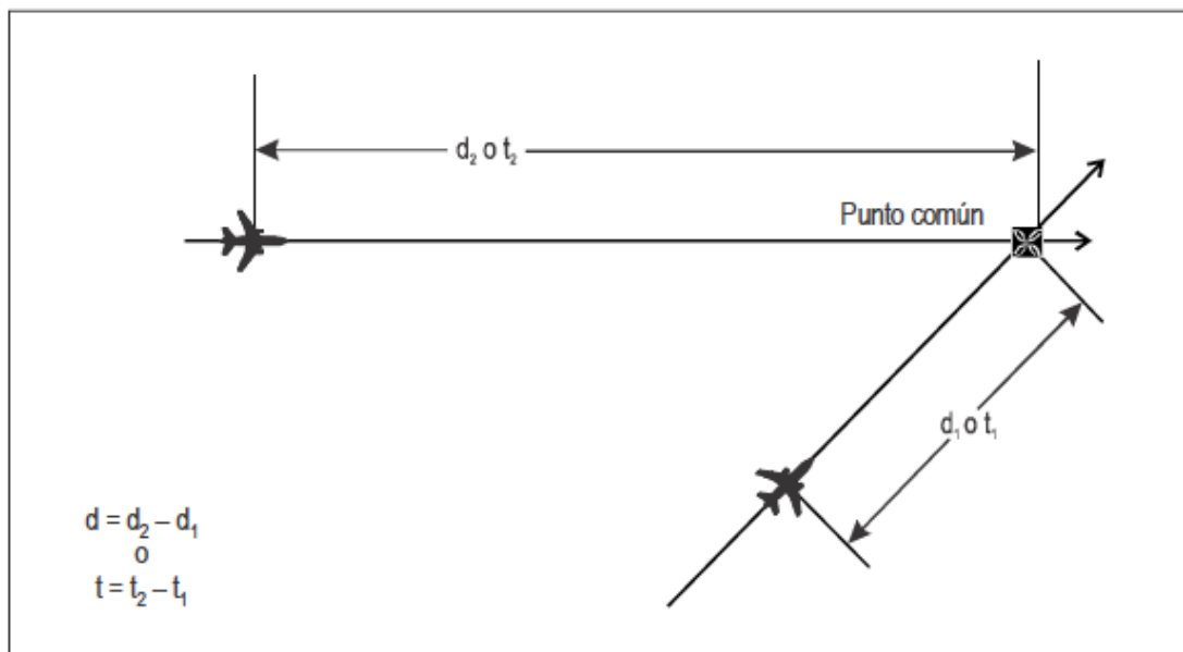
Figura 7-29. Cálculo de la distancia/tiempo longitudinal entre aeronaves — misma derrota, pero no idéntica y derrotas que se cruzan [véase 7.4.3.11.5 b)]
