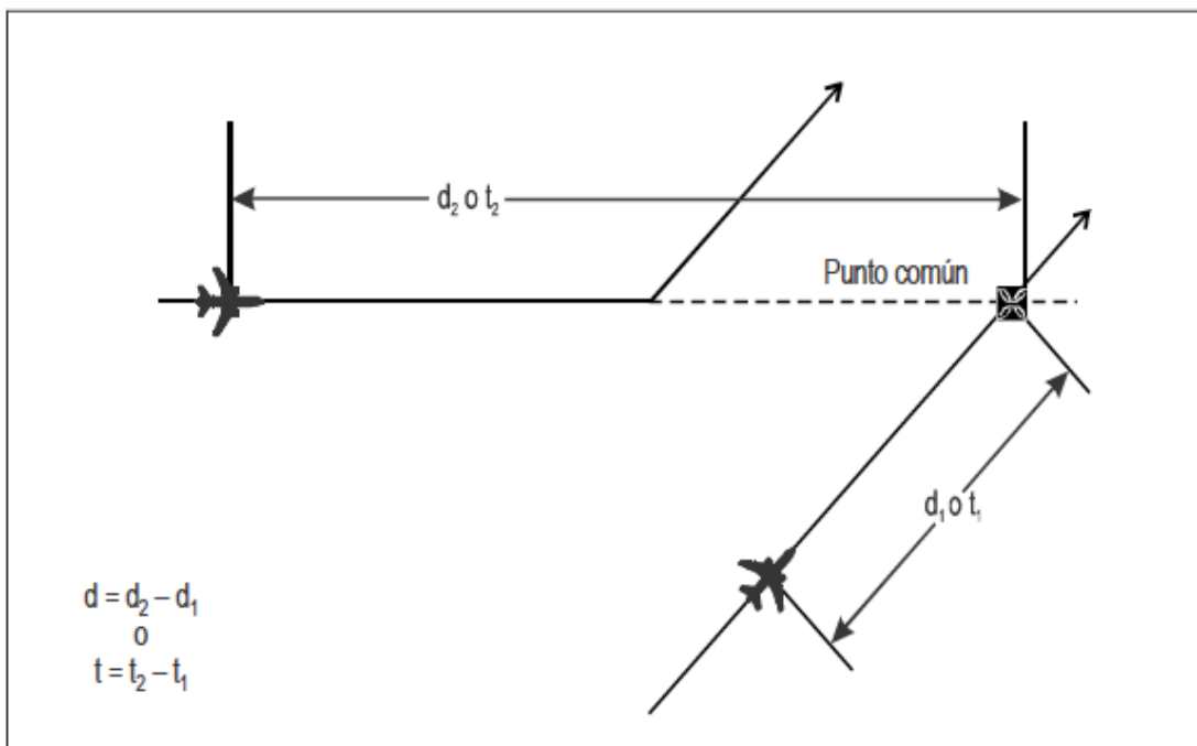
Figura 7-30. Cálculo de la distancia/tiempo longitudinal entre aeronaves — misma derrota prevista, pero no idéntica [véase 7.4.3.11.5 b)]
