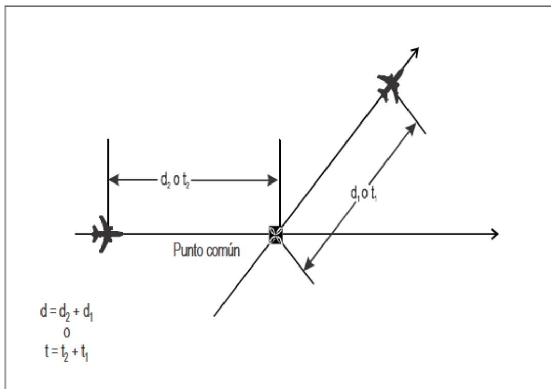
Figura 7-31. Cálculo de la distancia/tiempo longitudinal entre aeronaves — lados opuestos del punto común [véase 7.4.3.11.5 b)]
