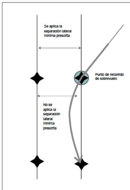
Viraje sobre un punto de recorrido de sobrevuelo
