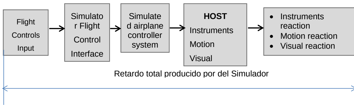
Figura A2E.- Retardo para una simulación de una aeronave controlada por computadoras y que usa equipamiento simulado de la aeronave emulada.
