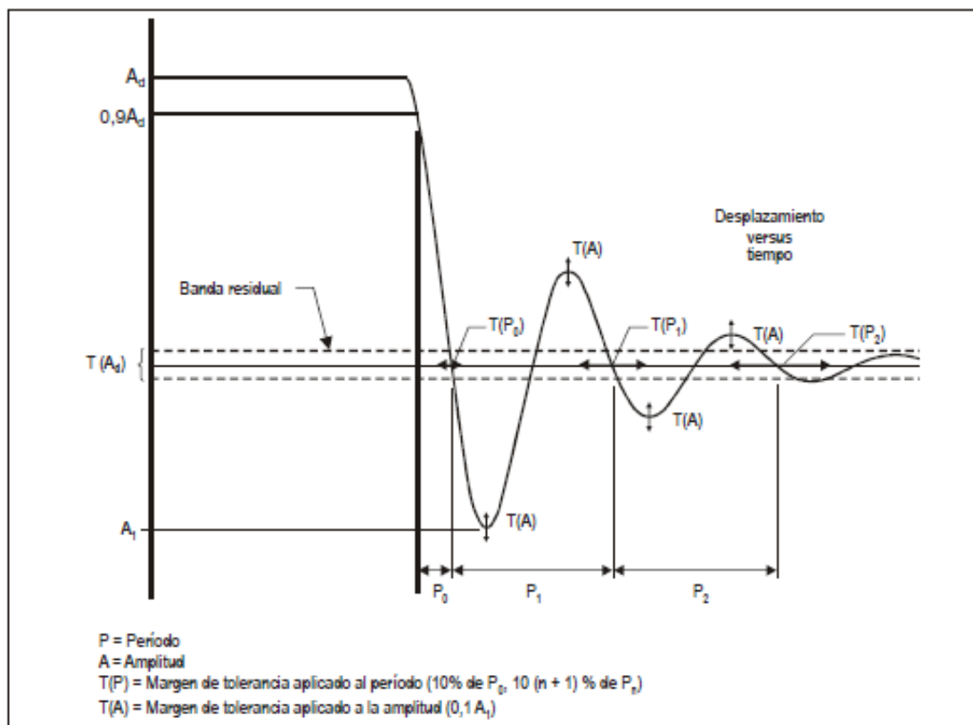
Figura C2A. Respuesta escalonada Sub-Amortiguada
