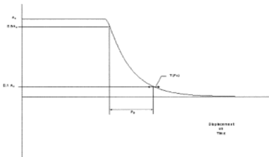
Figura C2B. Respuesta escalonada Críticamente Amortiguada
