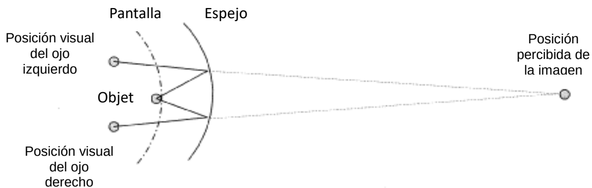
FIGURA C2I – DISPLAY COLIMADO
