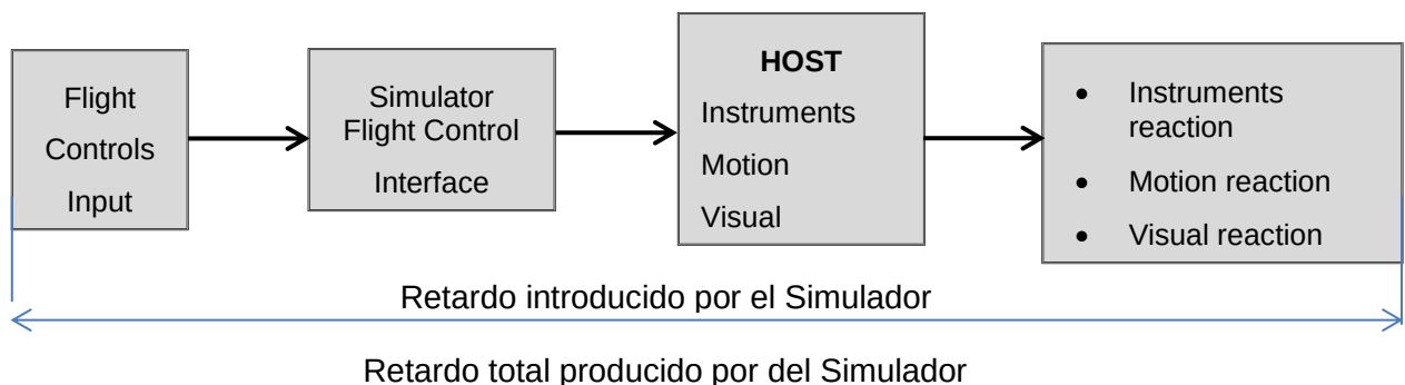
Figura A2C.- Retardo para la simulación de una aeronave no controlada por computadoras.
