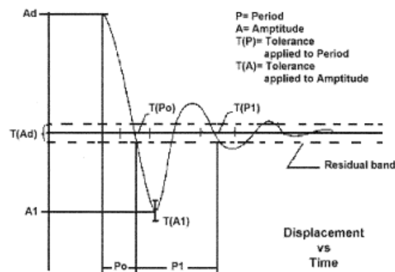
Figura D2A Respuesta Subamortiguada
