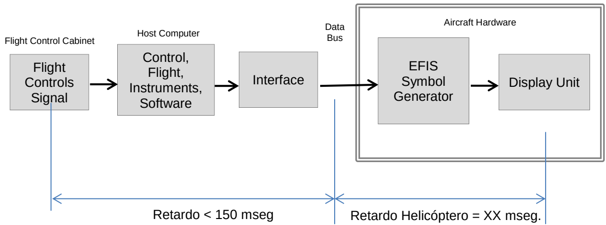
Figura C2HA.- Retardo para la simulación de helicópteros que usan instrumentos reales del helicóptero.
