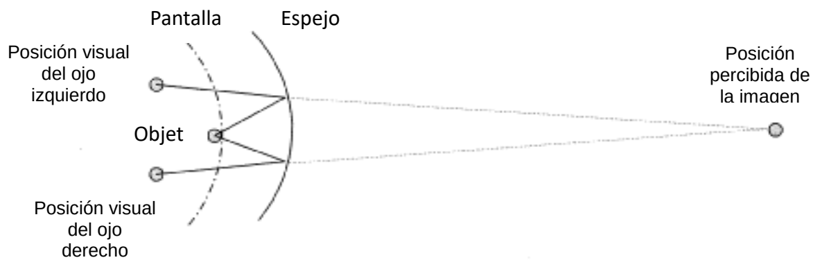
FIGURA C2I – DISPLAY COLIMADO
