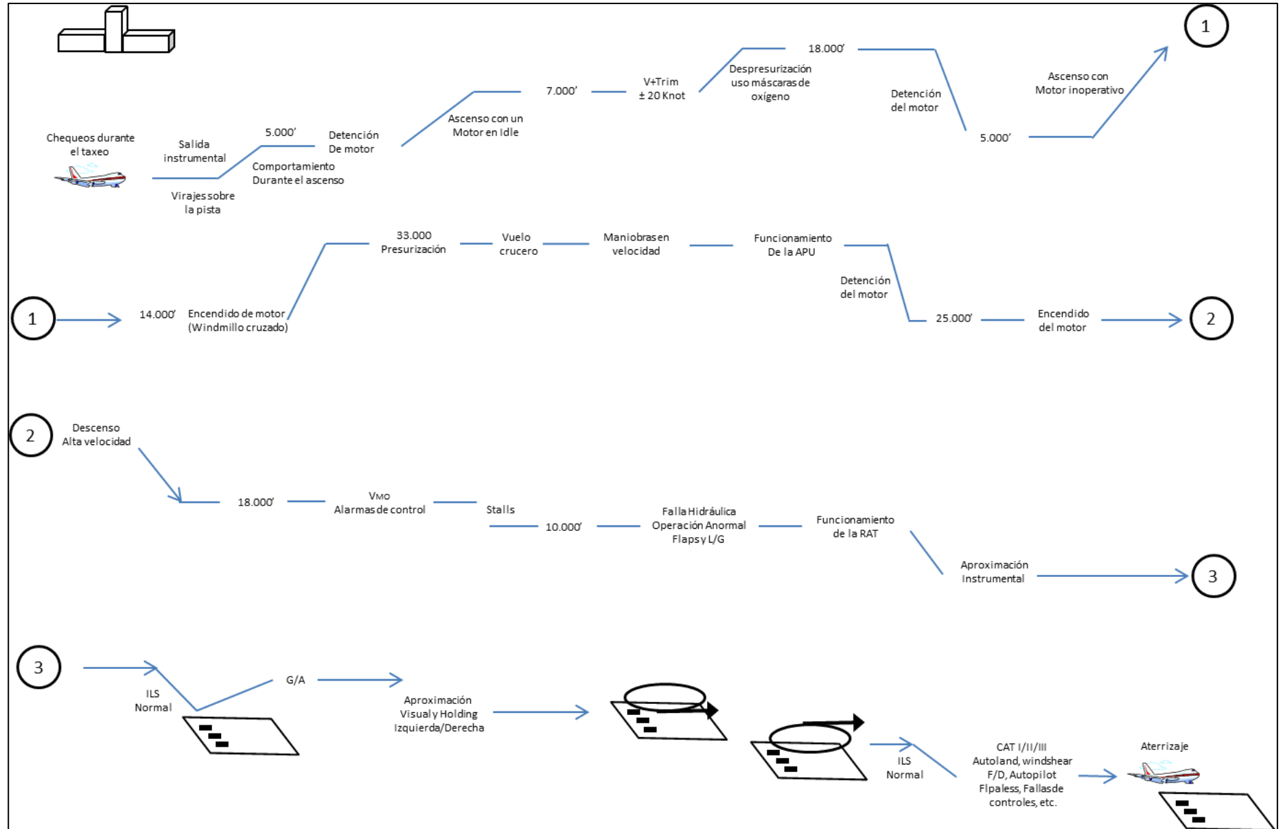
FIGURA A4J: PERFIL TÍPICO PARA LA EVALUACIÓN SUBJETIVA DE UN SVA
