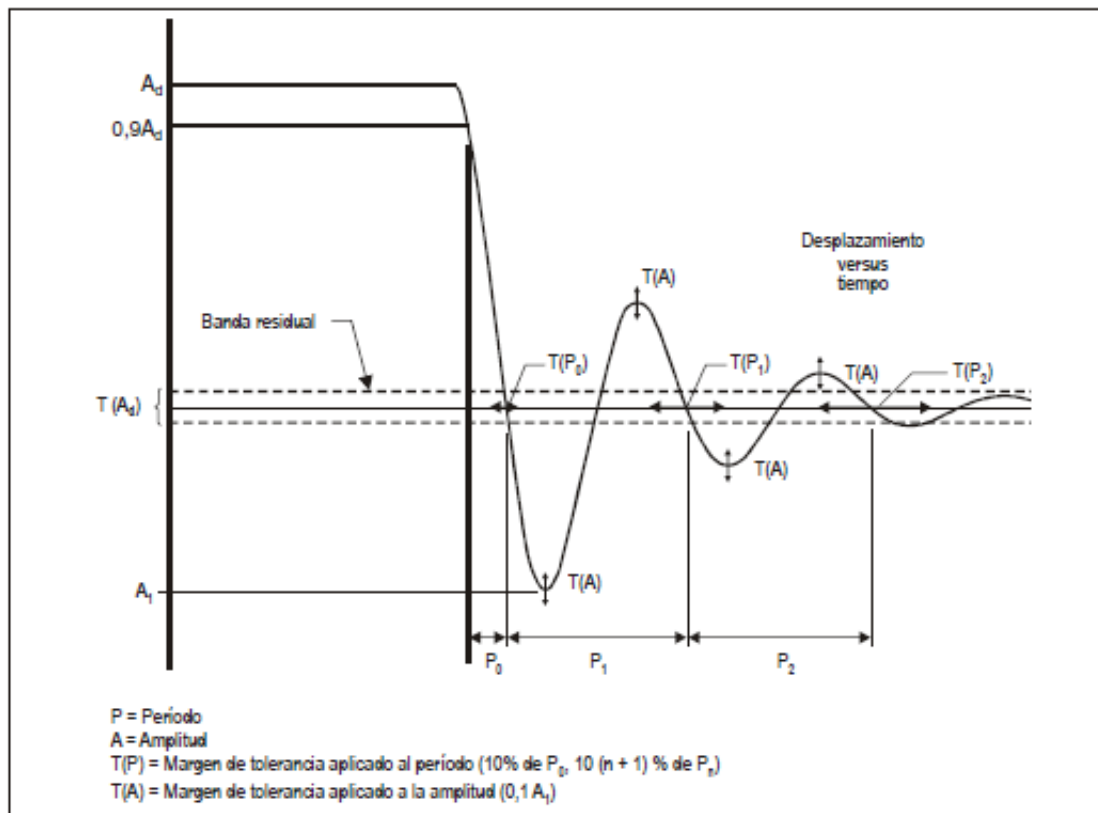
Figura C2A. Respuesta escalonada Sub-Amortiguada
