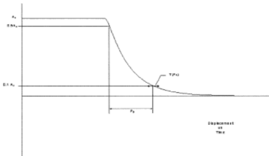
Figura C2B. Respuesta escalonada Críticamente Amortiguada
