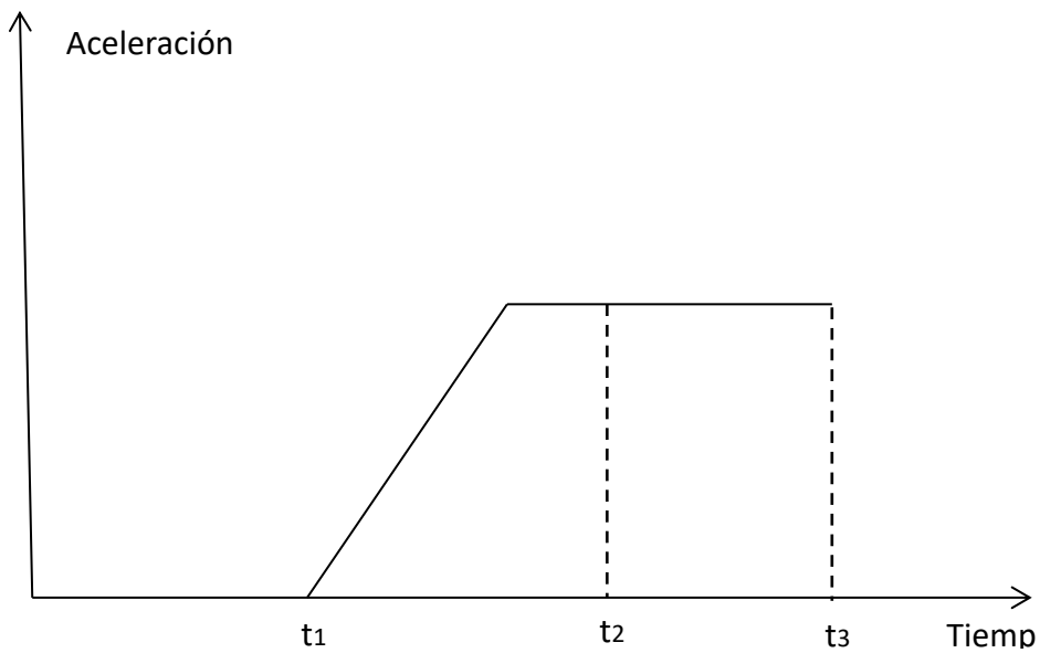
Figura C2D. Características de las señales de prueba
