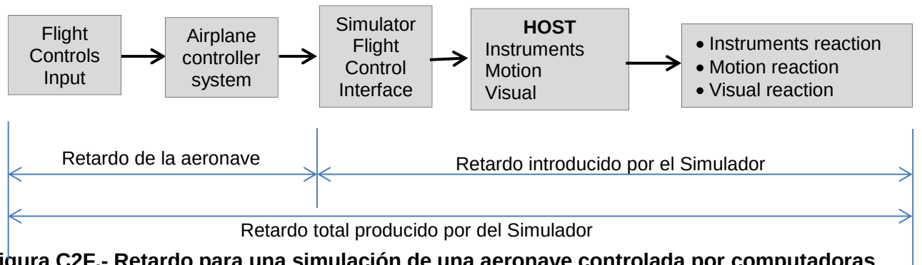
Figura C2F.- Retardo para una simulación de una aeronave controlada por computadoras y que usa equipamiento real del helicóptero emulado (Black Boxes)
