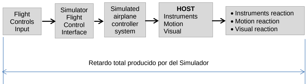
Figura C2G.- Retardo para una simulación de una aeronave controlada por computadoras y que usa software simulado de las cajas negras del helicóptero.
