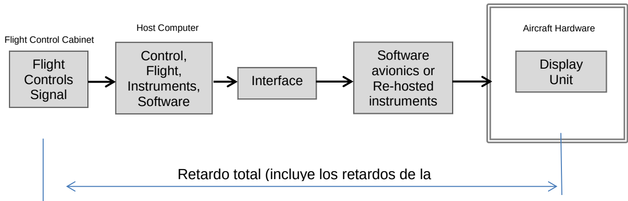
Figura A2FB. - Retardo para la simulación de una aeronave que usa aviónica simulada por software o instrumentos integrados en la aeronave emulada.
