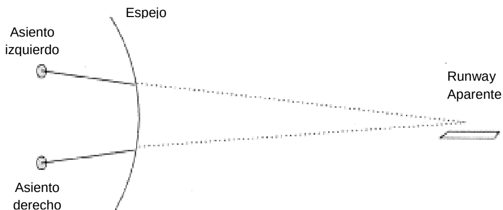
FIGURA C2J –VISUAL DE UNA RUNWAY EN UN DISPLAY COLIMADO
