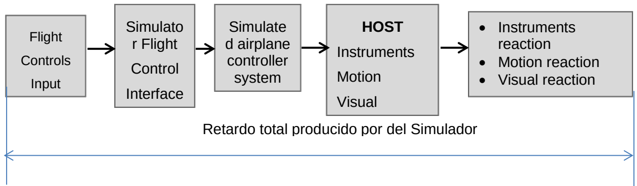
Figura A2E.- Retardo para una simulación de una aeronave controlada por computadoras y que usa equipamiento simulado de la aeronave emulada.
